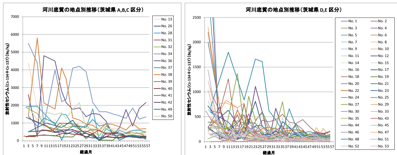
図 4.3-7 各地点の経年的な推移（茨城県：河川底質）
