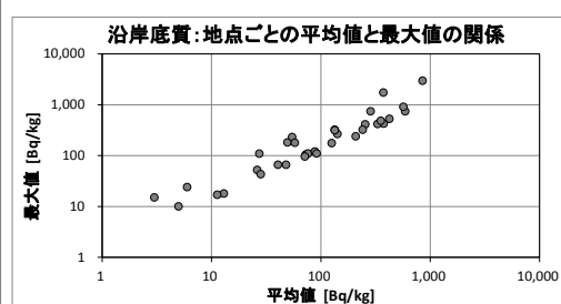
図 4.3-1 地点平均値の順位による区分の設定状況 (左: 設定のイメージ、右上: 区分整理結果 11 、右下: 地点平均値と最大値の関係)
