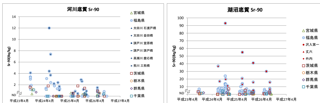
図 3.2-1 公共用水域の底質中の Sr-90 の検出状況（左：河川、右：湖沼）
