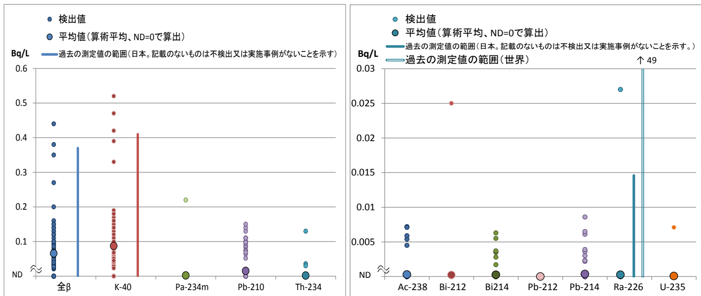
図 3.1-3 地下水の全 \beta 及び \gamma 線核種の検出状況
