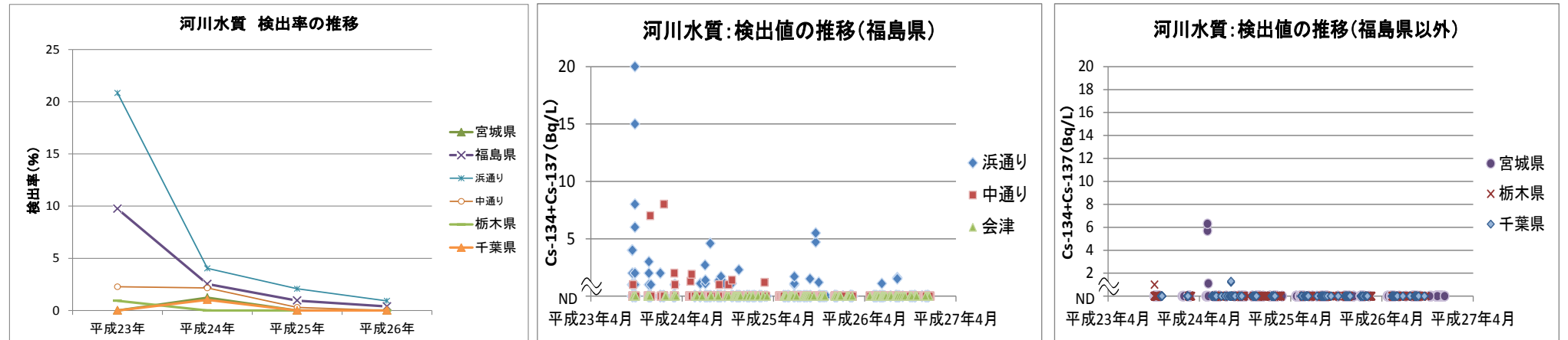
図 4.1-1 水質：公共用水域（河川）の放射性セシウムの検出率（左）及び検出値の推移（中及び右）
