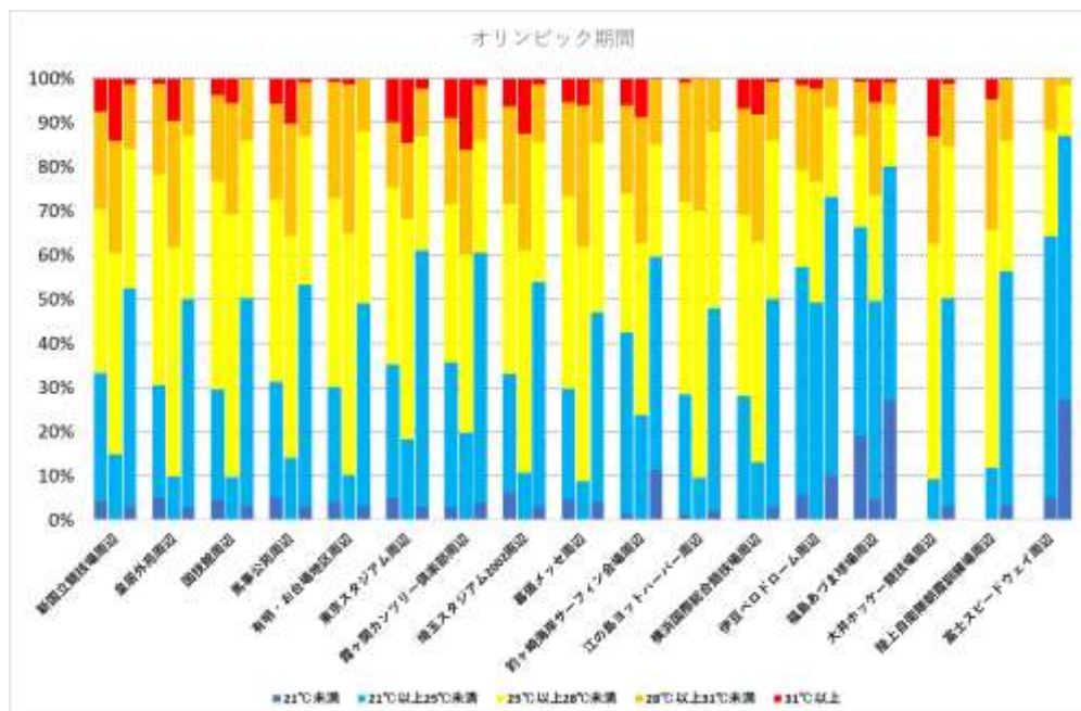
図 5-11(c) 運動指針で分けたオリンピック期間の標準型 WBGT 測定値の各年ごとの分布
