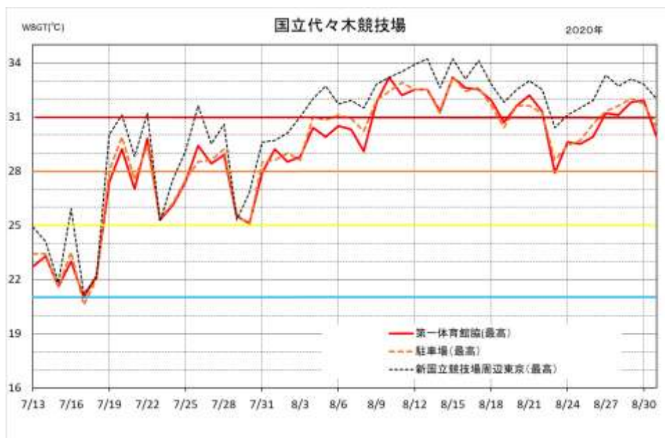
図 5-17 (b) 国立代々木競技場及び比較地点での日最高 WBGT の変化
