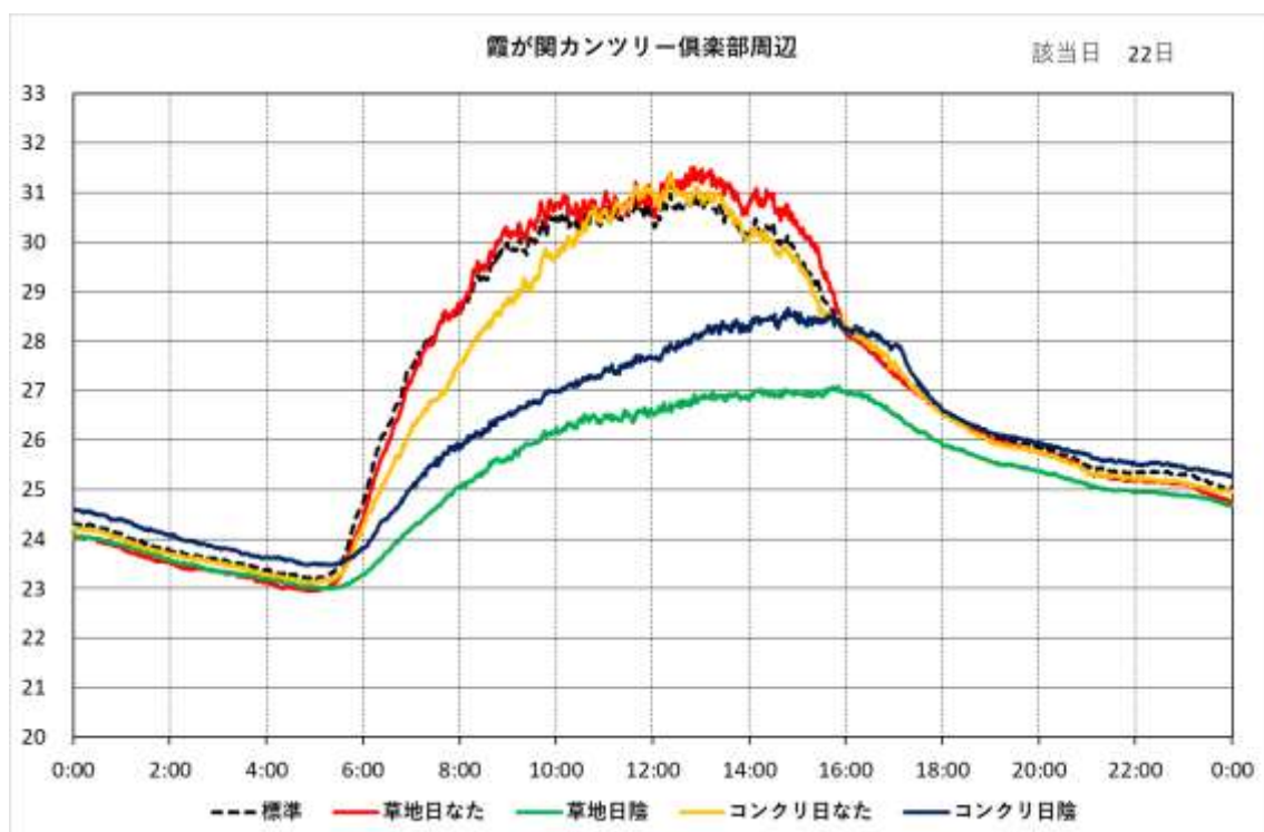
図 5-16 (g) 時刻別 WBGT の日変化（霞ヶ関カンツリー倶楽部周辺）
