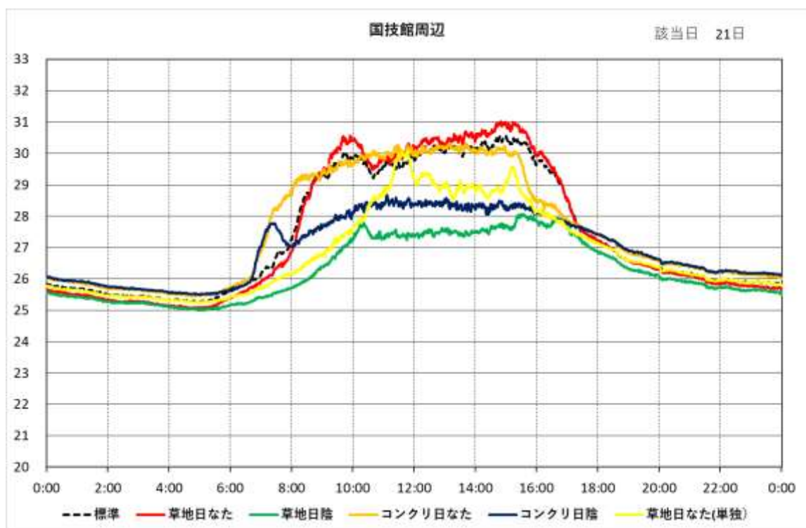
図 5-16 (c) 時刻別 WBGT の日変化 (国技館周辺)
