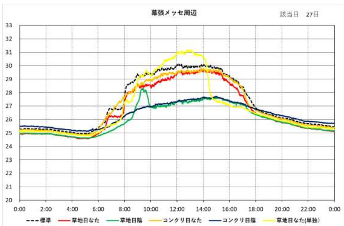
図 5-16(i) 時刻別 WBGT の日変化 (幕張メッセ周辺)
