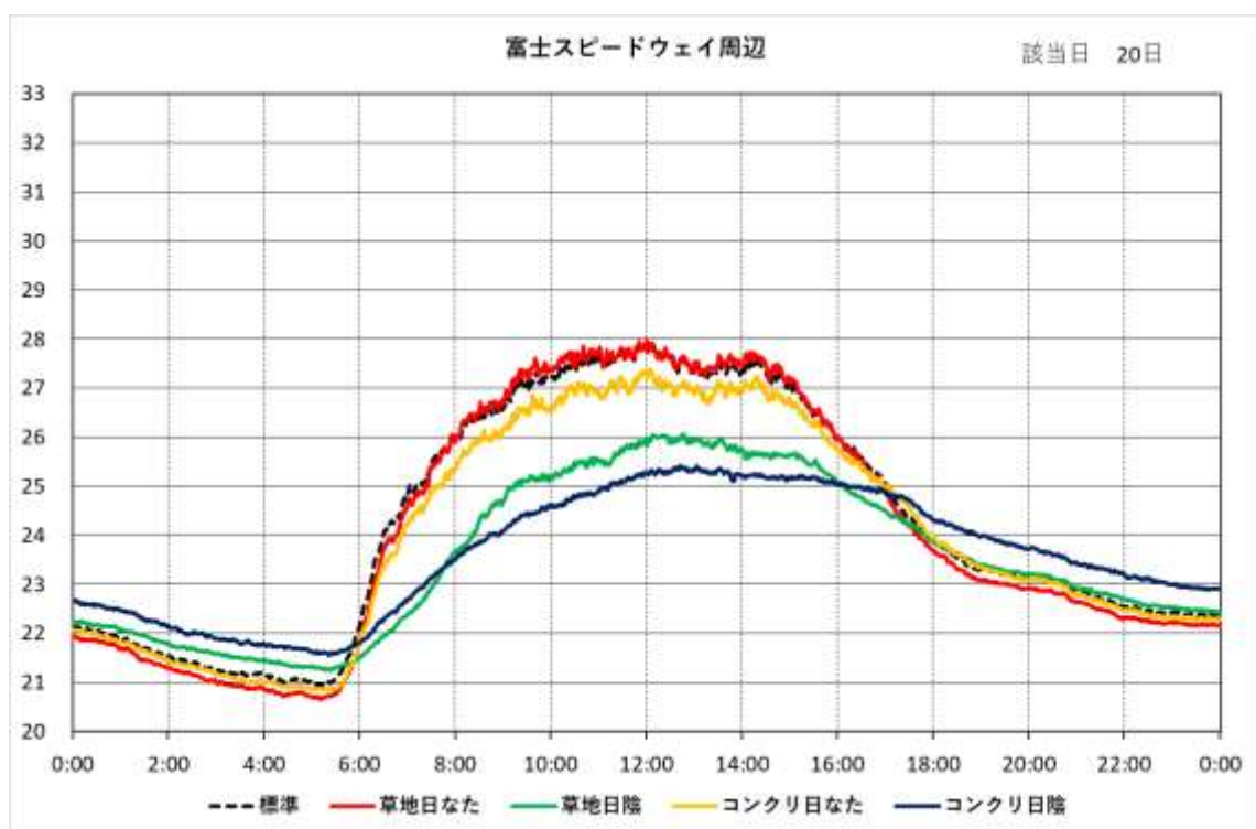
図 5-16 (q) 時刻別 WBGT の日変化 (富士スピードウェイ周辺)
