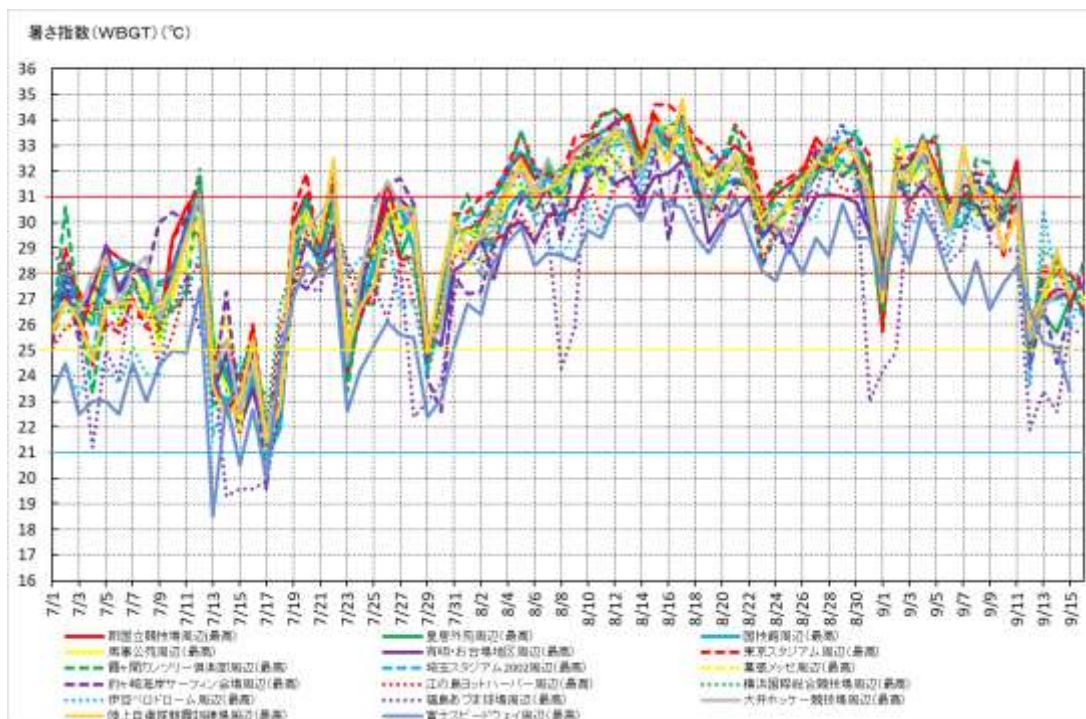
図 5-4 WBGT 日最高値の変化（17 地区、標準点）
