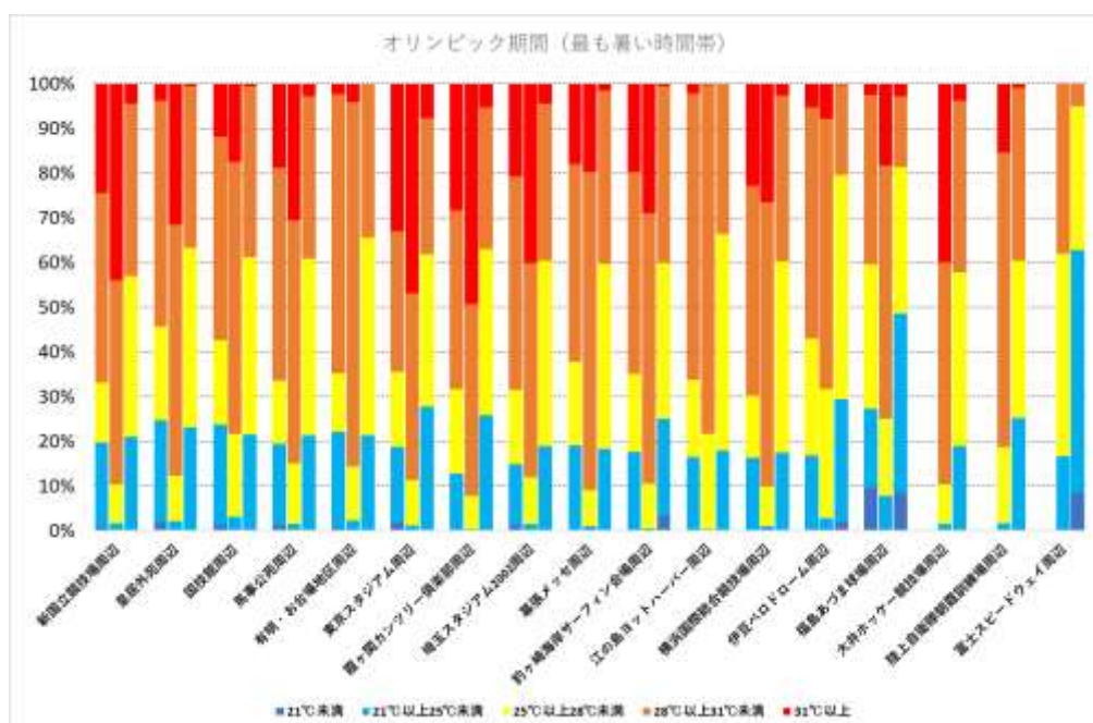
図 5-12(e) 運動指針で分けたオリンピック期間の競技時間帯の標準型 WBGT 測定値の各年ごとの分布
