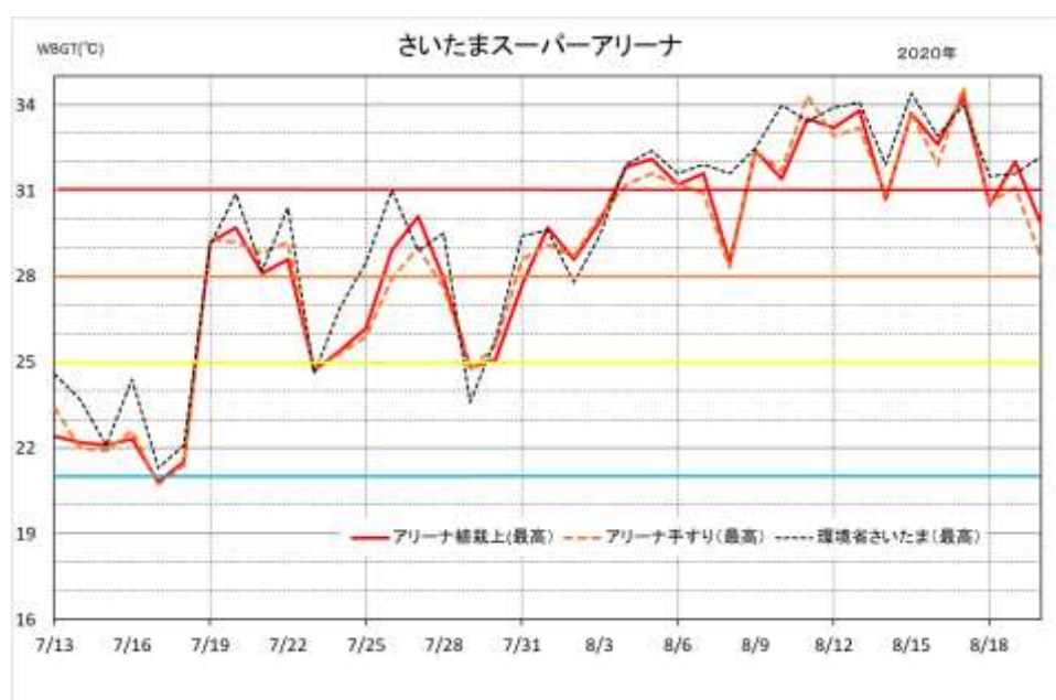
図 5-17(a) さいたまスーパーアリーナ及び比較地点での日最高 WBGT の変化 比較地点と同様の変化を示しているが、比較地点（「さいたま」）が高い場合も多い。
