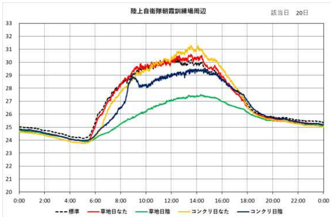
図 5-16 (p) 時刻別 WBGT の日変化 (陸上自衛隊朝霞訓練場周辺)
