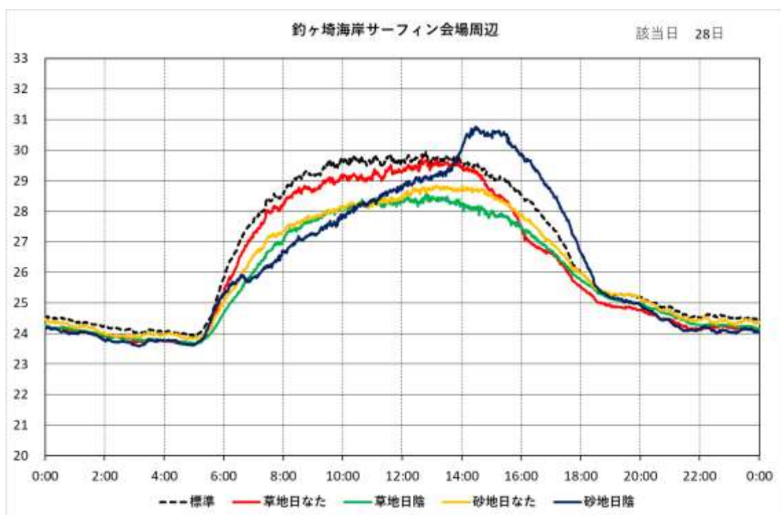
図 5-16(j) 時刻別 WBGT の日変化 (釣ヶ崎海岸サーフィン会場周辺)
