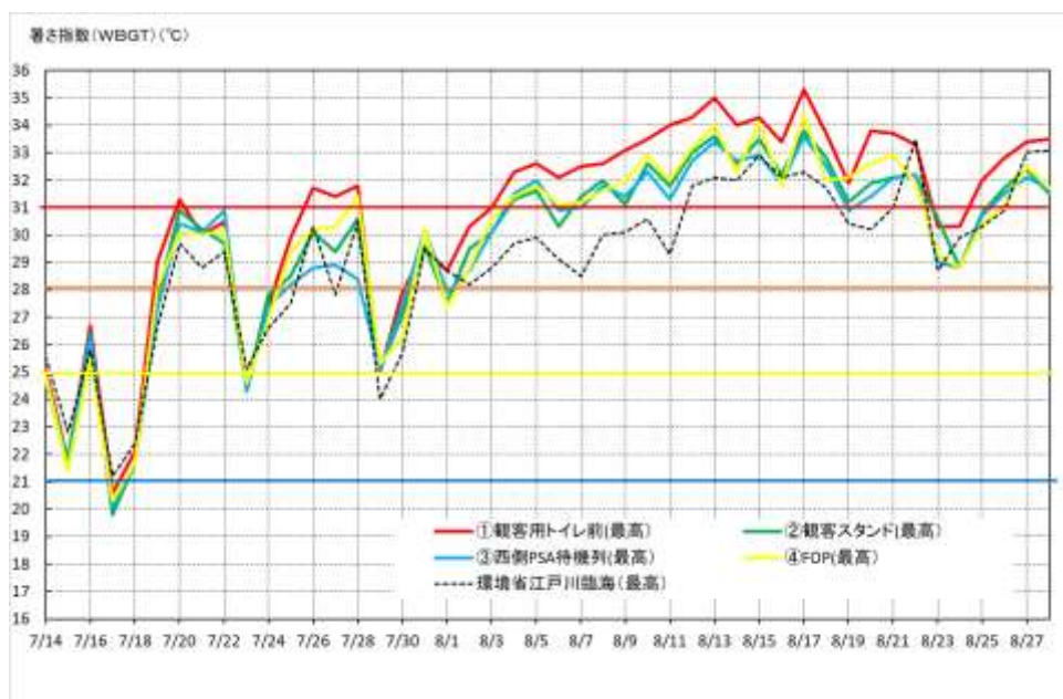
図 5-17 (c) カヌー・スラロームセンター及び比較地点での日最高 WBGT の変化
