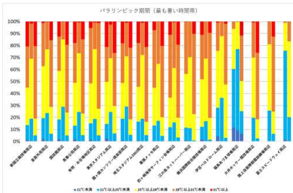
図 5-13(e) 運動指針で分けたパラリンピック期間の競技時間帯の標準型 WBGT 測定値の各年ごとの分布
