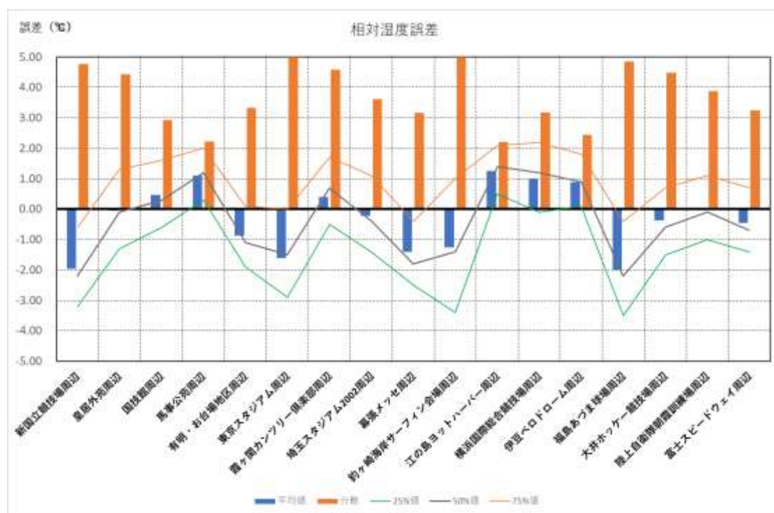
図 5-15 (d) 相対湿度の誤差の地区別の分布
