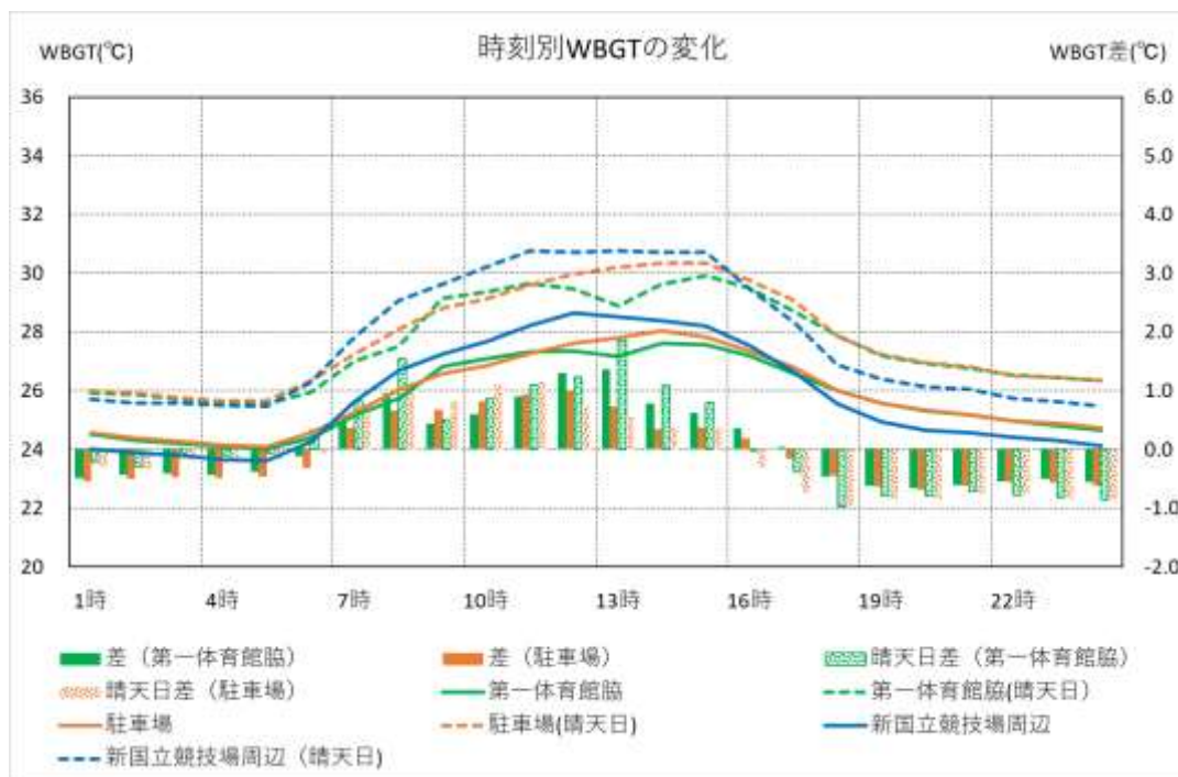
図 5-18(b) 国立代々木競技場及び比較地点での時刻別の WBGT の変化
