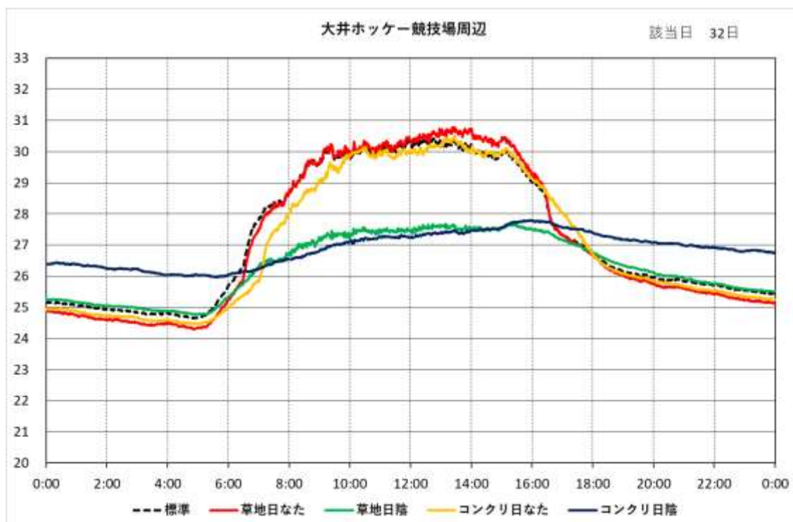
図 5-16 (o) 時刻別 WBGT の日変化 (大井ホッケー競技場周辺)
