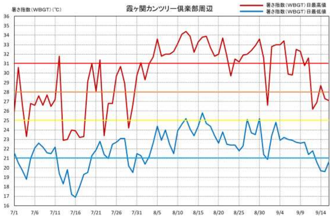
図 5-7 (g) WBGT 日最高値・日最低値の変化（霞ヶ関カントリー倶楽部周辺）
