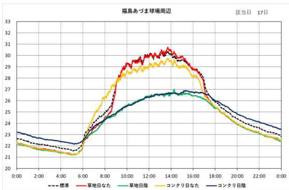
図 5-16 (n) 時刻別 WBGT の日変化 (福島あづま球場周辺)
