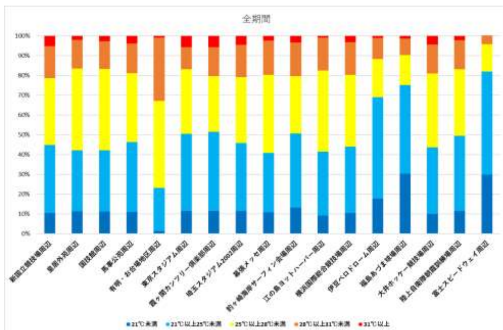
図 5-11(b) 運動指針で分けた全測定期間の標準型 WBGT 測定値の3年まとめた分布
