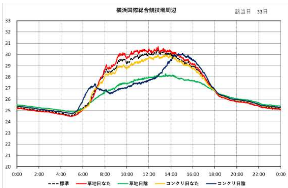
図 5-16(l) 時刻別 WBGT の日変化 (横浜国際総合競技場周辺)
