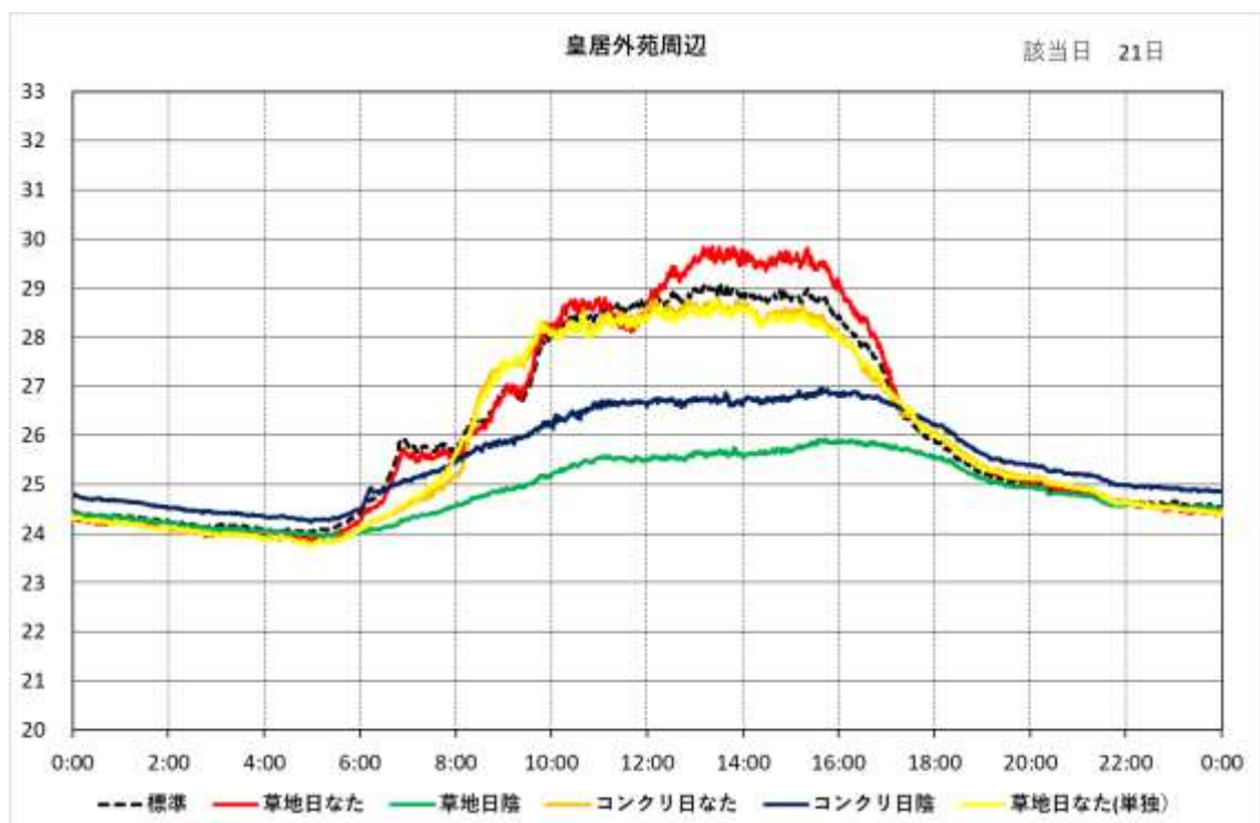
図 5-16(b) 時刻別 WBGT の日変化（皇居外苑周辺）
