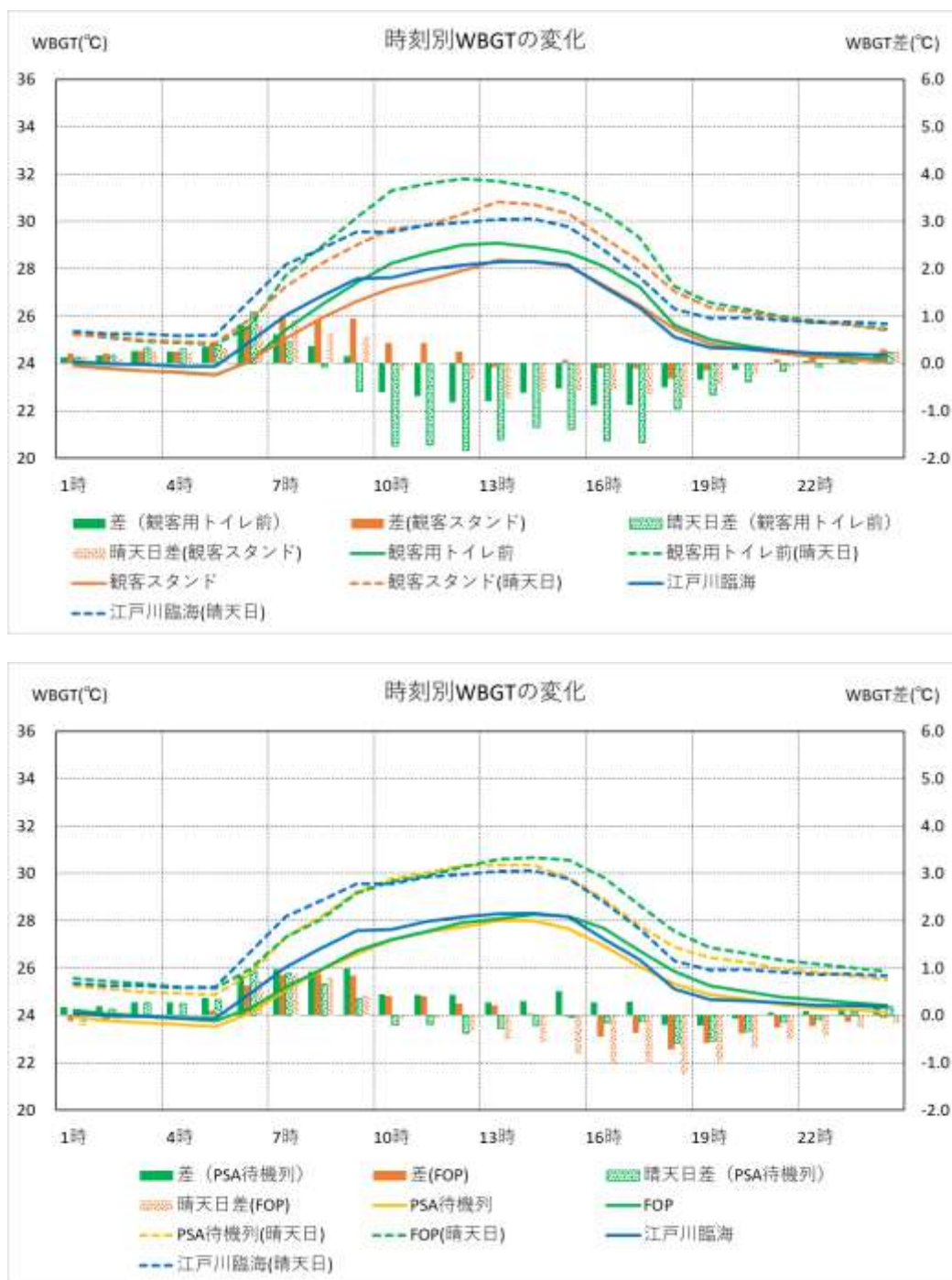
図 5-18(c) カヌー・スラロームセンター及び比較地点での時刻別の WBGT の変化
