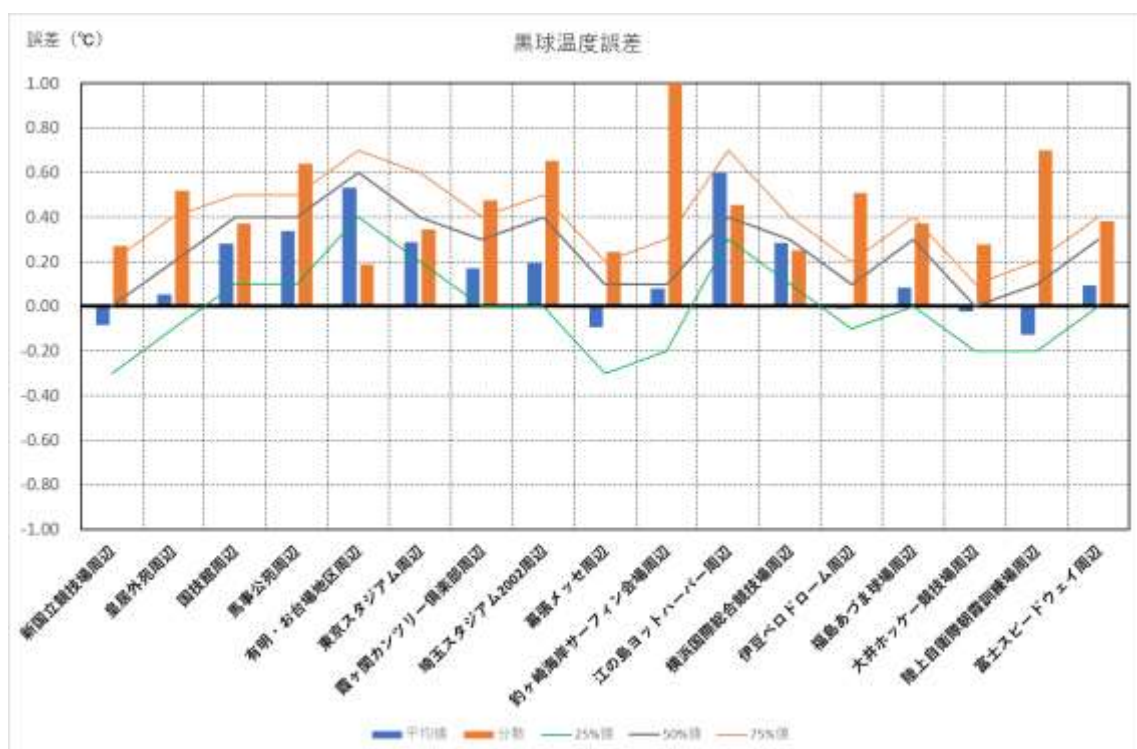
図 5-15(c) 黒球温度の誤差の地区別の分布
