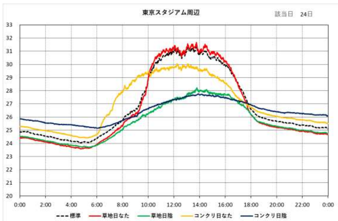
図 5-16 (f) 時刻別 WBGT の日変化 (東京スタジアム周辺)
