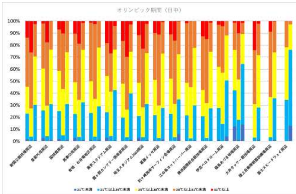
図 5-12(a) 運動指針で分けたオリンピック期間の日中の標準型 WBGT 測定値の各年ごとの分布
