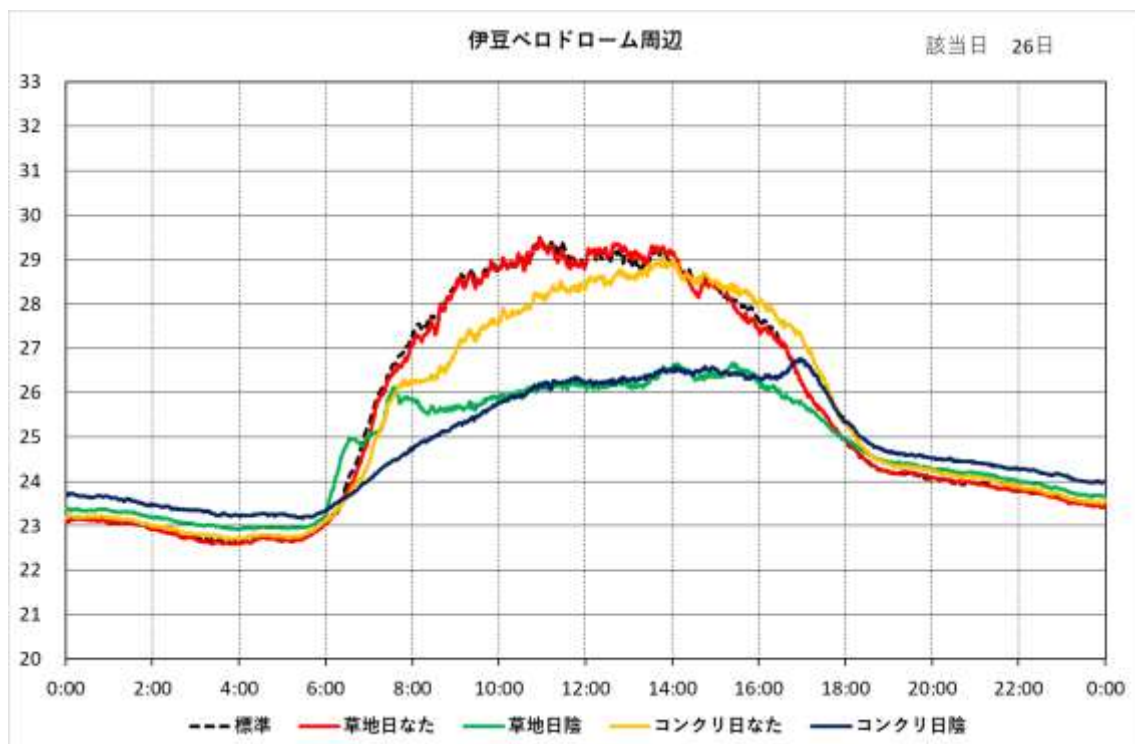
図 5-16 (m) 時刻別 WBGT の日変化 (伊豆ペロドローム周辺)
