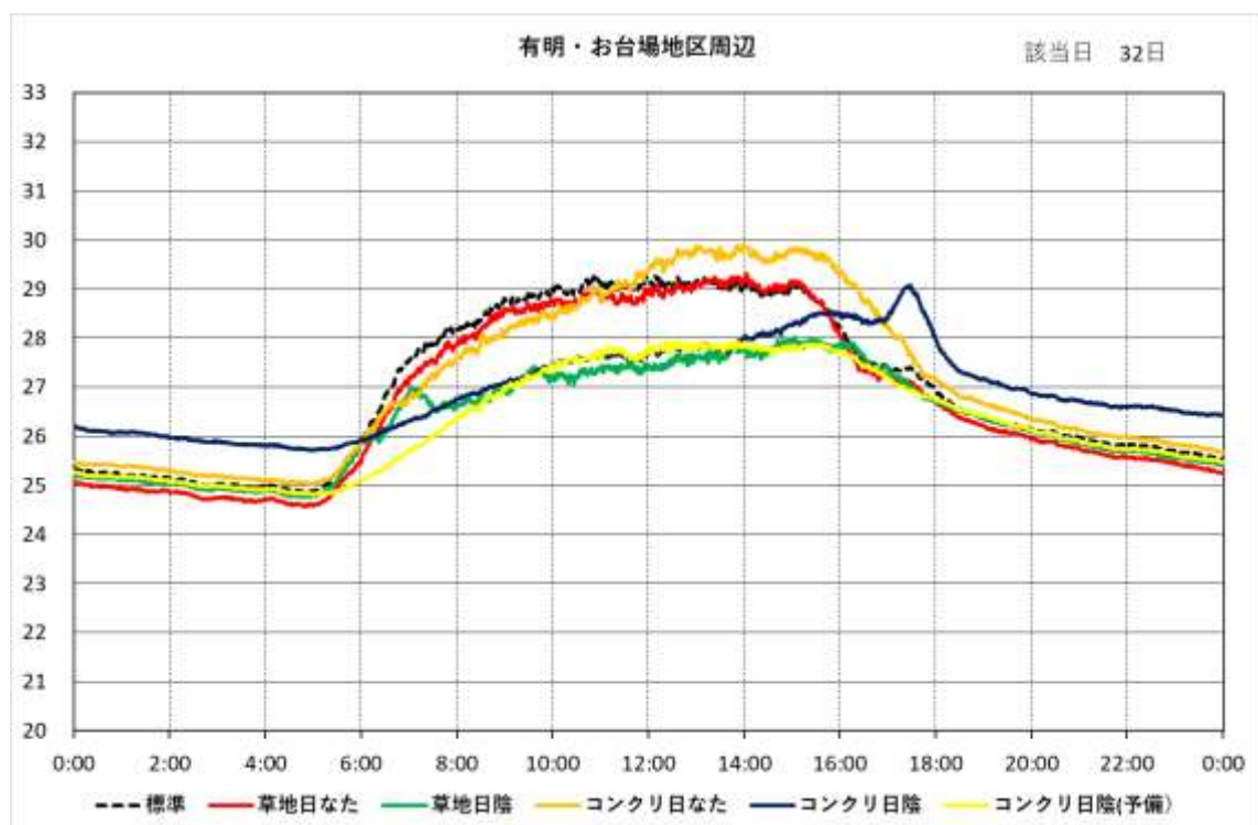
図 5-16 (e) 時刻別 WBGT の日変化 (有明・お台場地区周辺)
