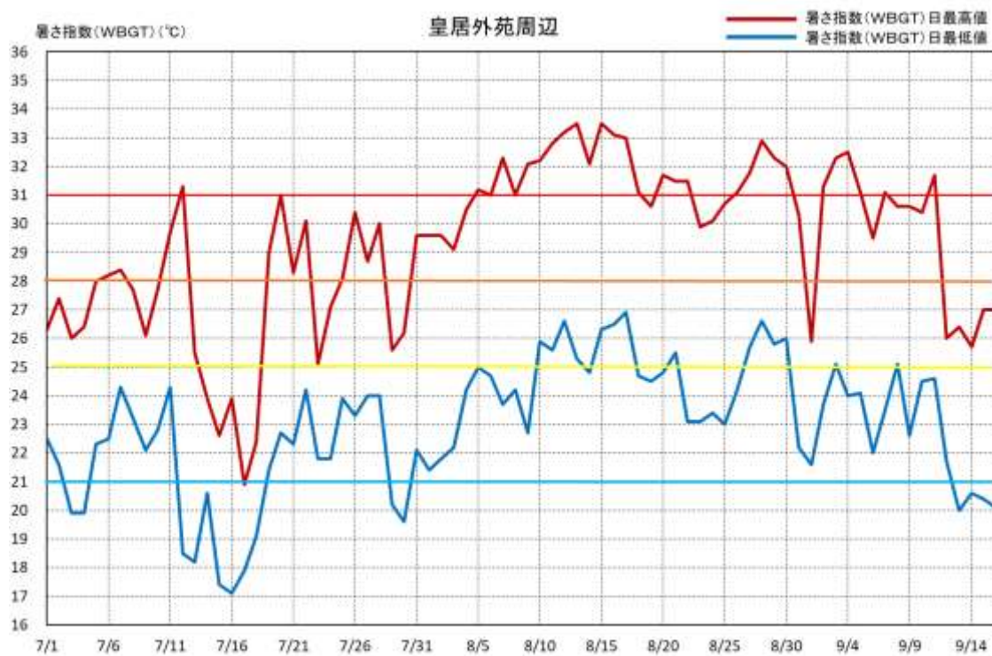
図 5-7 (b) WBGT 日最高値・日最低値の変化（皇居外苑周辺）
