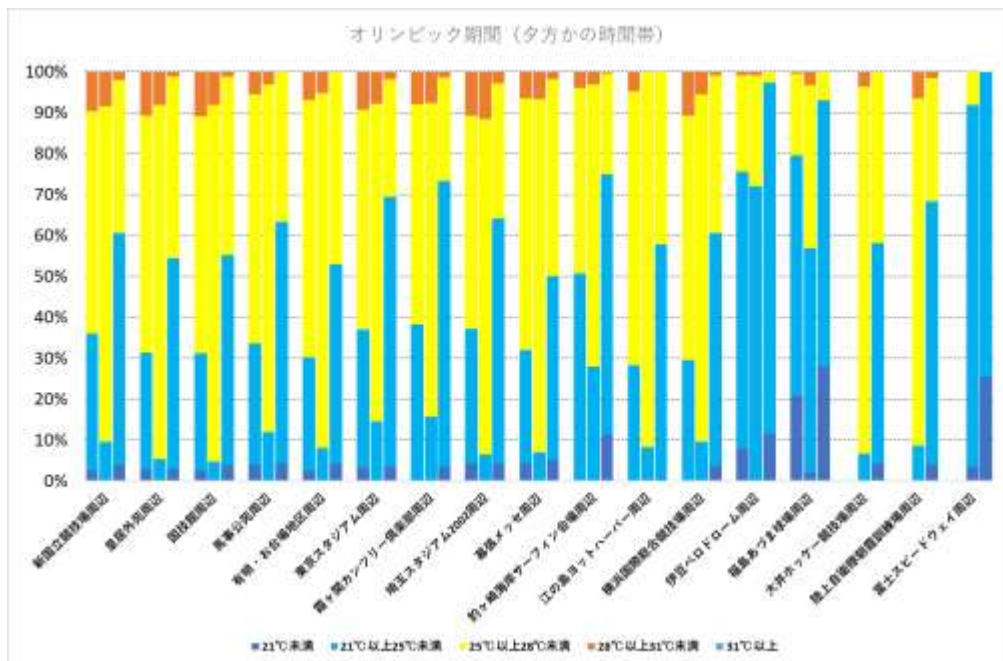
図 5-13(a) 運動指針で分けたパラリンピック期間の日中の標準型 WBGT 測定値の各年ごとの分布
