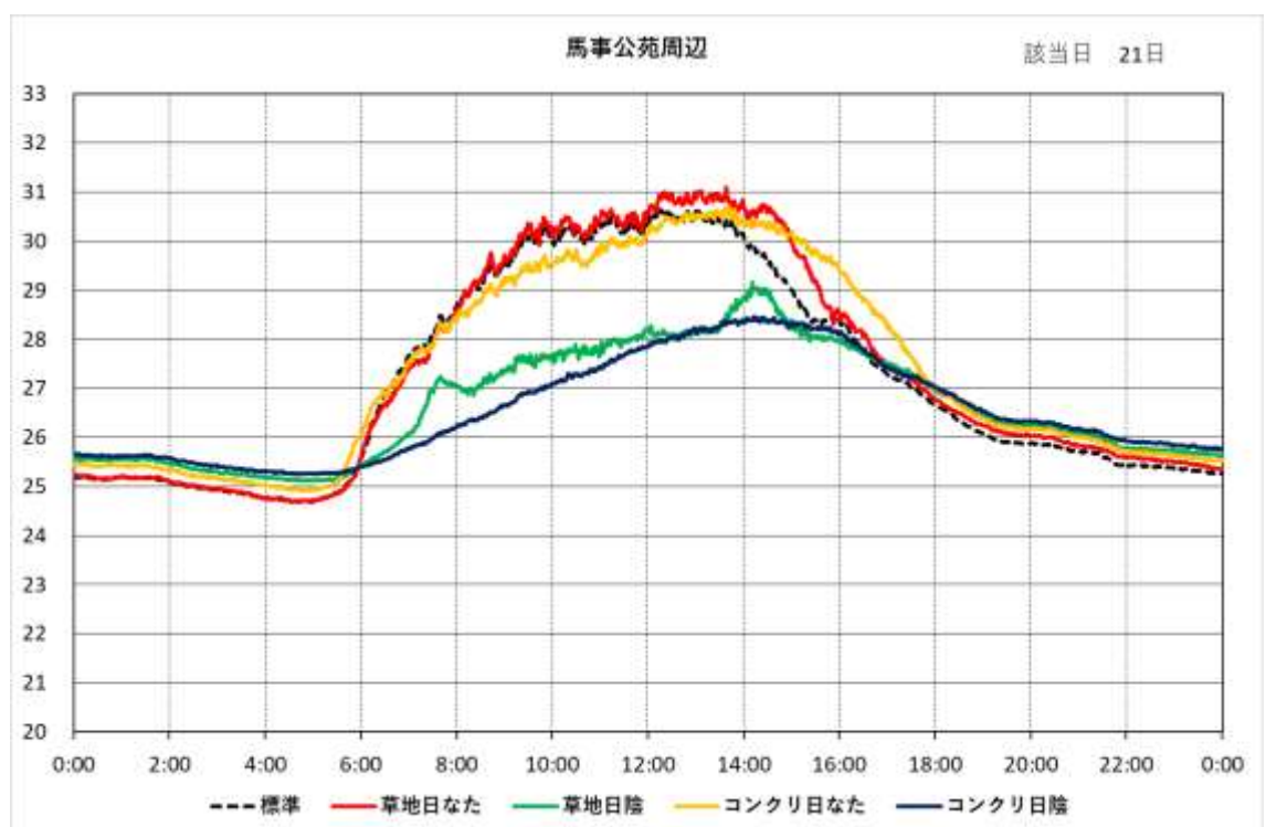
図 5-16 (d) 時刻別 WBGT の日変化 (馬事公苑周辺)
