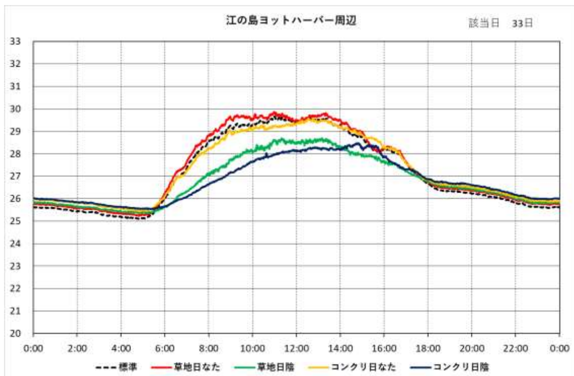
図 5-16(k) 時刻別 WBGT の日変化 (江の島ヨットハーバー周辺)
