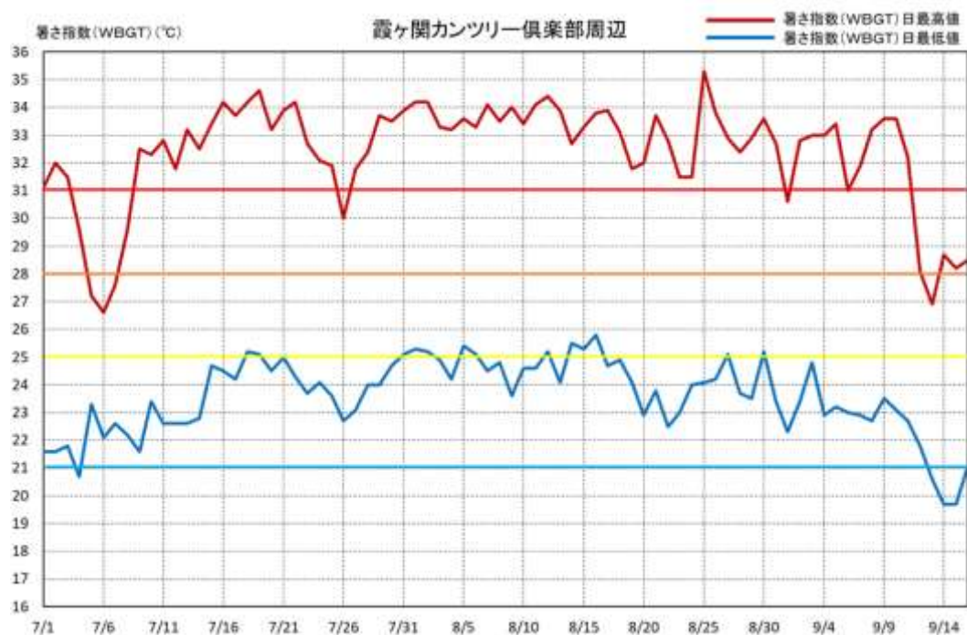
図 5-9-(b) 2018 年、2019 年、2020 年の各暦日の日最高値、日最低値の最高値（霞ヶ関カンツリー倶楽部周辺）の変化
