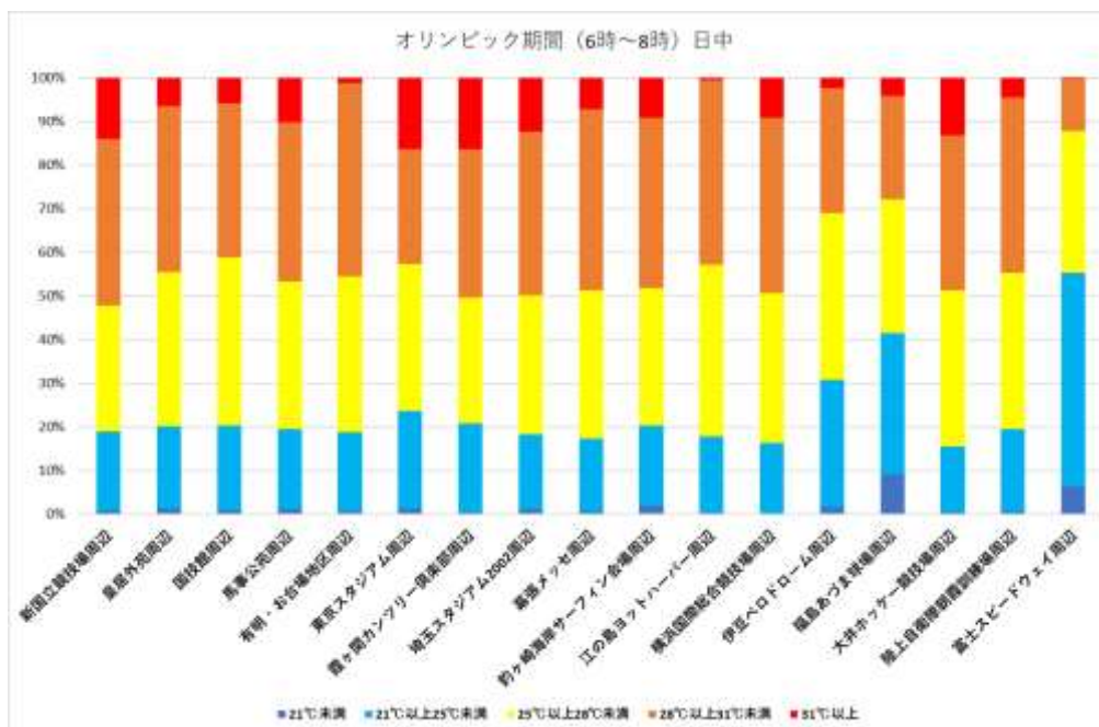
図 5-12(b) 運動指針で分けたオリンピック期間の日中の標準型 WBGT 測定値の 3 年まとめた分布
