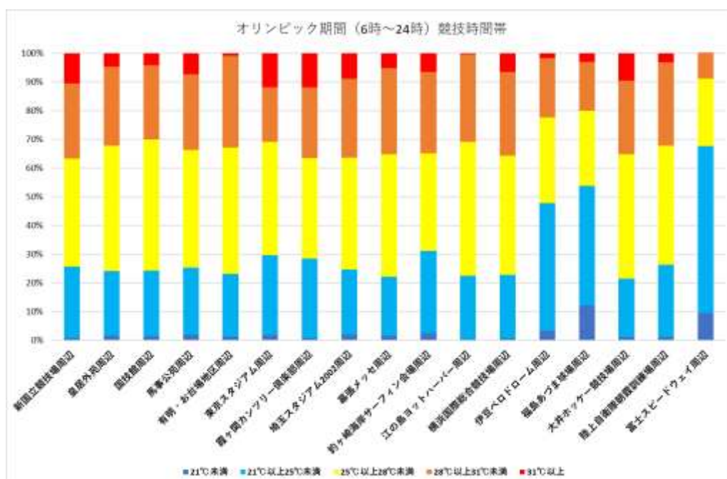
図 5-12(d) 運動指針で分けたオリンピック期間の競技時間帯の標準型 WBGT 測定値の 3 年まとめた分布
