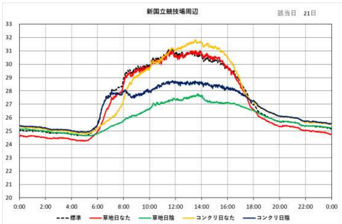
図 5-16(a) 時刻別 WBGT の日変化（新国立競技場周辺）
