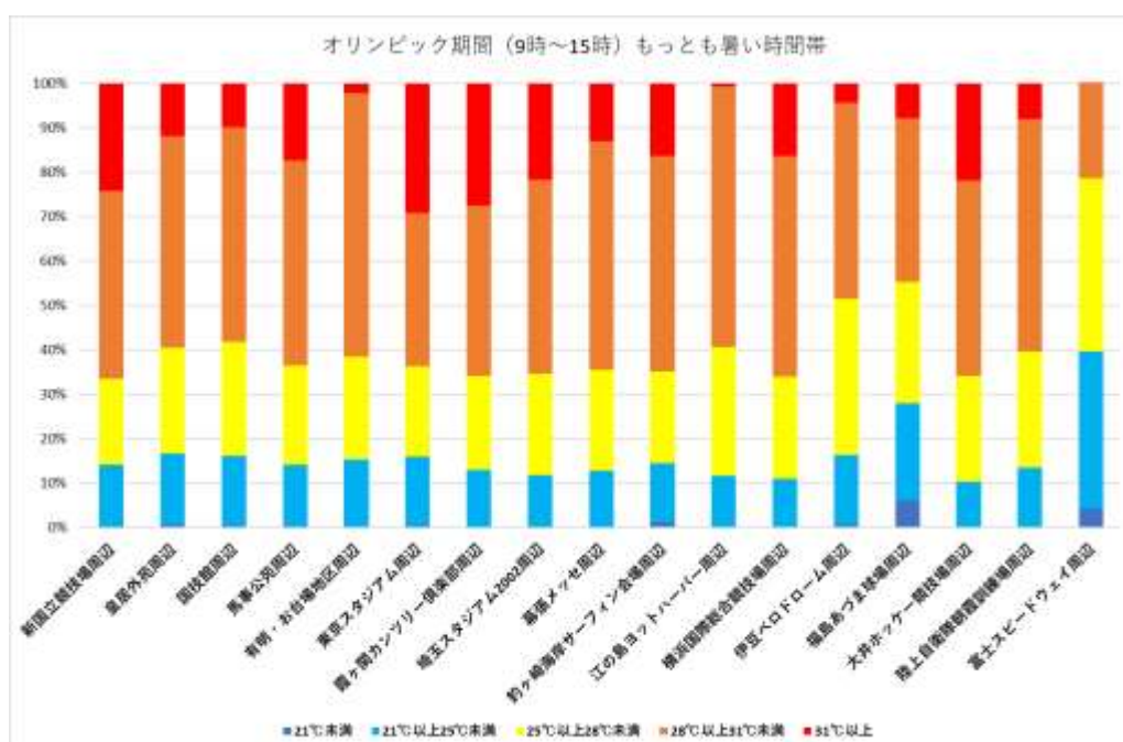
図 5-12(f) 運動指針で分けたオリンピック期間の競技時間帯の標準型 WBGT 測定値の3年まとめた分布
