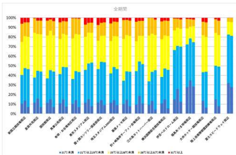
図 5-11(a) 運動指針で分けた全測定期間の標準型 WBGT 測定値の各年ごとの分布
