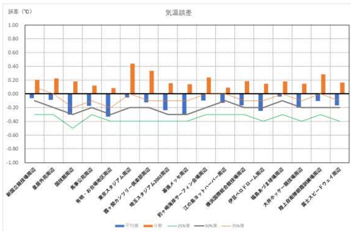
図 5-15 (b) 気温の誤差の地区別の分布
