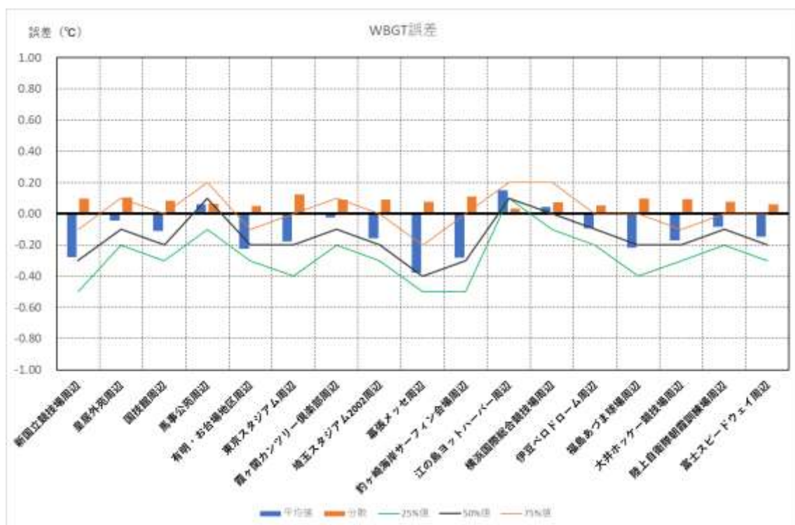
図 5-15(a) WBGT の誤差の地区別の分布
