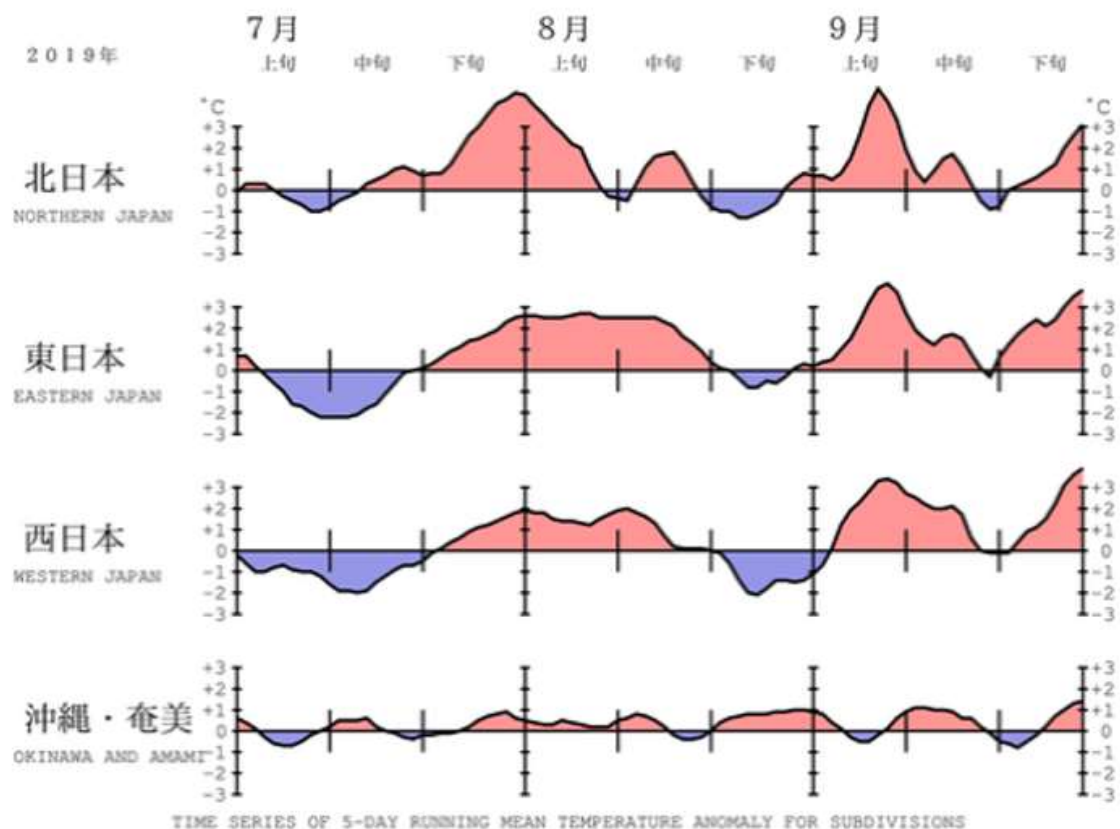
図 5-1(c) 地域平均気温の年間偏差の 5 日移動平均時系列 (2019 年)
