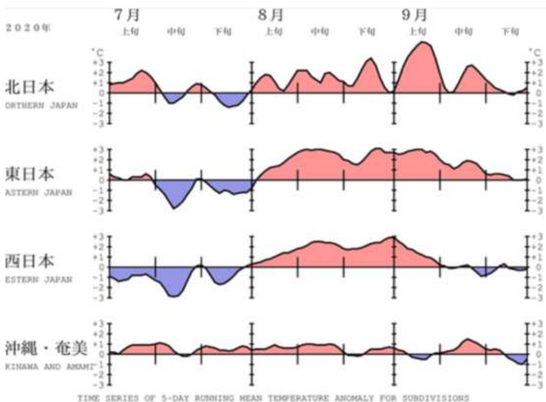
図5-1(a) 地域平均気温の平年偏差の5日移動平均時系列(2020年)
