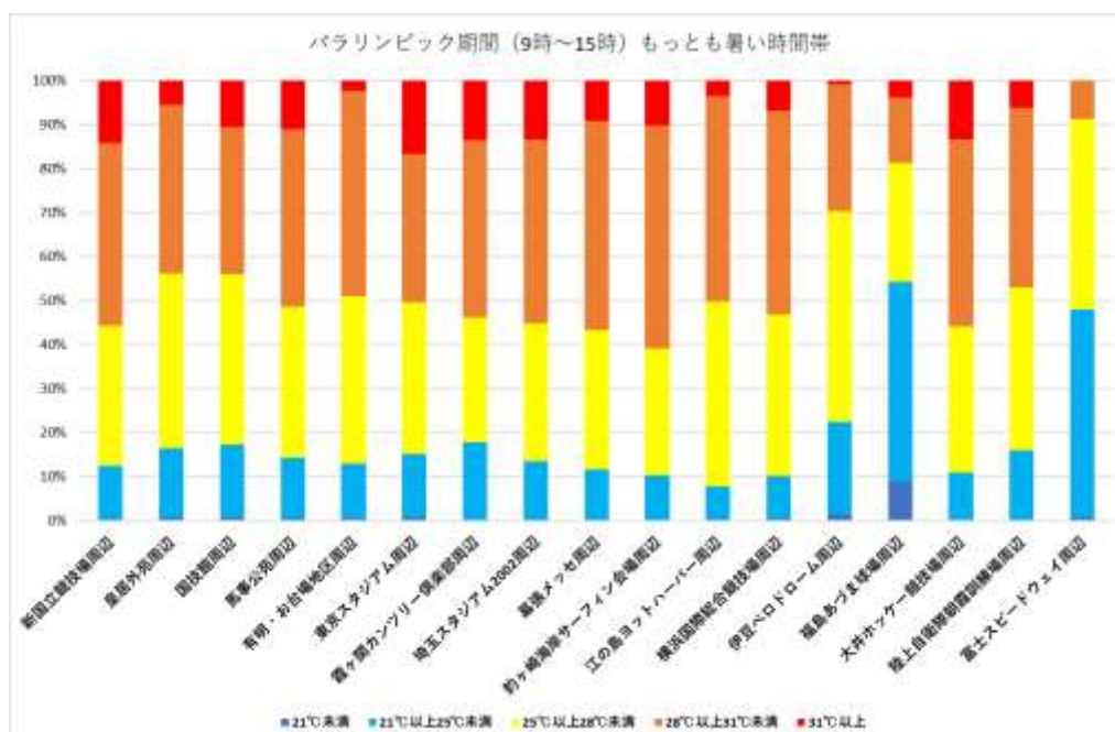
図 5-13(f) 運動指針で分けたパラリンピック期間の競技時間帯の標準型 WBGT 測定値の3年まとめた分布
