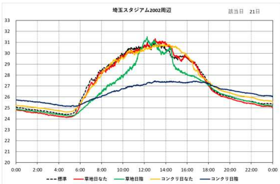
図 5-16 (h) 時刻別 WBGT の日変化（埼玉スタジアム 2002 周辺）
