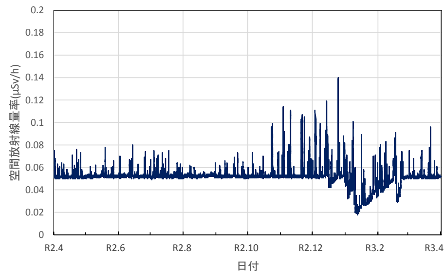
新潟県糸魚川市 糸魚川地域振興局の空間放射線量率(10分値使用)
