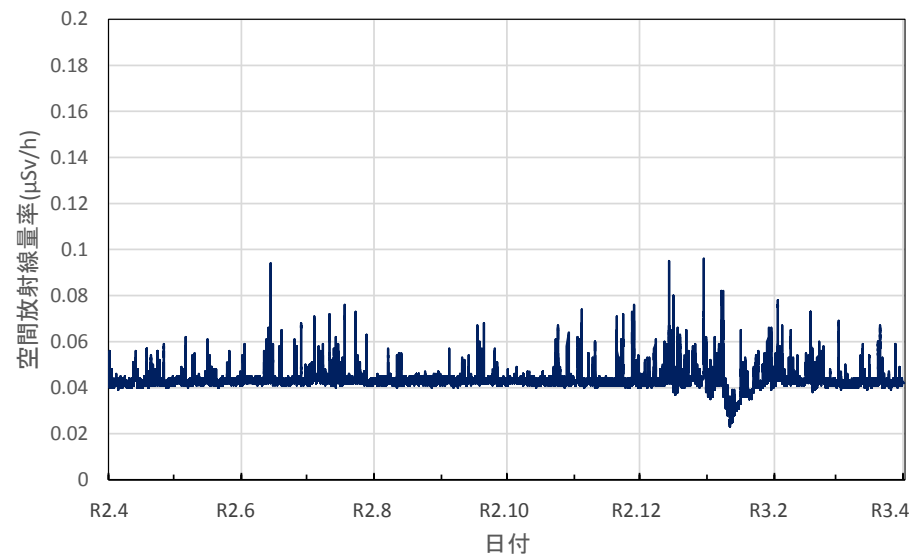
福井県永平寺町 永平寺町役場の空間放射線量率(10分値使用)
