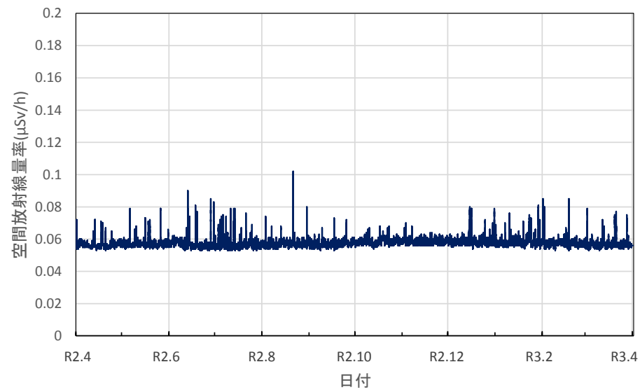
岐阜県岐阜市 防災交流センターの空間放射線量率(10分値使用)
