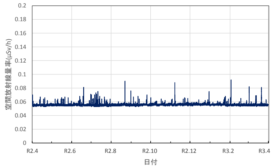
京都府京都市 保健環境研究所の空間放射線量率(10分値使用)
