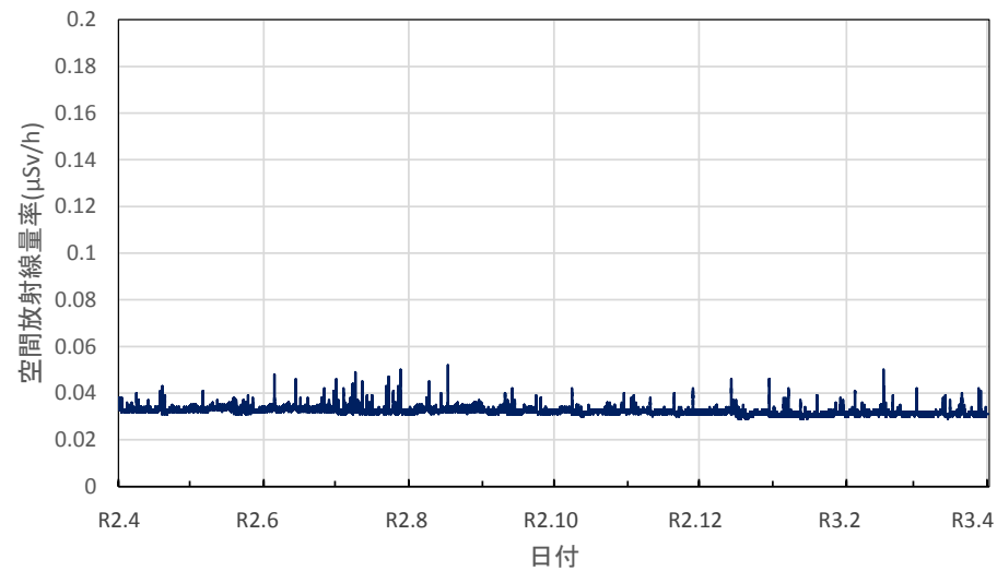
宮城県気仙沼市 気仙沼保健福祉事務所の空間放射線量率(10分値使用)
