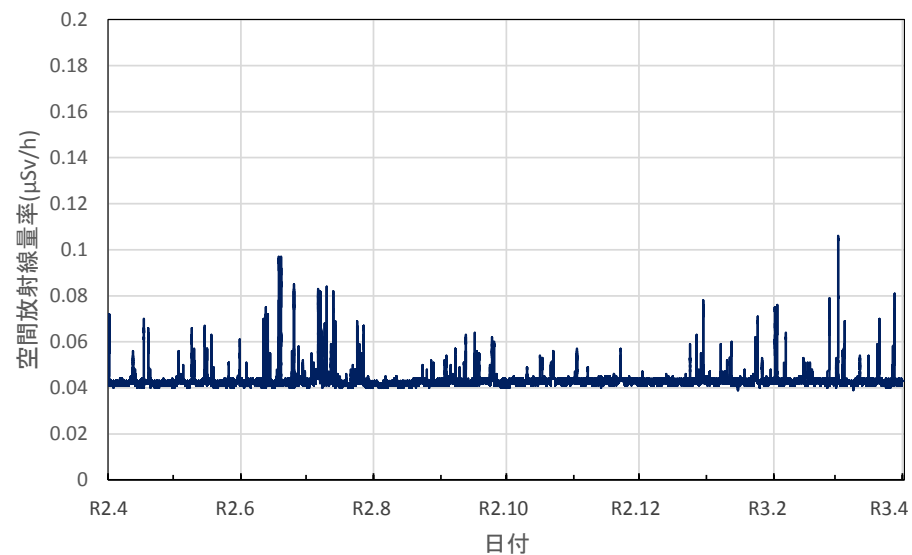
長崎県平戸市 県北保健所の空間放射線量率(10分値使用)
