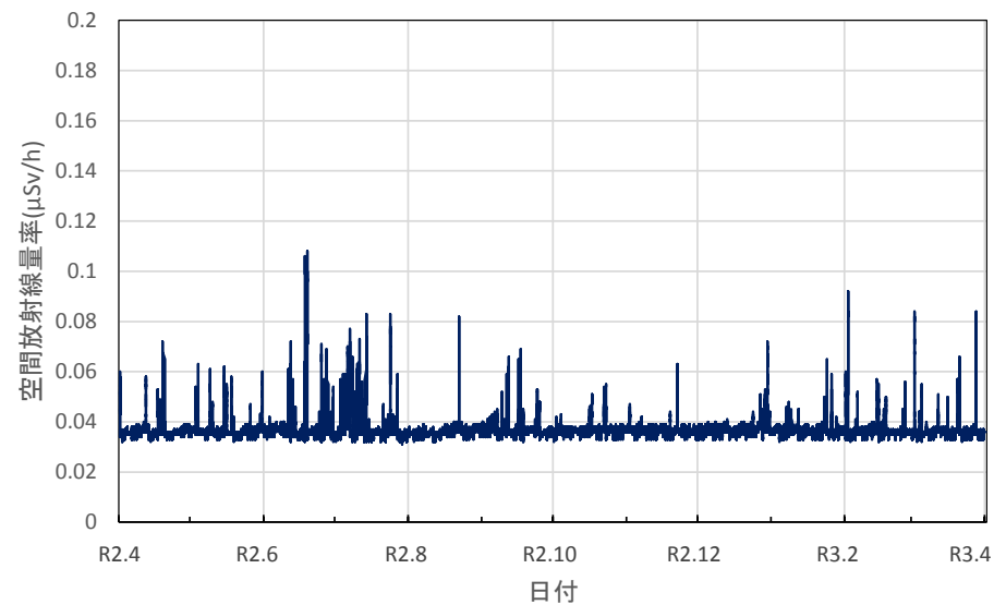
福岡県久留米市 久留米総合庁舎の空間放射線量率(10分値使用)
