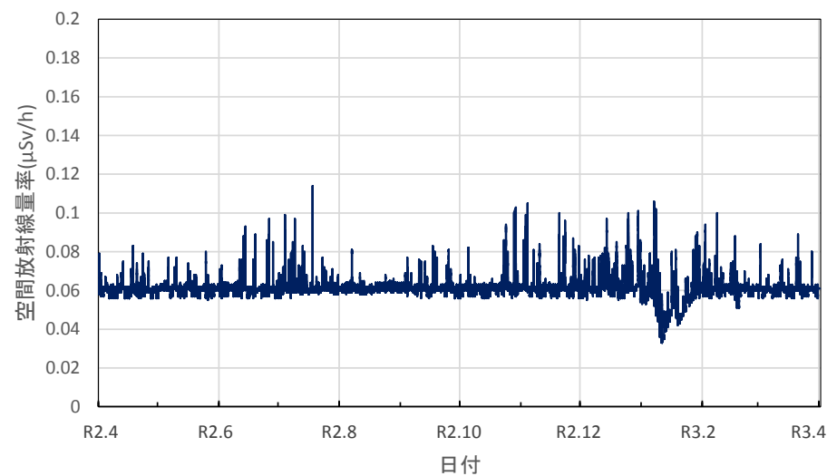
石川県津幡町 県石川中央保健福祉センター 河北地域センターの空間放射線量率(10分値使用)
