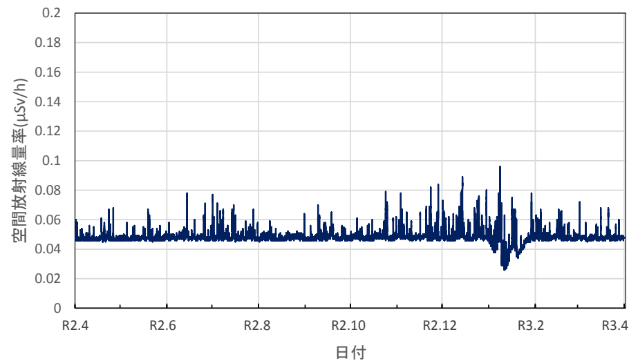
新潟県新潟市 放射線監視センター新潟分室の空間放射線量率(10分 値使用)
