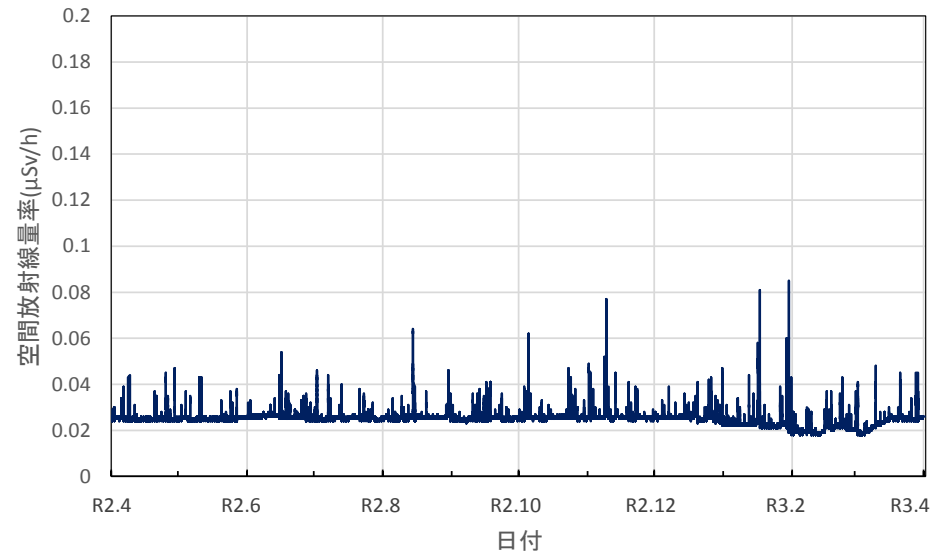
北海道室蘭市 胆振総合振興局の空間放射線量率(10分値使用)
