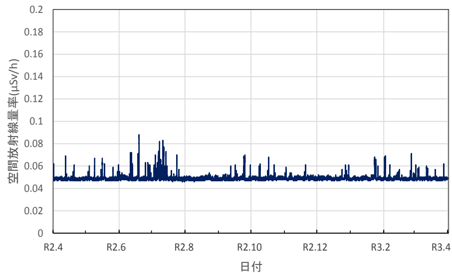
大分県大分市 県衛生環境研究センターの空間放射線量率(10分値使用)
