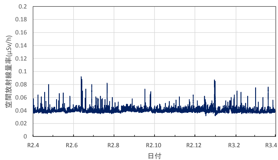
京都府南丹市 南丹土木事務所美山出張所の空間放射線量率(10分値使用)
