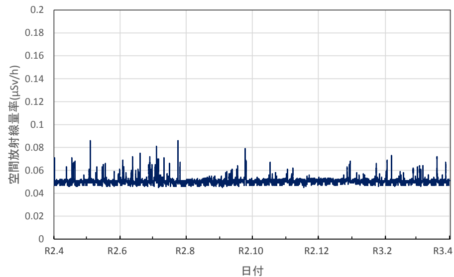
宮崎県小林市 小林保健所の空間放射線量率(10分値使用)
