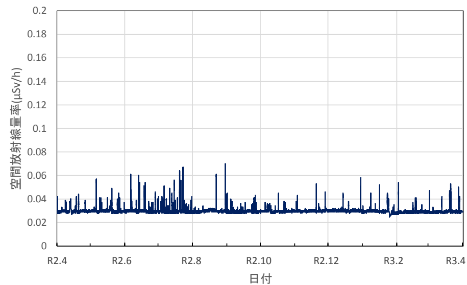
長野県軽井沢町 軽井沢町役場の空間放射線量率(10分値使用)
