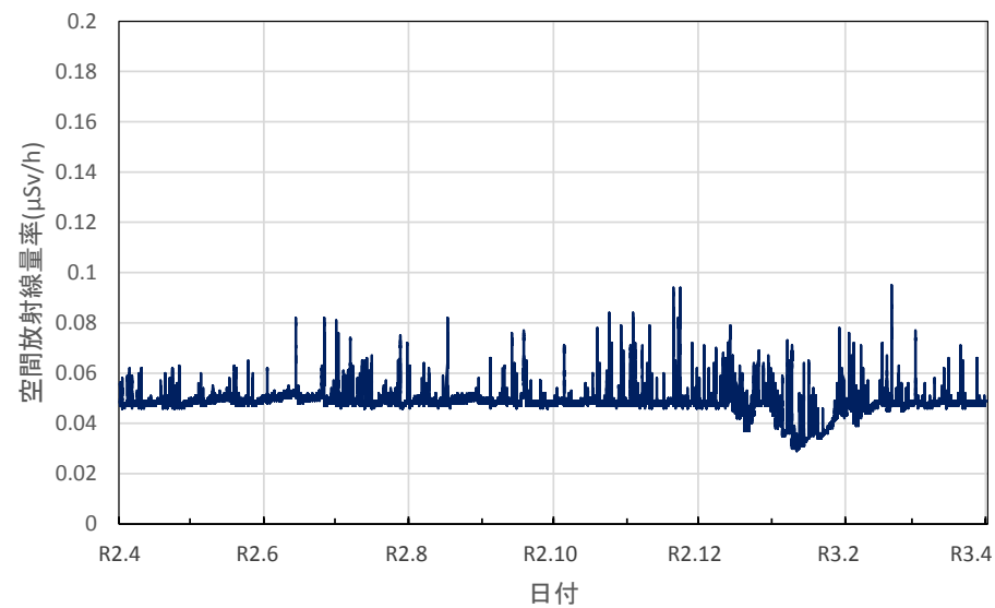
山形県三川町 庄内総合支庁の空間放射線量率(10分値使用)
