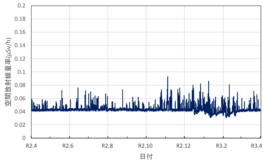
新潟県長岡市 長岡地域振興局の空間放射線量率(10分値使用)
