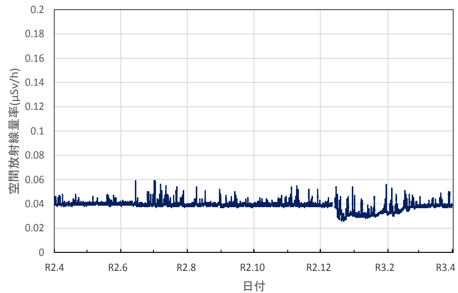
岩手県奥州市 奥州地区合同庁舎の空間放射線量率(10分値使用)
