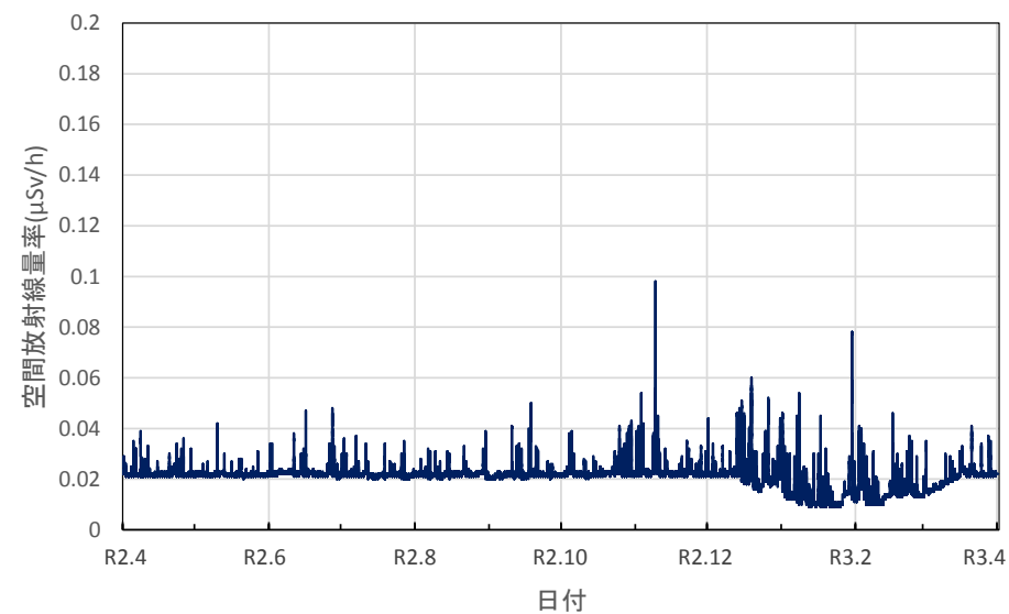
青森県むつ市 むつ市役所川内庁舎の空間放射線量率(10分値使用)
