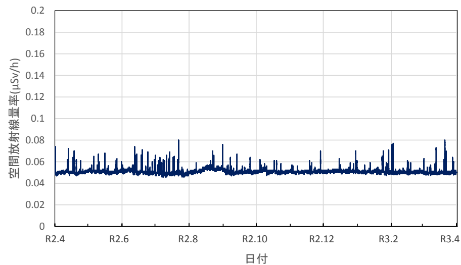
愛知県設楽町 新城設楽建設事務所設楽支所の空間放射線量率(10 分値使用)
