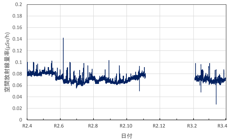
広島県三次市 北部厚生環境事務所の空間放射線量率(10分値使用)
