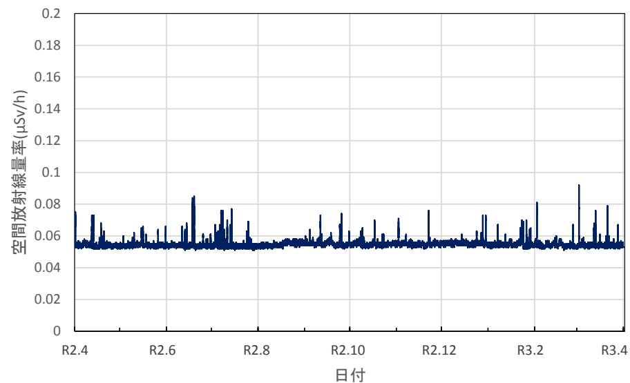
香川県丸亀市 中讃保健福祉事務所の空間放射線量率(10分値使用)
