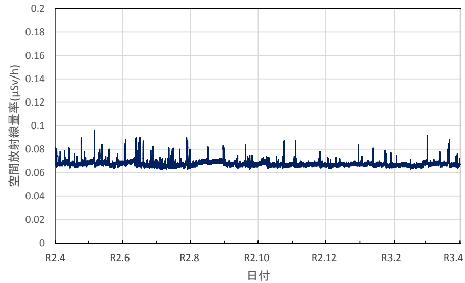
茨城県北茨城市 北茨城市役所の空間放射線量率(10分値使用)
