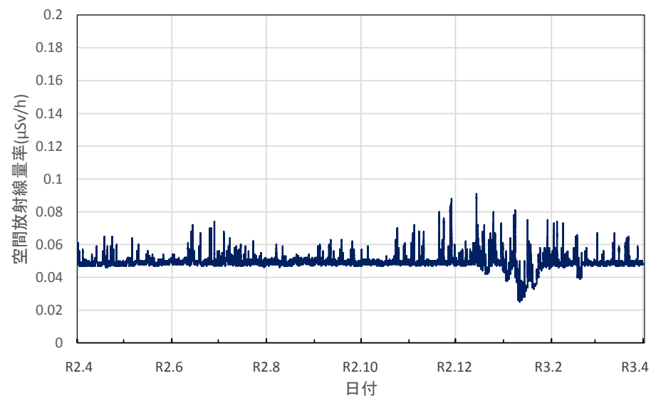
石川県金沢市 県保健環境センターの空間放射線量率(10分値使用)
