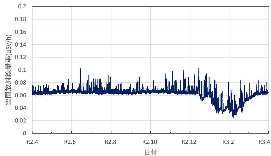
新潟県阿賀町 新潟地域振興局津川庁舎の空間放射線量率(10分値使用)
