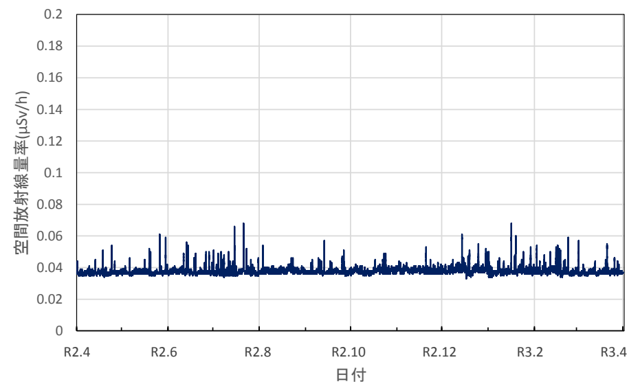
長野県長野市 環境保全研究所の空間放射線量率(10分値使用)
