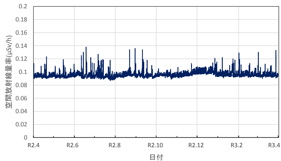
山口県山口市 県環境保健センター大蔵庁舎の空間放射線量率(10分値使用)
