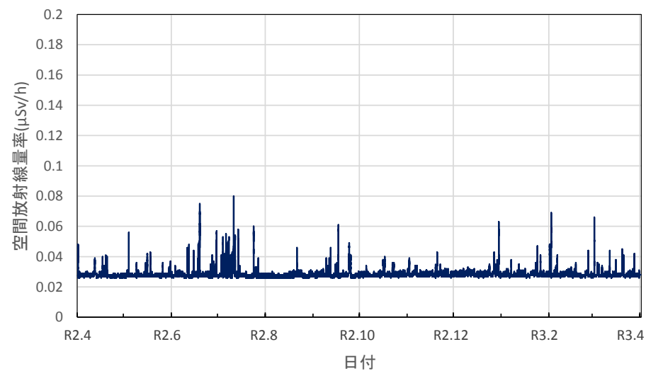
熊本県宇土市 県保健環境科学研究所の空間放射線量率(10分値使用)
