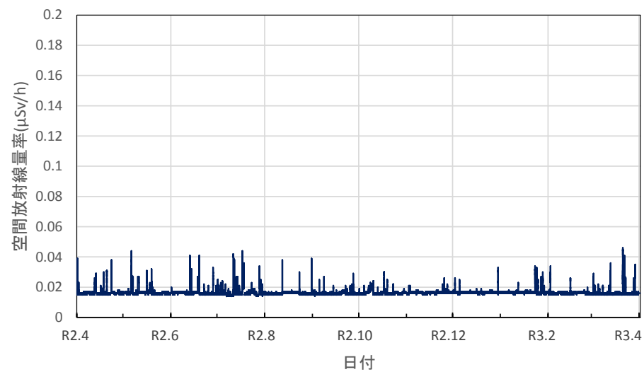
神奈川県小田原市 県立小田原城北工業高等学校の空間放射線量率 (10分値使用)
