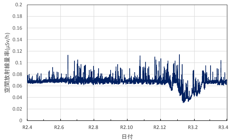
新潟県村上市 村上地域振興局の空間放射線量率(10分値使用)
