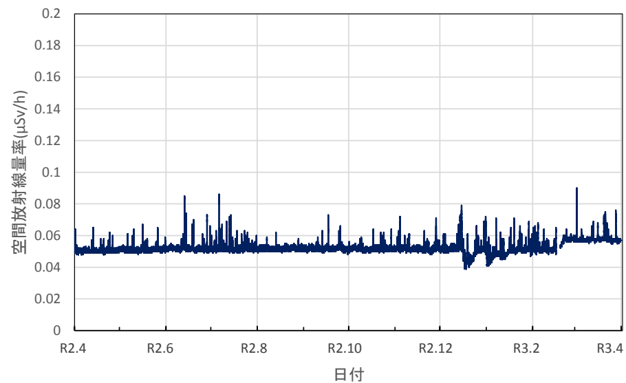
滋賀県長浜市 県木之本合同庁舎の空間放射線量率(10分値使用)
