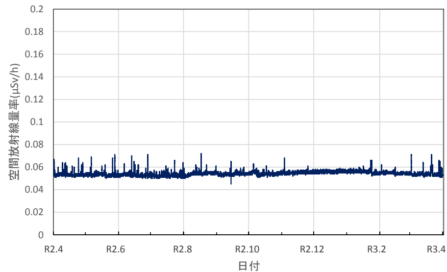
栃木県宇都宮市 子ども総合科学館の空間放射線量率(10分値使用)
