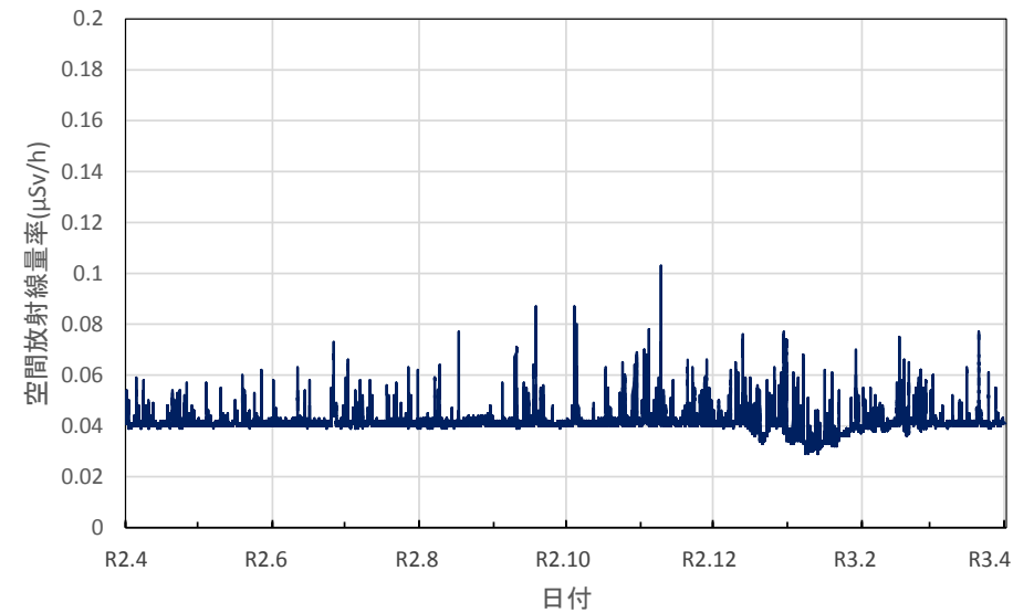
秋田県能代市 山本地域振興局の空間放射線量率(10分値使用)
