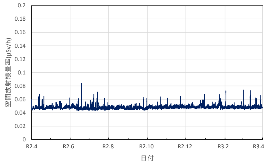
岡山県岡山市 県環境保健センターの空間放射線量率(10分値使用)
