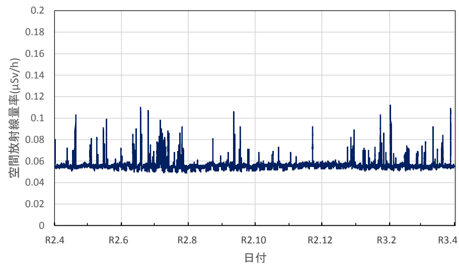
山口県下関市 西部高等産業技術学校の空間放射線量率(10分値使用)
