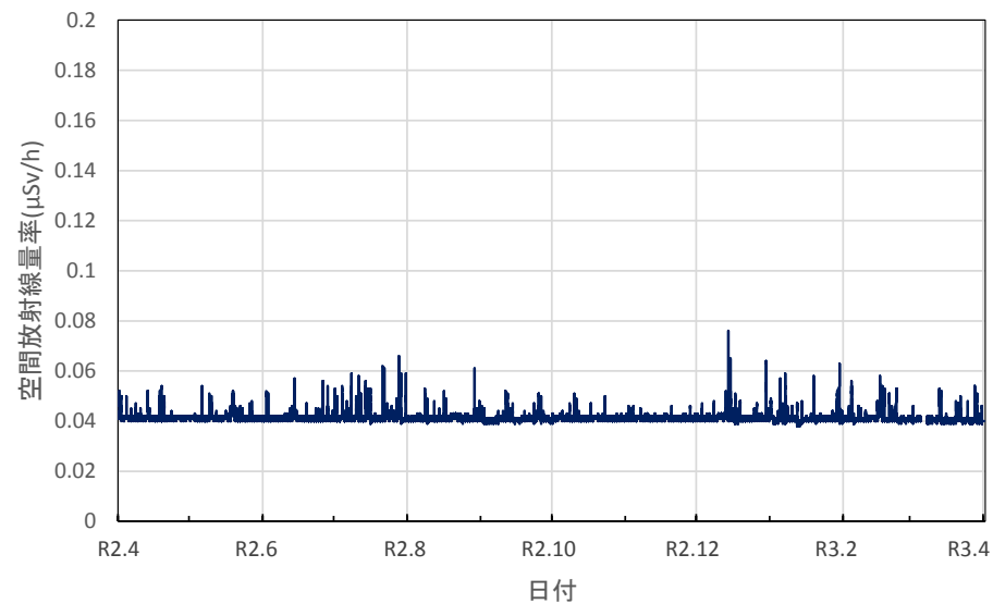
宮城県大河原町 大河原合同庁舎の空間放射線量率(10分値使用)
