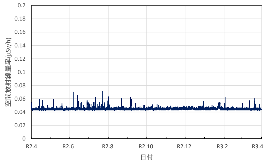
山梨県甲府市 県衛生環境研究所の空間放射線量率(10分値使用)
