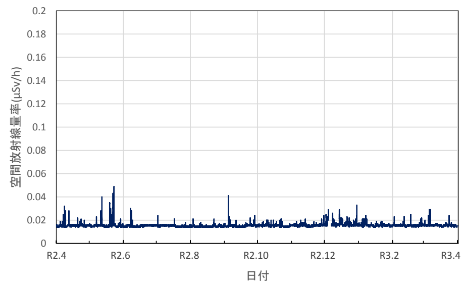
沖縄県石垣市 八重山福祉保健所の空間放射線量率(10分値使用)
