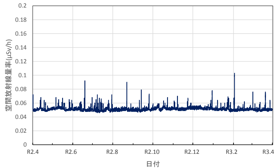
京都府木津川市 木津総合庁舎の空間放射線量率(10分値使用)
