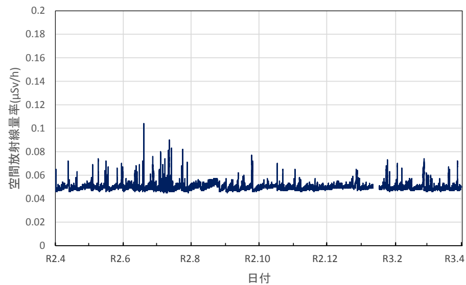
大分県佐伯市 佐伯豊南高等学校の空間放射線量率(10分値使用)
