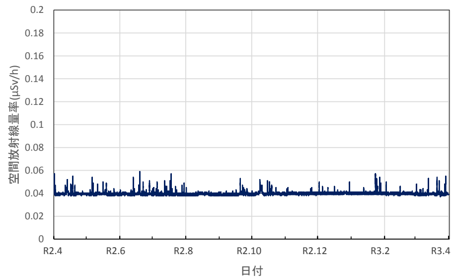
神奈川県逗子市 県立逗葉高等学校の空間放射線量率(10分値使用)
