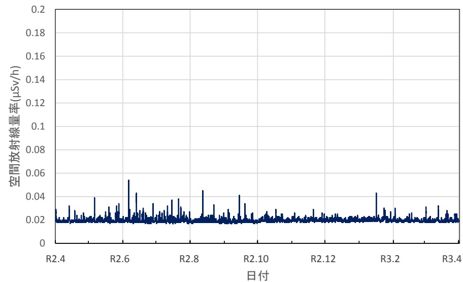
群馬県前橋市 県衛生環境研究所の空間放射線量率(10分値使用)
