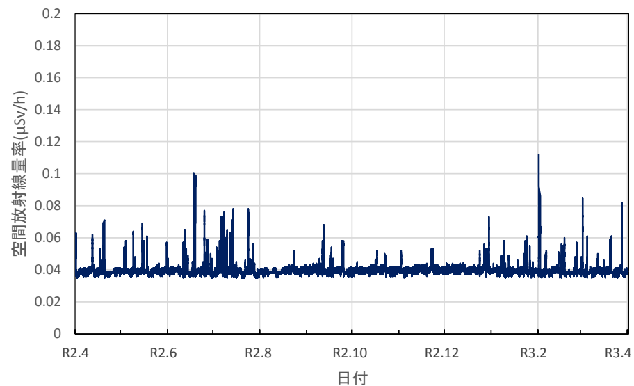
福岡県飯塚市 飯塚総合庁舎の空間放射線量率(10分値使用)
