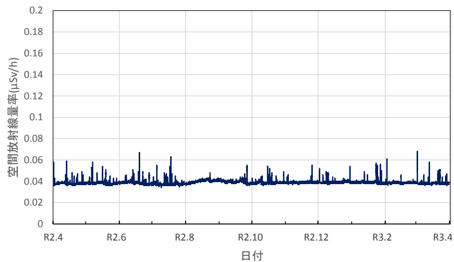
千葉県茂原市 県大気汚染常時監視測定局の空間放射線量率(10分値使用)
