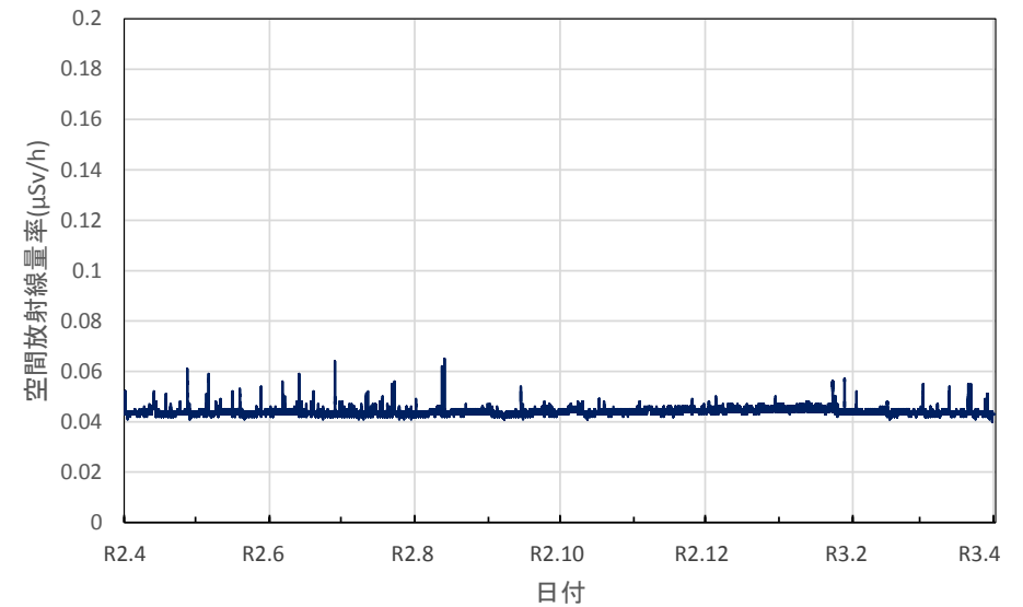
埼玉県さいたま市 埼玉県庁の空間放射線量率(10分値使用)
