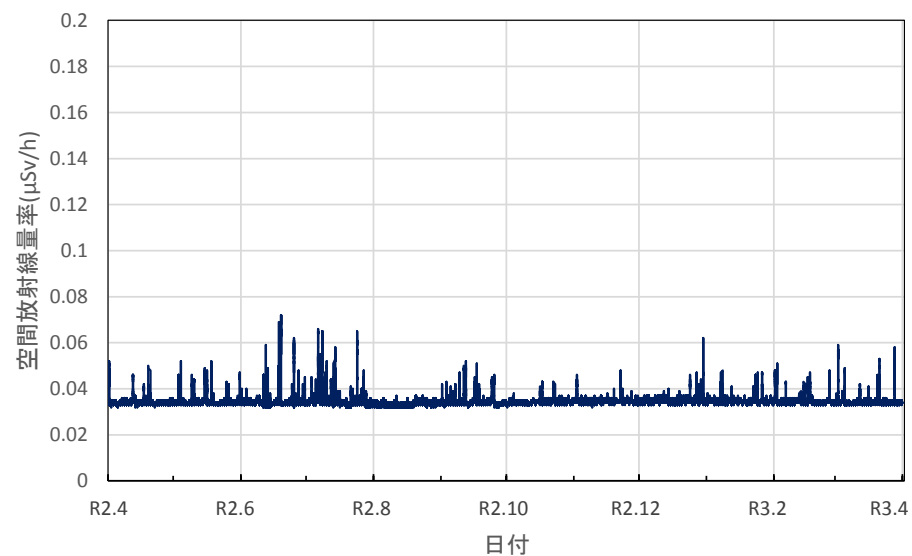
福岡県太宰府市 県保健環境研究所の空間放射線量率(10分値使用)
