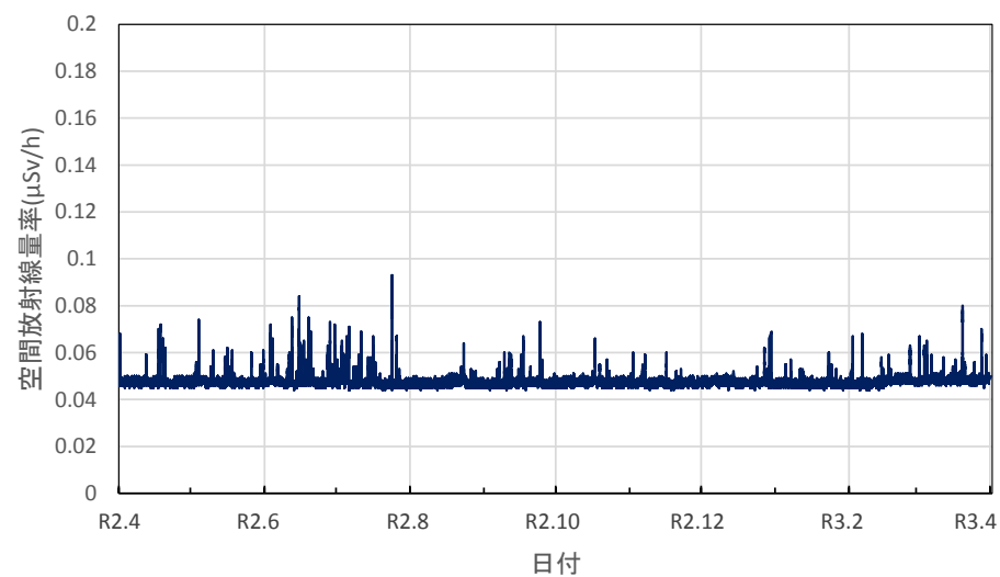
鹿児島県霧島市 始良・伊佐地域振興局霧島庁舎の空間放射線量率(10分値使用)
