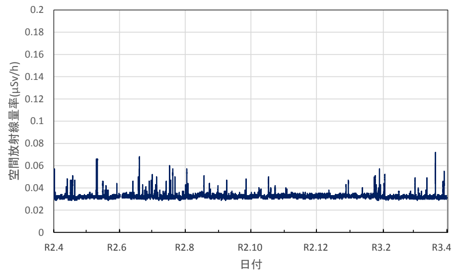
静岡県静岡市 県工業技術研究所の空間放射線量率(10分値使用)
