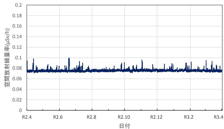
香川県さぬき市 東讃保健福祉事務所の空間放射線量率(10分値使用)
