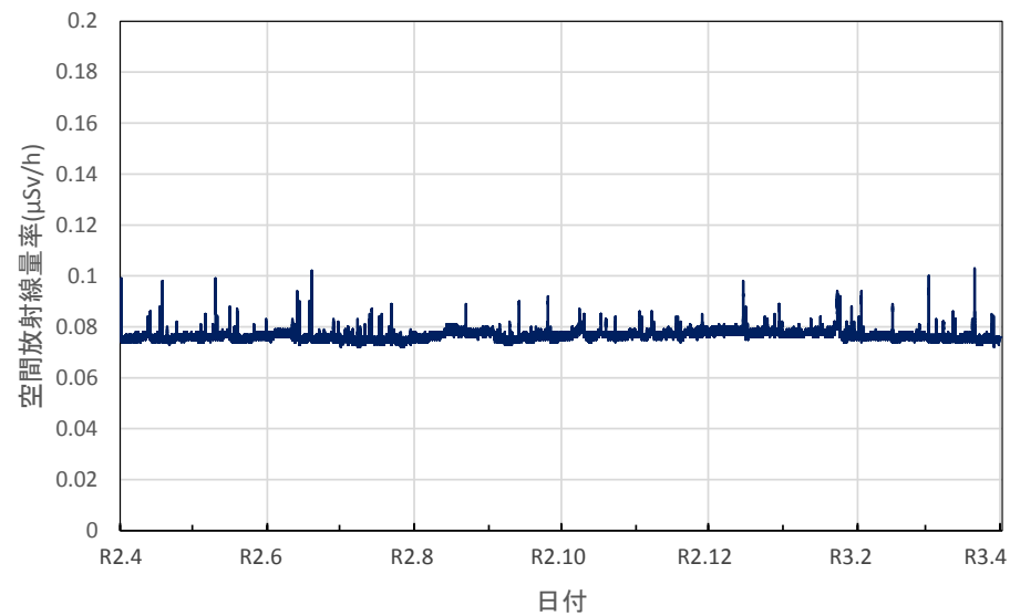
愛知県岡崎市 西三河県民事務所の空間放射線量率(10分値使用)
