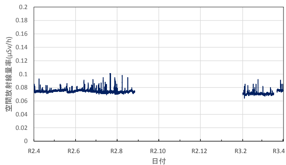
福島県二本松市 県男女共生センターの空間放射線量率(10分値使用)
