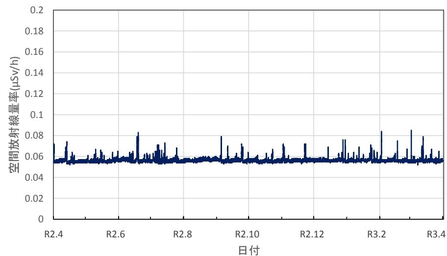
香川県観音寺市 西讃保健福祉事務所の空間放射線量率(10分値使用)
