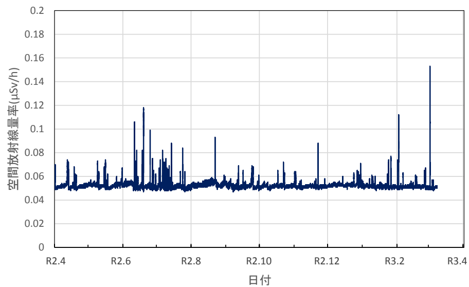
愛媛県八幡浜市 市立武道館の空間放射線量率(10分値使用)
