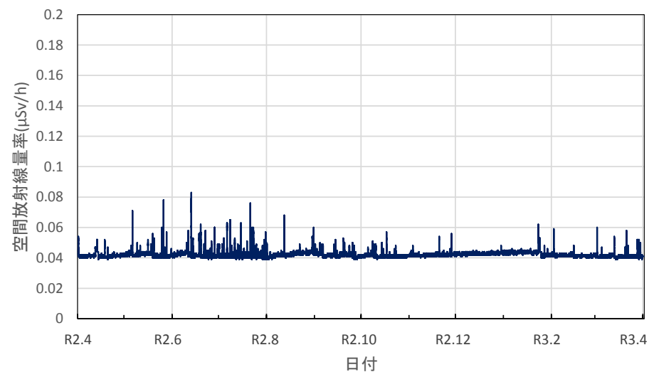
群馬県富岡市 富岡市生涯学習センターの空間放射線量率(10分値使用)
