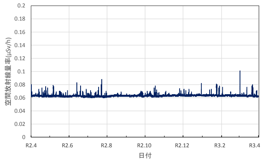
千葉県香取市 小見川市民センターの空間放射線量率(10分値使用)
