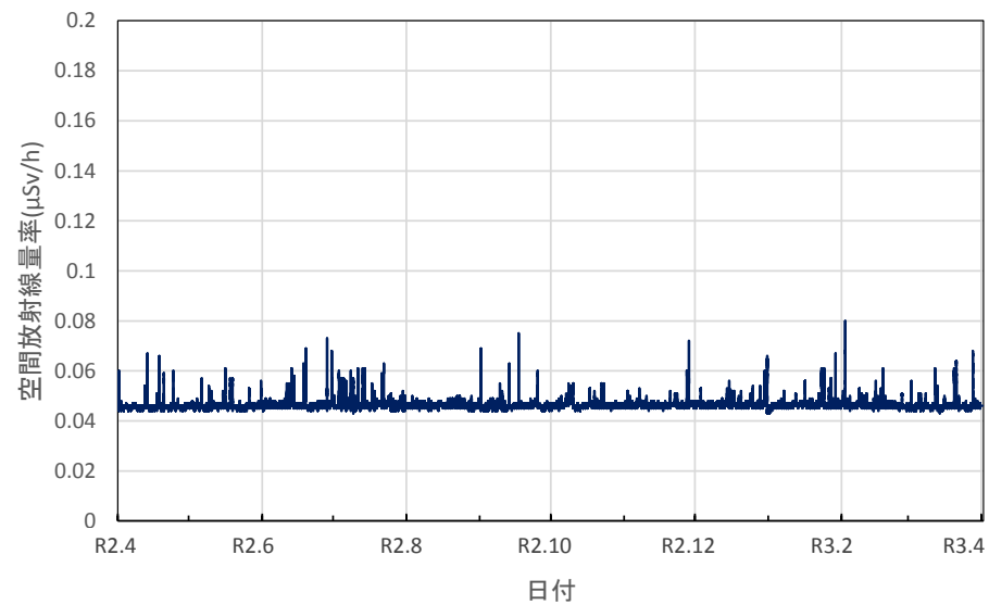
三重県四日市市 県保健環境研究所の空間放射線量率(10分値使用)
