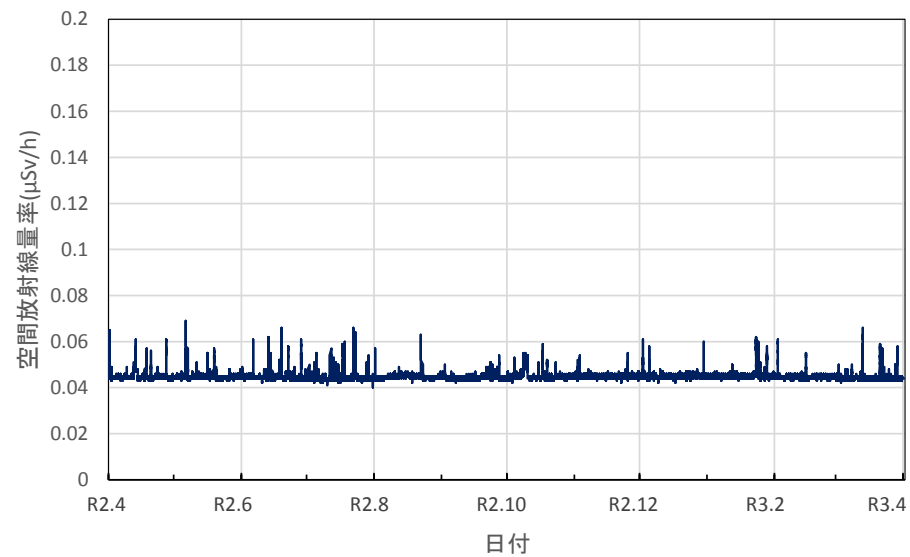
神奈川県横浜市 県立岸根高等学校の空間放射線量率(10分値使用)
