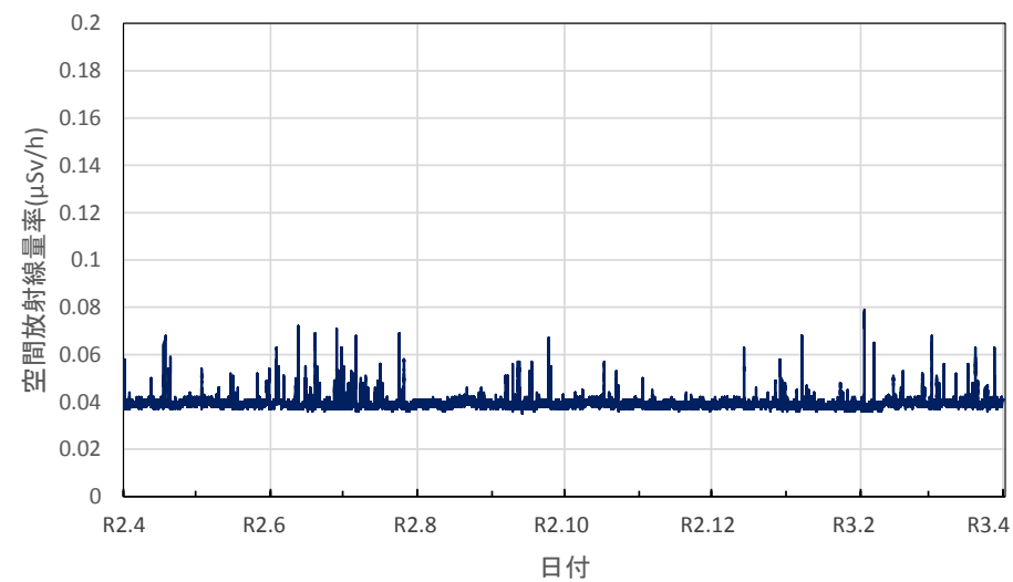
鹿児島県南さつま市 南薩地域振興局の空間放射線量率(10分値使用)
