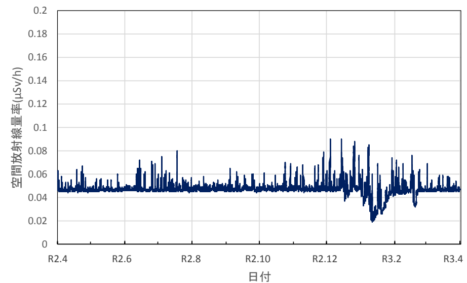
富山県射水市 県環境科学センターの空間放射線量率(10分値使用)
