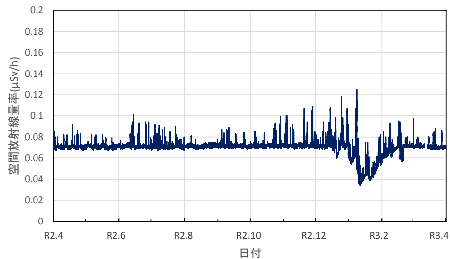
富山県小矢部市 砺波厚生センター小矢部支所の空間放射線量率(10分値使用)
