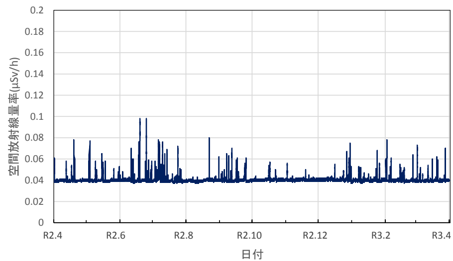
佐賀県嬉野市 県立塩田工業高等学校の空間放射線量率(10分値使用)
