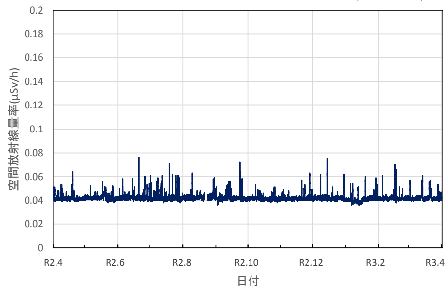
岩手県釜石市 釜石地区合同庁舎の空間放射線量率(10分値使用)
