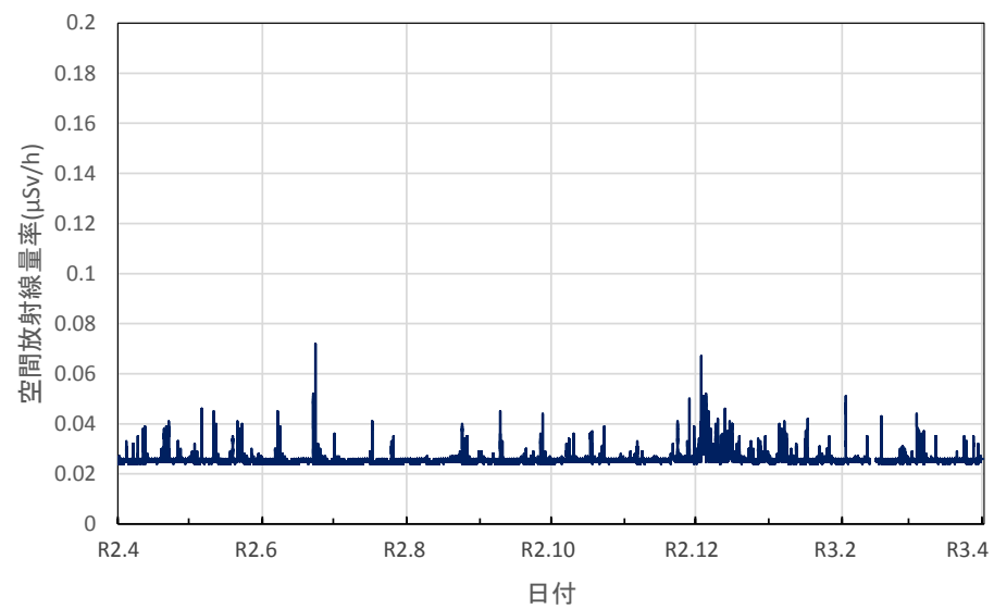
沖縄県名護市 北部福祉保健所の空間放射線量率(10分値使用)
