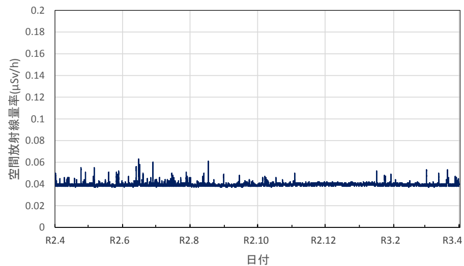
栃木県宇都宮市 県保健環境センターの空間放射線量率(10分値使用)
