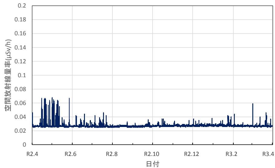
千葉県市原市 県環境研究センターの空間放射線量率(10分値使用)
