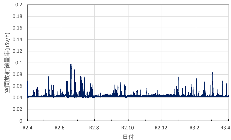
福岡県糸島市 糸島総合庁舎の空間放射線量率(10分値使用)
