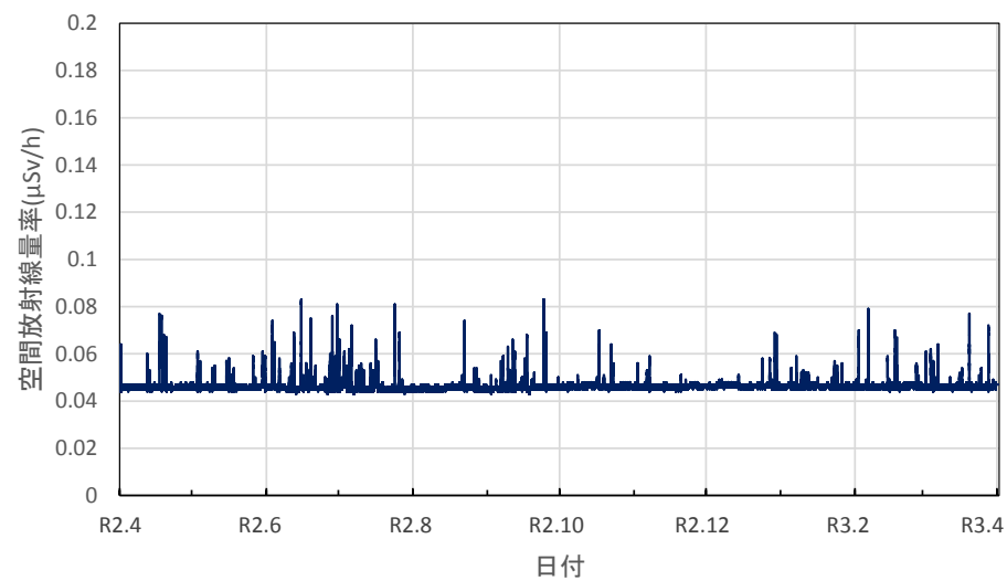
鹿児島県鹿児島市 県環境保健センターの空間放射線量率(10分値使用)
