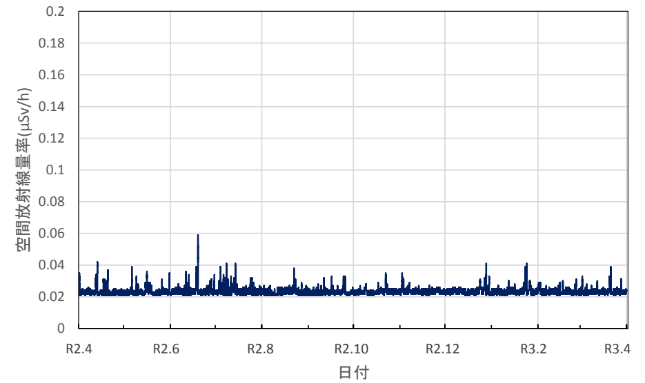
高知県高知市 県保健衛生総合庁舎の空間放射線量率(10分値使用)
