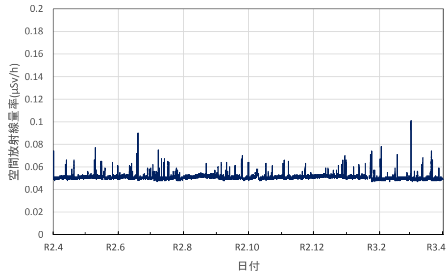
大阪府泉佐野市 市立佐野中学校の空間放射線量率(10分値使用)
