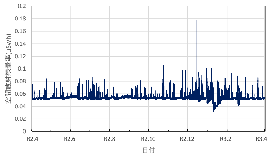
石川県小松市 さわ池ふれあいパークの空間放射線量率(10分値使用)
