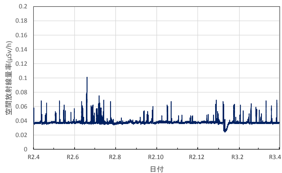
大分県国東市 国東高等学校の空間放射線量率(10分値使用)
