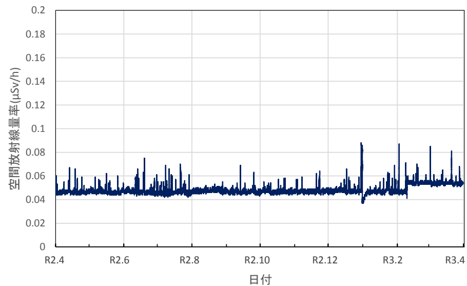
滋賀県東近江市 県東近江保健所の空間放射線量率(10分値使用)
