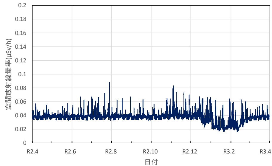
秋田県大仙市 仙北地域振興局の空間放射線量率(10分値使用)
