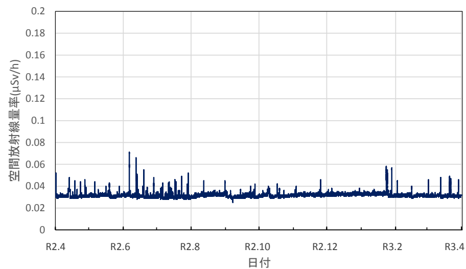
東京都八王子市 東京都立大学 南大沢キャンパスの空間放射線量率(10分値使用)
