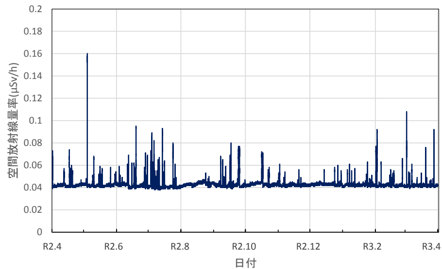
熊本県水俣市 県環境センターの空間放射線量率(10分値使用)
