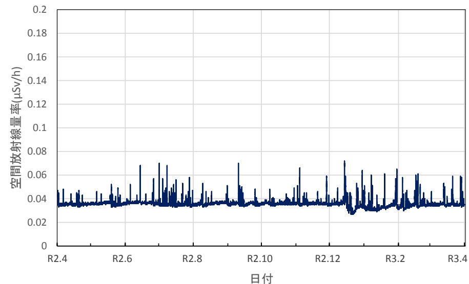
宮城県大崎市 大崎合同庁舎の空間放射線量率(10分値使用)
