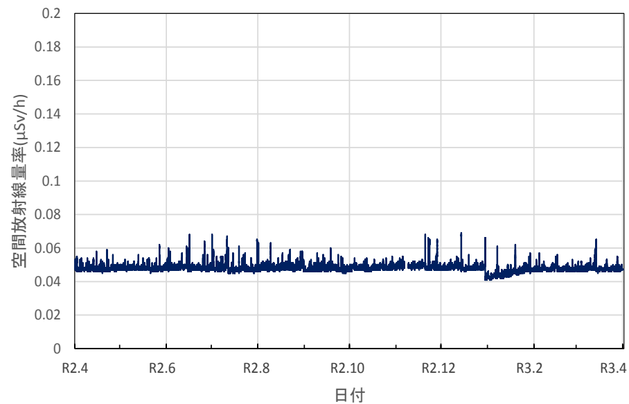
岩手県久慈市 久慈地区合同庁舎の空間放射線量率(10分値使用)
