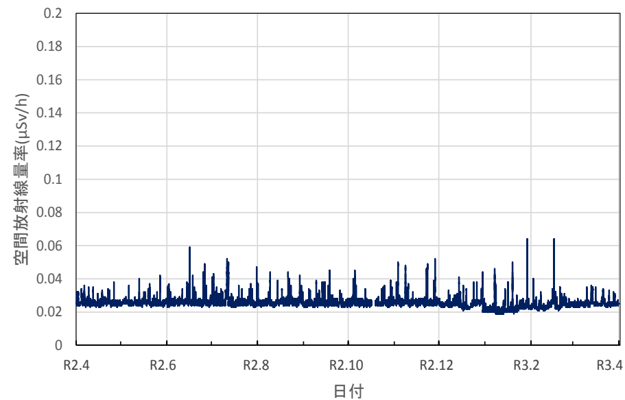
岩手県二戸市 二戸地区合同庁舎の空間放射線量率(10分値使用)
