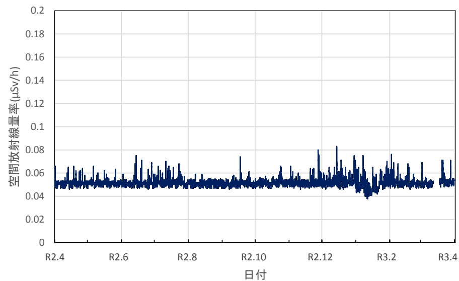
福井県越前市 越前市役所の空間放射線量率(10分値使用)
