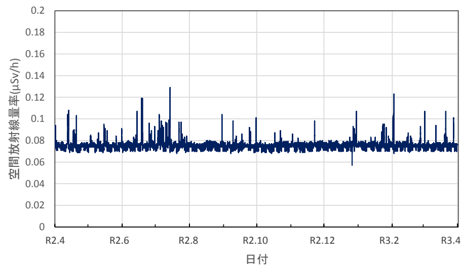
広島県東広島市 西部東厚生環境事務所の空間放射線量率(10分値使用)
