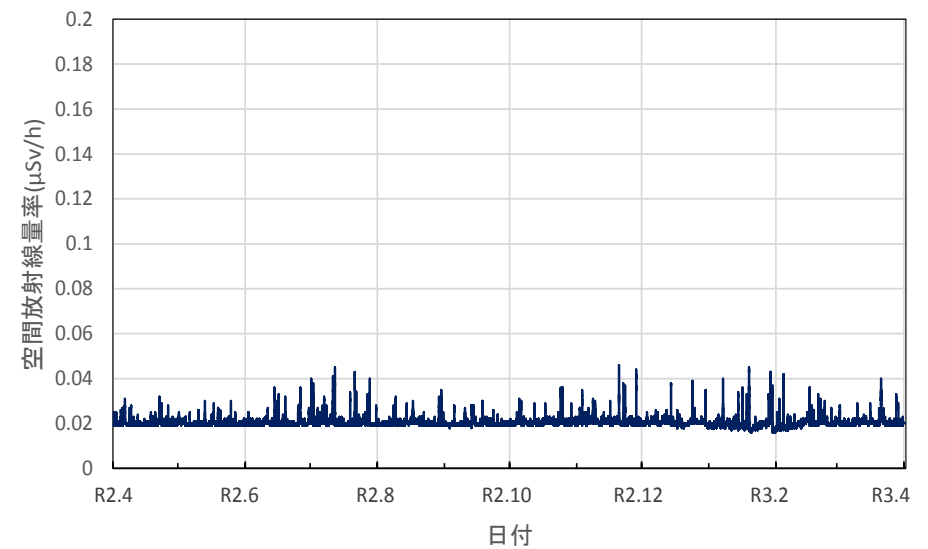
岩手県盛岡市 県環境保健研究センターの空間放射線量率(10分値使用)
