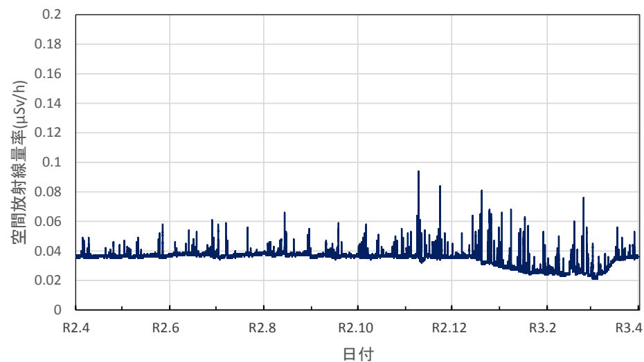
北海道札幌市 北海道原子力環境センター札幌分室の空間放射線量率(10分値使用)
