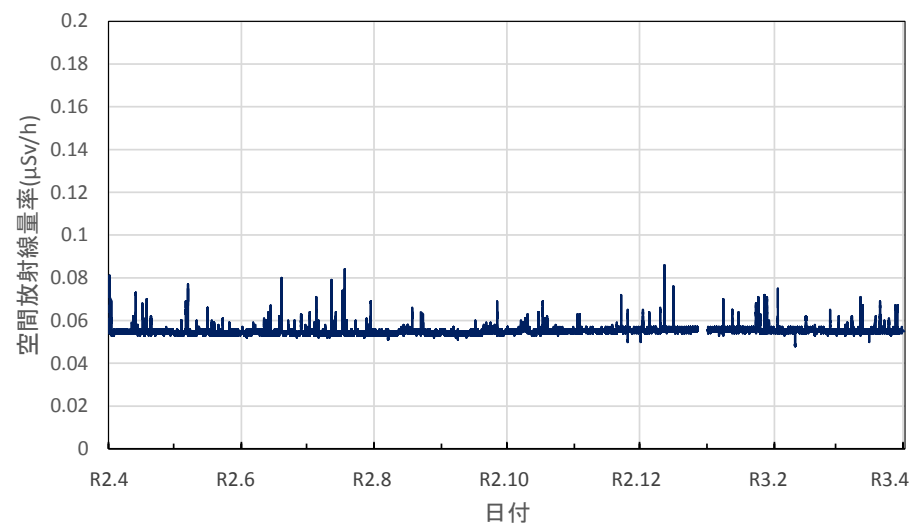
千葉県館山市 県安房農業普及センター跡地の空間放射線量率(10分値使用)
