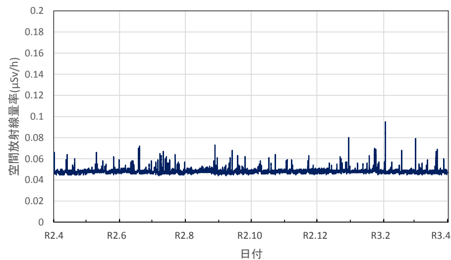
奈良県大和高田市 県高田土木事務所の空間放射線量率(10分値使用)
