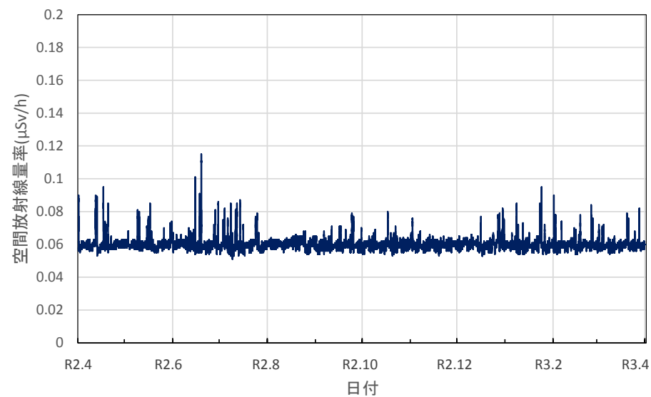
高知県四万十市 中村高等技術学校の空間放射線量率(10分値使用)
