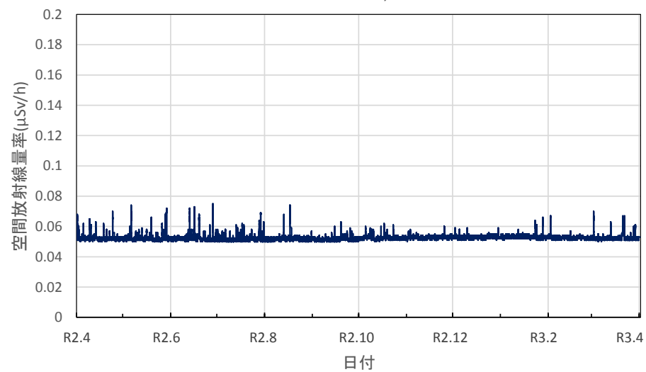
茨城県水戸市 旧県環境監視センター(石川局)の空間放射線量率(10分値使用)
