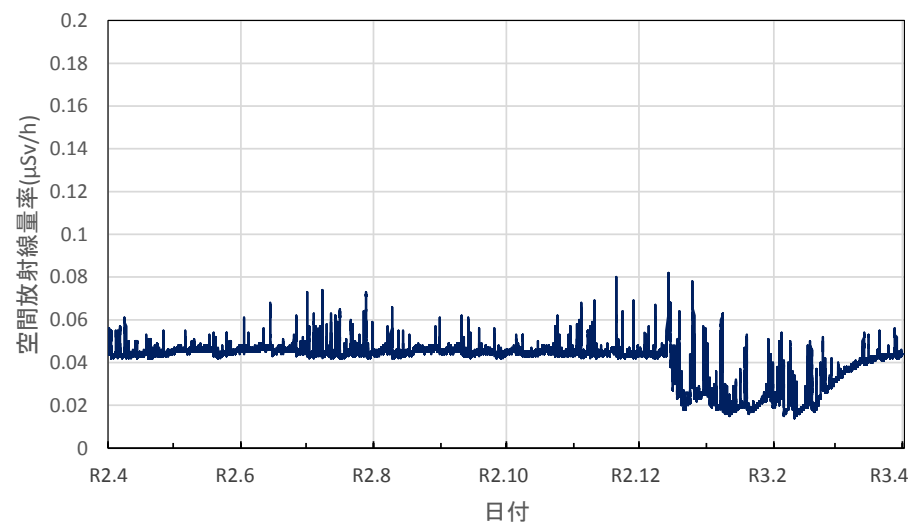
山形県村山市 県環境科学研究所の空間放射線量率(10分値使用)
