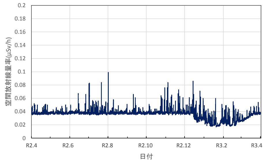
山形県新庄市 最上総合支庁の空間放射線量率(10分値使用)
