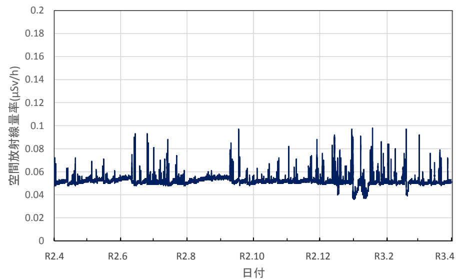
鳥取県大山町 大山町役場大山支所の空間放射線量率(10分値使用)
