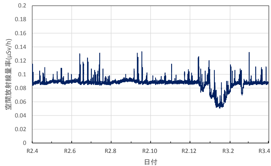
島根県奥出雲町 県仁多土木事業所の空間放射線量率(10分値使用)
