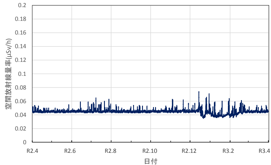
山形県山形市 県衛生研究所の空間放射線量率(10分値使用)
