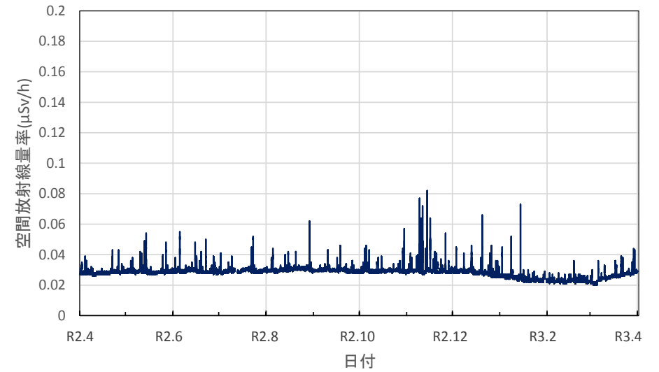
北海道網走市 オホーツク総合振興局の空間放射線量率(10分値使用)
