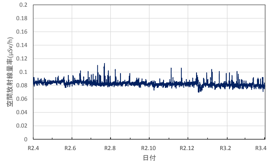
福島県伊達市 霊山総合支所の空間放射線量率(10分値使用)
