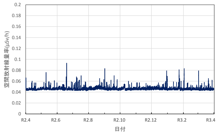
和歌山県橋本市 伊都総合庁舎の空間放射線量率(10分値使用)
