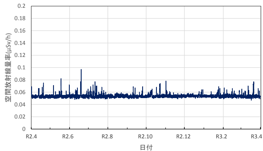
徳島県美波町 南部総合県民局美波庁舎の空間放射線量率(10分値使用)
