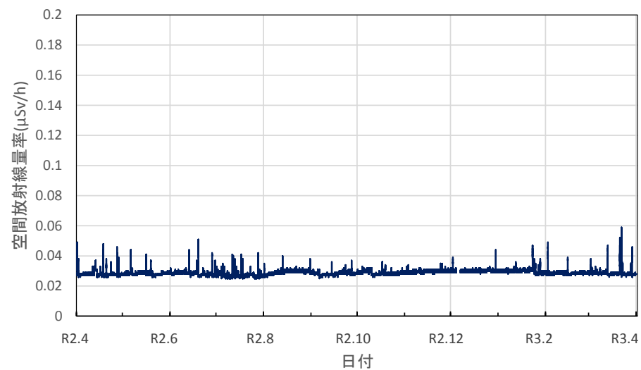
神奈川県海老名市 (地独) 県立産業技術総合研究所の空間放射線量率(10分値使用)
