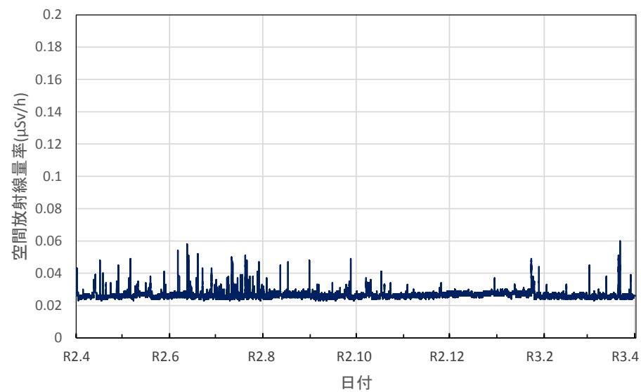
山梨県上野原市 上野原市役所の空間放射線量率(10分値使用)
