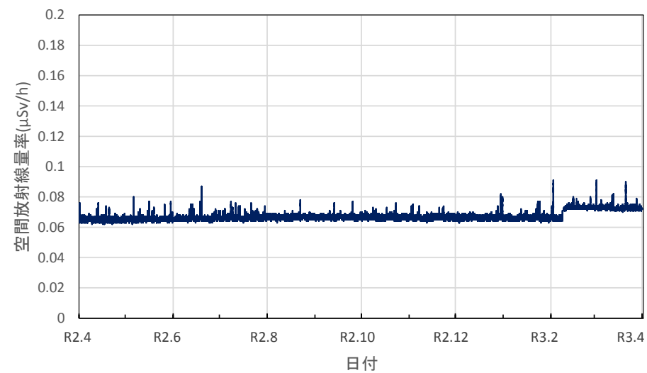
滋賀県草津市 県草津保健所(南部合同庁舎)の空間放射線量率(10分値使用)
