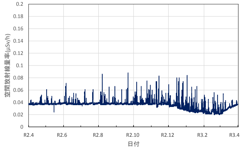
北海道稚内市 宗谷総合振興局の空間放射線量率(10分値使用)
