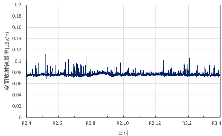
愛知県名古屋市 環境調査センターの空間放射線量率(10分値使用)
