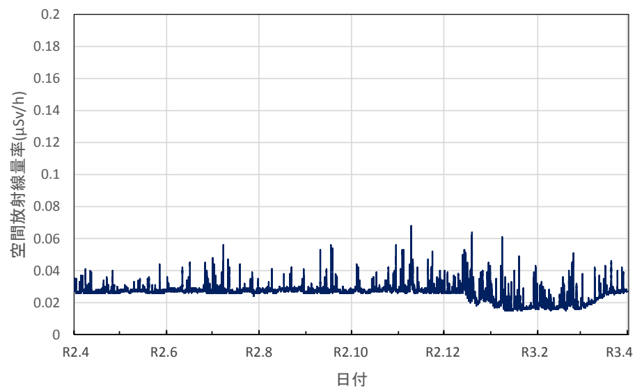
青森県青森市 県環境保健センターの空間放射線量率(10分値使用)
