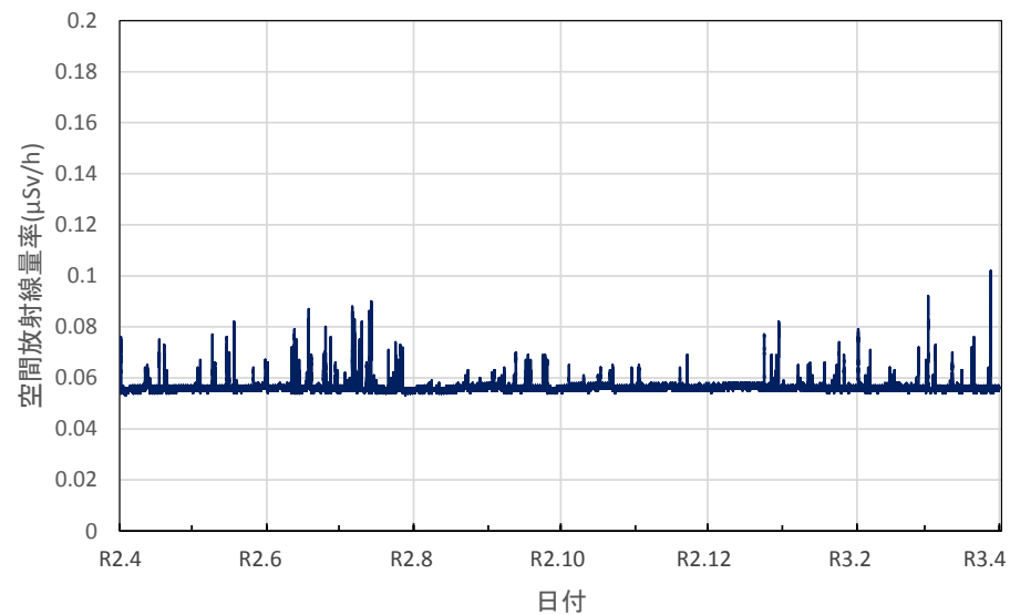
長崎県壱岐市 県壱岐保健所の空間放射線量率(10分値使用)
