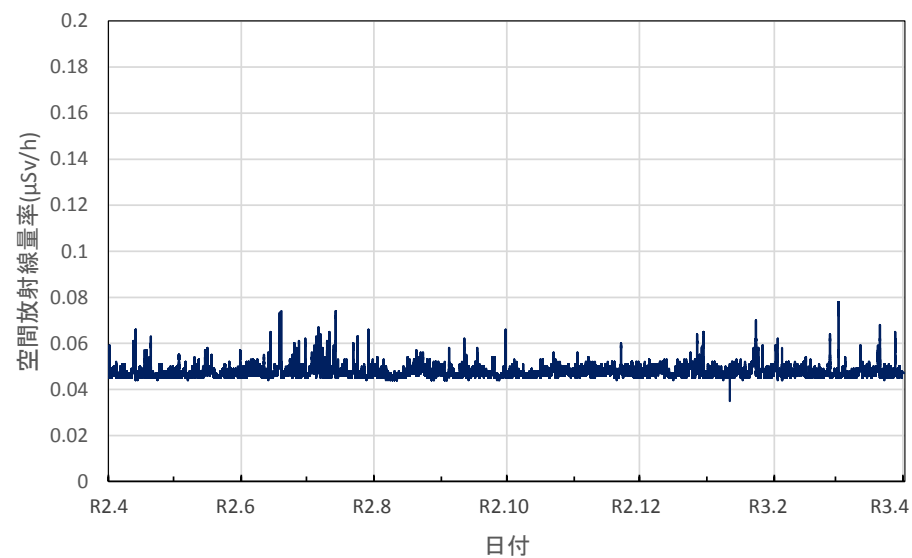
広島県広島市 県健康福祉センターの空間放射線量率(10分値使用)
