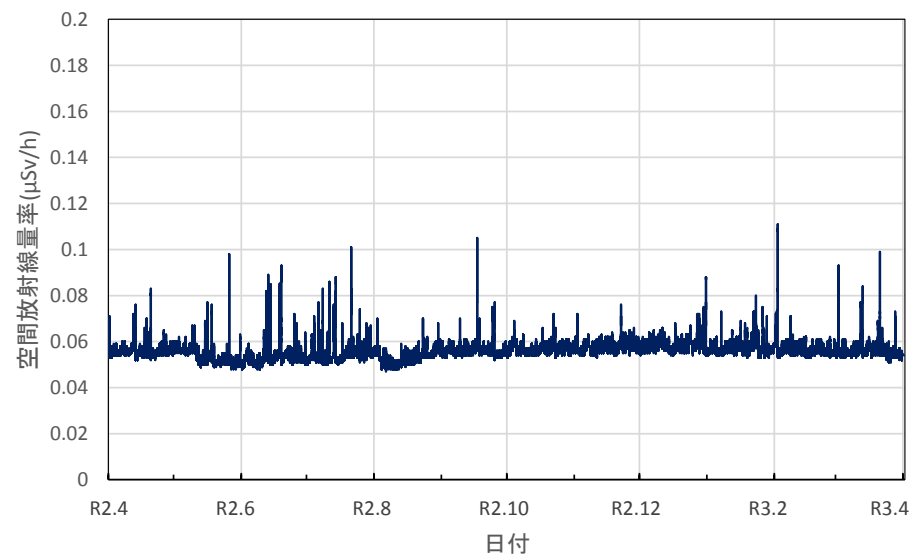
岡山県津山市 県食肉衛生検査所の空間放射線量率(10分値使用)
