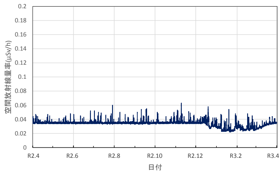
青森県弘前市 弘前市役所の空間放射線量率(10分値使用)
