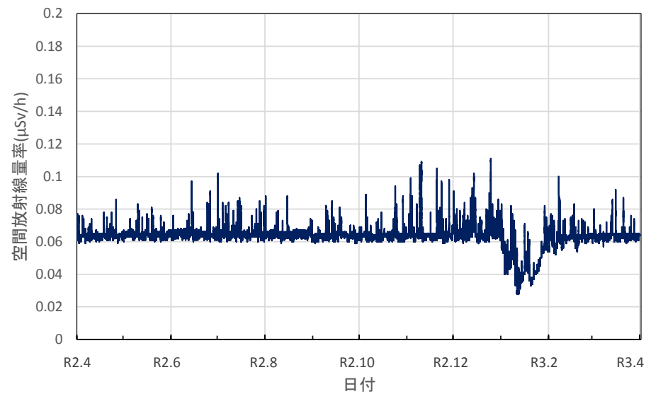
新潟県新発田市 新発田地域振興局の空間放射線量率(10分値使用)
