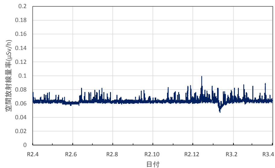
福井県あわら市 あわら市役所の空間放射線量率(10分値使用)
