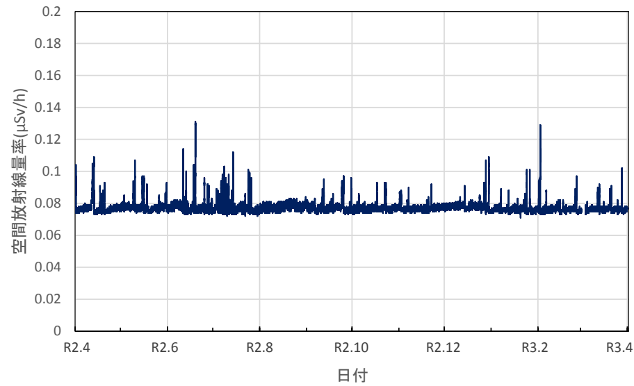
愛媛県松山市 県産業技術研究所の空間放射線量率(10分値使用)
