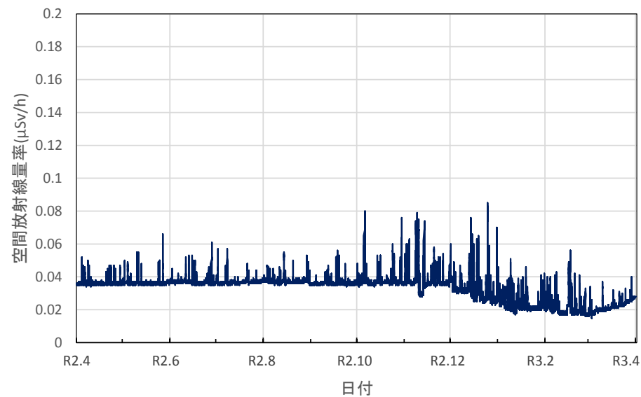
北海道倶知安町 後志総合振興局の空間放射線量率(10分値使用)
