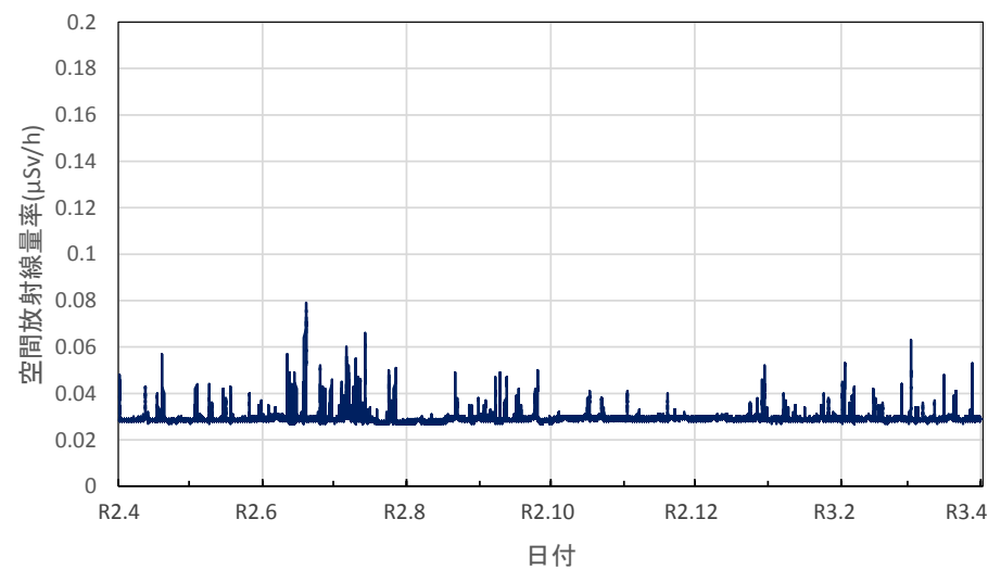
長崎県大村市 県環境保健研究センターの空間放射線量率(10分値使用)
