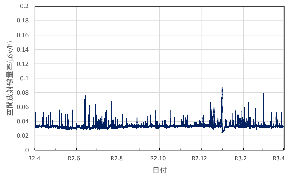
滋賀県高島市 南部消防署の空間放射線量率(10分値使用)
