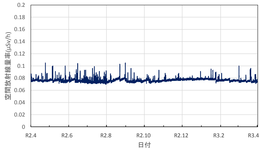
栃木県那須塩原市 那須塩原市役所本庁舎の空間放射線量率(10分値使用)
