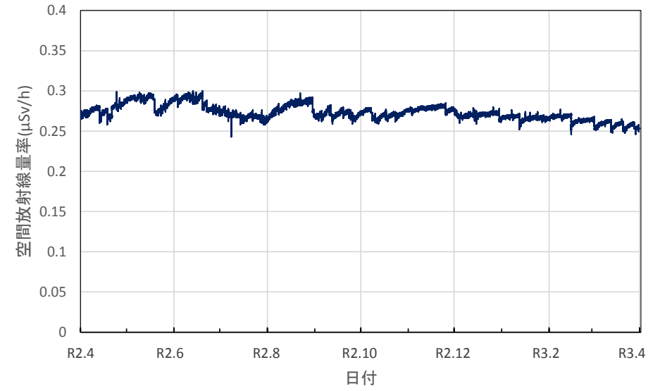
福島県大熊町 大野の空間放射線量率(10分値使用)
