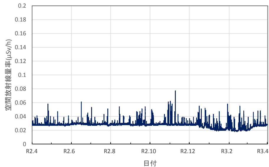
北海道函館市 渡島総合振興局の空間放射線量率(10分値使用)
