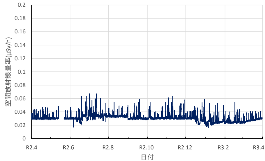
秋田県鹿角市 鹿角地域振興局の空間放射線量率(10分値使用)
