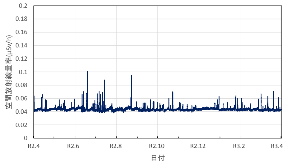
高知県安芸市 安芸広域公園里のゾーンの空間放射線量率(10分値使用)
