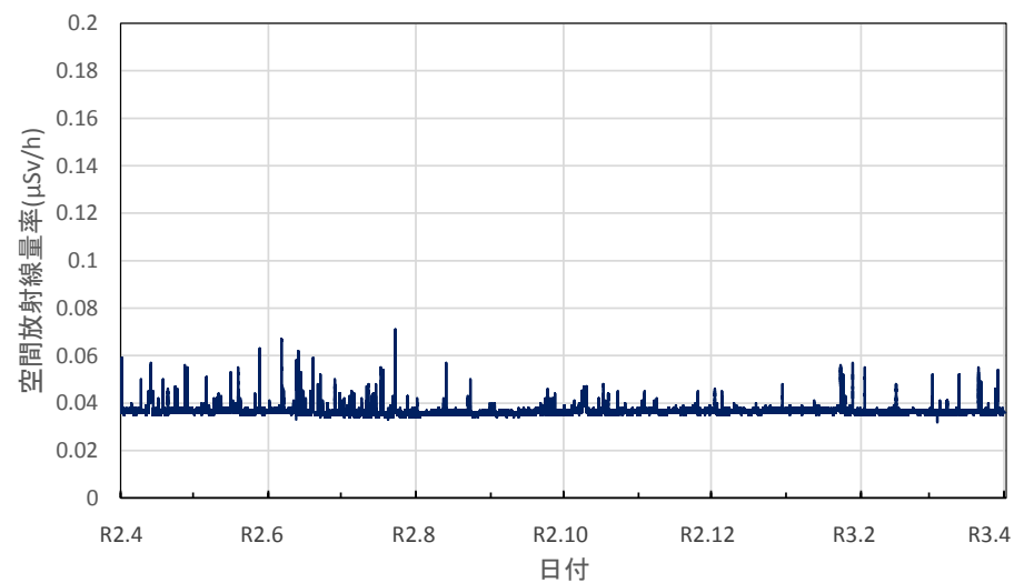
東京都新宿区 都健康安全研究センターの空間放射線量率(10分値使用)
