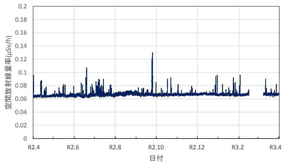
愛媛県今治市 県立今治東中等教育学校の空間放射線量率(10分値使用)
