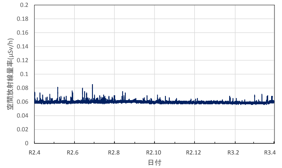
茨城県筑西市 筑西市役所の空間放射線量率(10分値使用)
