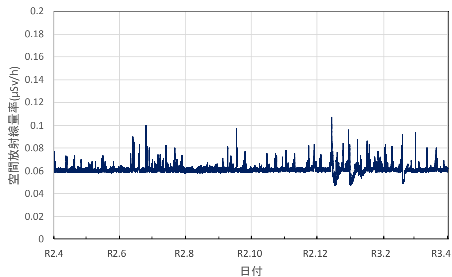
鳥取県湯梨浜町 県衛生環境研究所の空間放射線量率(10分値使用)
