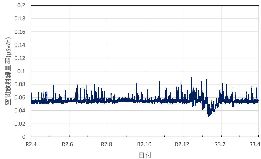
福井県鯖江市 鯖江市役所の空間放射線量率(10分値使用)
