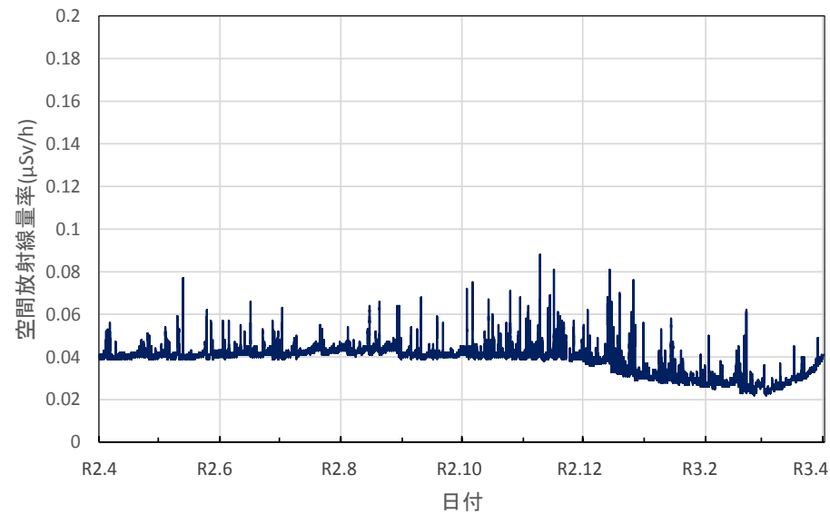
北海道旭川市 上川総合振興局の空間放射線量率(10分値使用)
