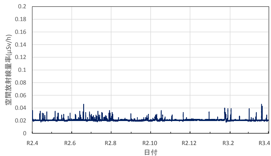
山梨県富士吉田市 富士吉田合同庁舎の空間放射線量率(10分値使用)
