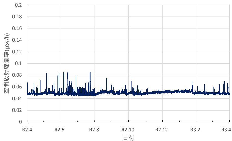
群馬県太田市 ぐんまこどもの国の空間放射線量率(10分値使用)
