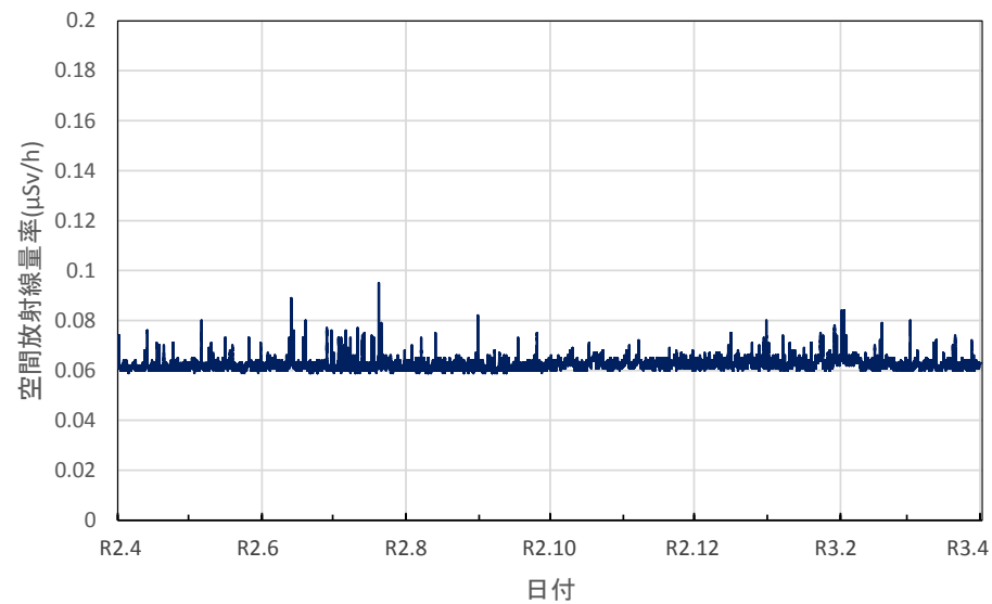
岐阜県各務原市 保健環境研究所の空間放射線量率(10分値使用)
