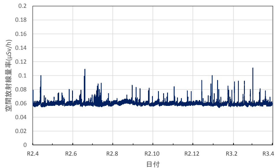
徳島県三好市 池田総合体育館の空間放射線量率(10分値使用)
