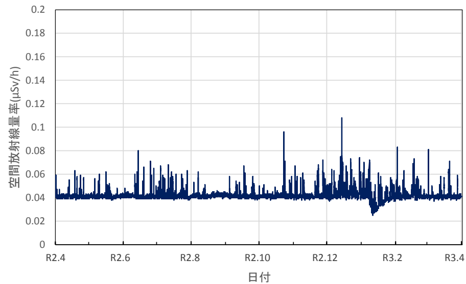
福井県坂井市 坂井市役所三国支所の空間放射線量率(10分値使用)
