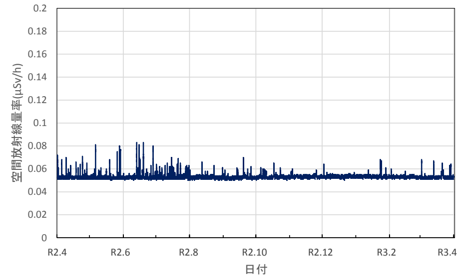
栃木県真岡市 県東環境森林事務所の空間放射線量率(10分値使用)
