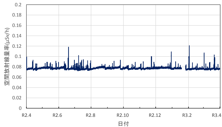
大阪府東大阪市 環境衛生検査センターの空間放射線量率(10分値使用)
