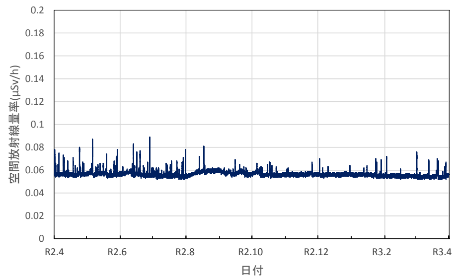
茨城県水戸市 茨城県庁の空間放射線量率(10分値使用)
