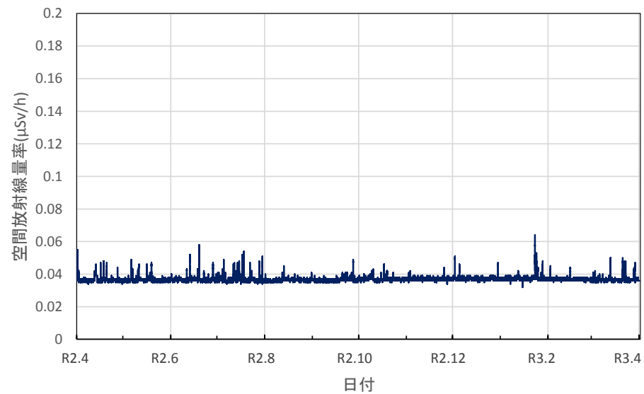
神奈川県茅ヶ崎市 衛生研究所の空間放射線量率(10分値使用)
