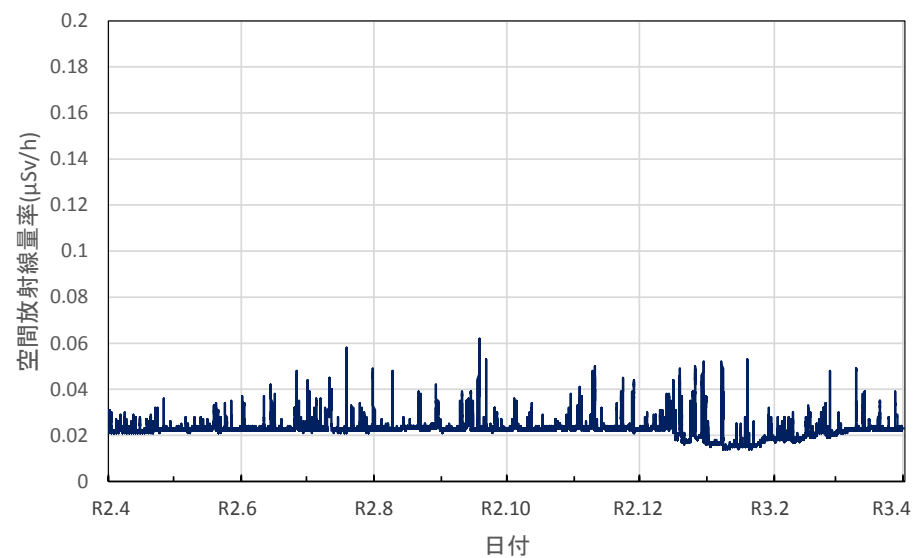
青森県十和田市 十和田市役所の空間放射線量率(10分値使用)
