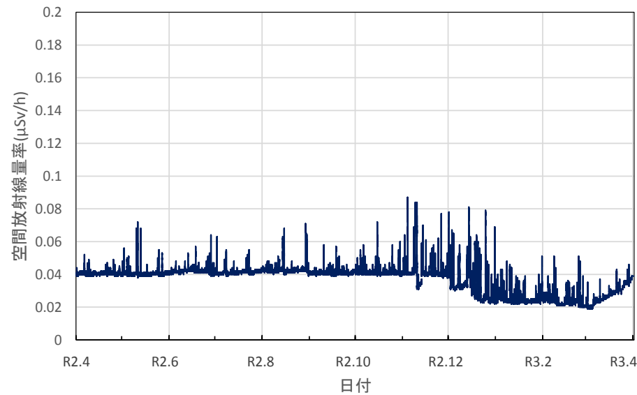
北海道岩見沢市 空知総合振興局の空間放射線量率(10分値使用)
