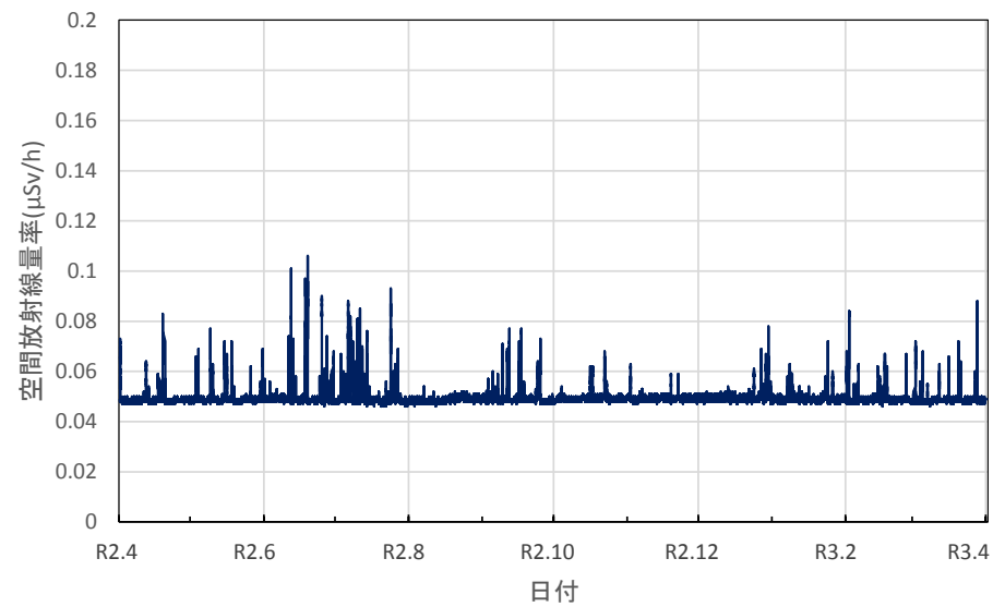
佐賀県佐賀市 県環境センターの空間放射線量率(10分値使用)
