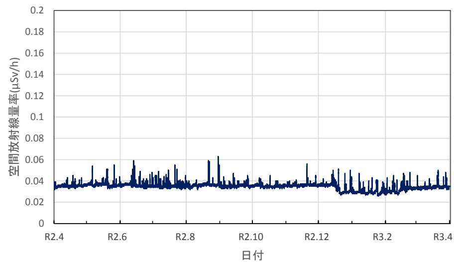
群馬県草津町 総合保健福祉センターの空間放射線量率(10分値使用)
