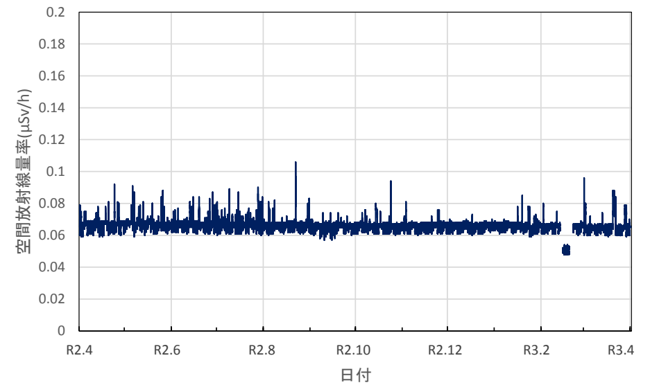
栃木県那須町 那須町役場の空間放射線量率(10分値使用)
