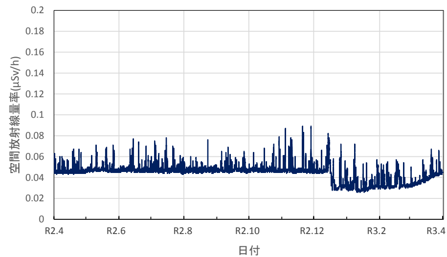
新潟県南魚沼市 南魚沼地域振興局健康福祉環境部の空間放射線量率(10分値使用)
