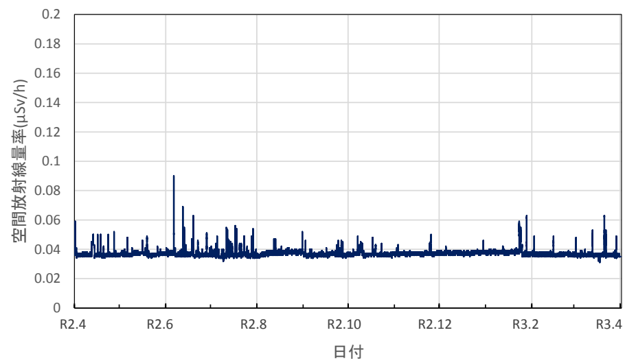
神奈川県相模原市 相模川発電管理事務所の空間放射線量率(10分 値使用)
