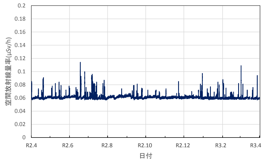
福岡県北九州市 八幡総合庁舎の空間放射線量率(10分値使用)
