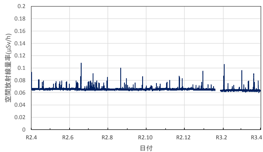
大阪府大阪市 大阪健康安全基盤研究所の空間放射線量率(10分値使用)
