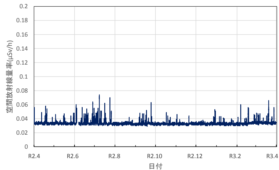
鹿児島県鹿屋市 大隅地域振興局の空間放射線量率(10分値使用)
