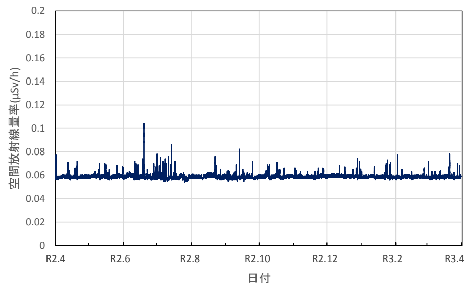
和歌山県田辺市 西牟婁総合庁舎の空間放射線量率(10分値使用)
