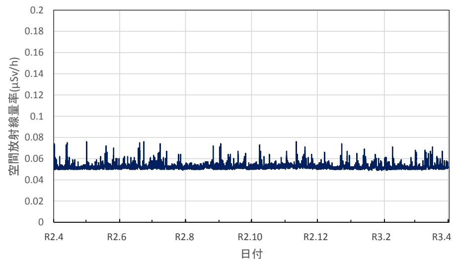
香川県高松市 県環境保健研究センターの空間放射線量率(10分値使用)
