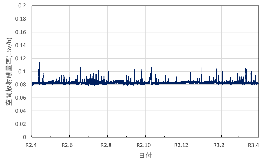
三重県尾鷲市 広域防災拠点施設の空間放射線量率(10分値使用)
