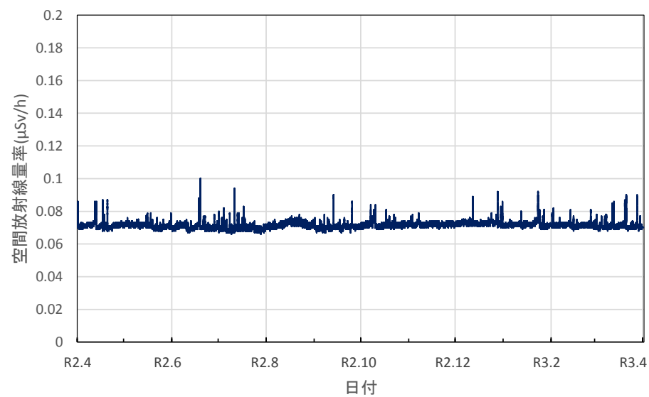
和歌山県新宮市 東牟婁総合庁舎の空間放射線量率(10分値使用)
