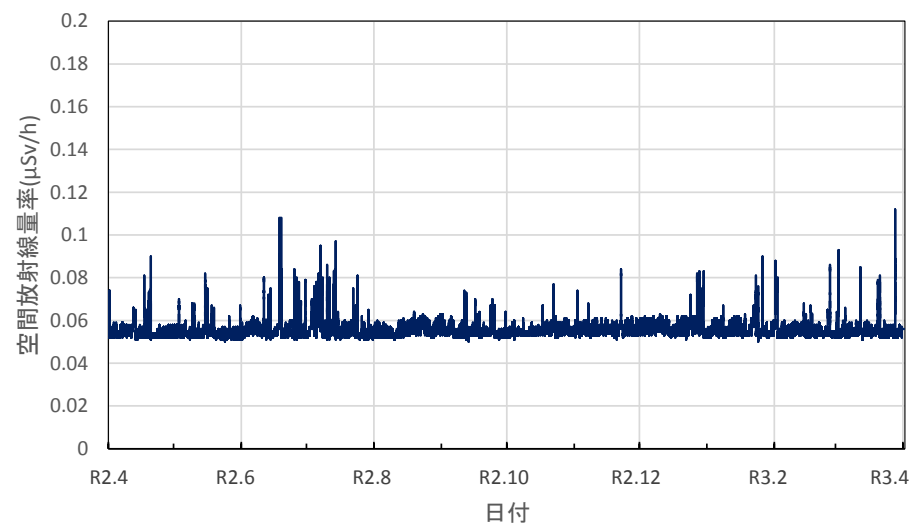
山口県岩国市 岩国健康福祉センターの空間放射線量率(10分値使用)
