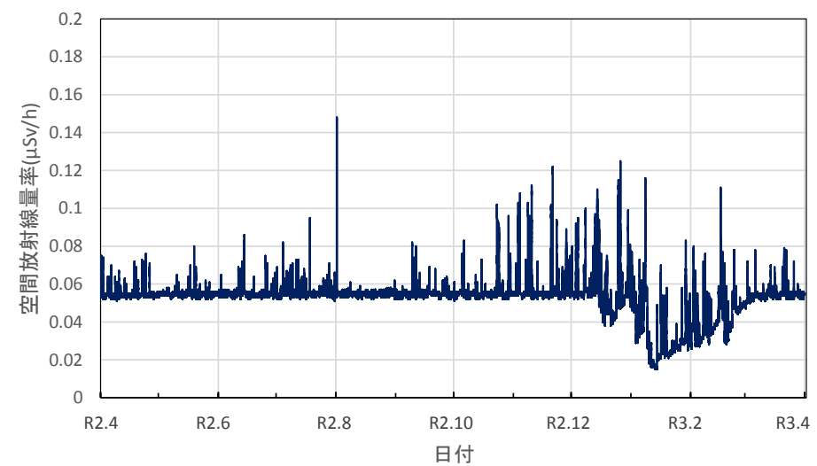
新潟県上越市 上越地域振興局健康福祉環境部の空間放射線量率(10分値使用)
