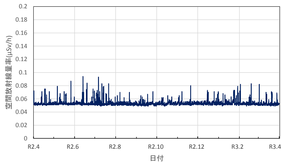
愛知県一宮市 木曽川消防署大気測定局の空間放射線量率(10分値 使用)
