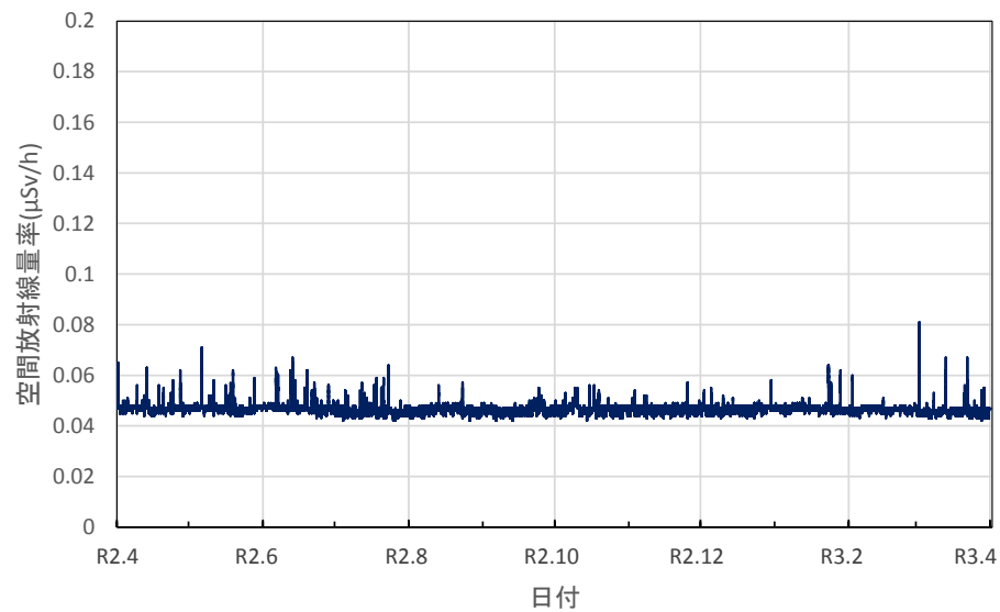
千葉県市川市 市立大柏小学校の空間放射線量率(10分値使用)
