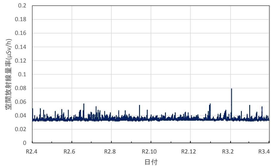
滋賀県大津市 県衛生科学センターの空間放射線量率(10分値使用)
