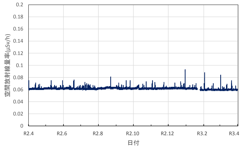
大阪府富田林市 富田林保健所の空間放射線量率(10分値使用)
