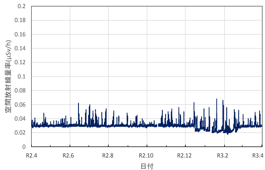
岩手県花巻市 花巻地区合同庁舎の空間放射線量率(10分値使用)
