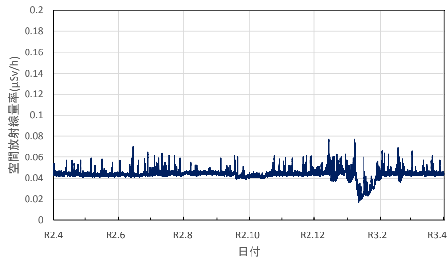
福井県福井市 原子力環境監視センター福井分析管理室の空間放射線量率(10分値使用)
