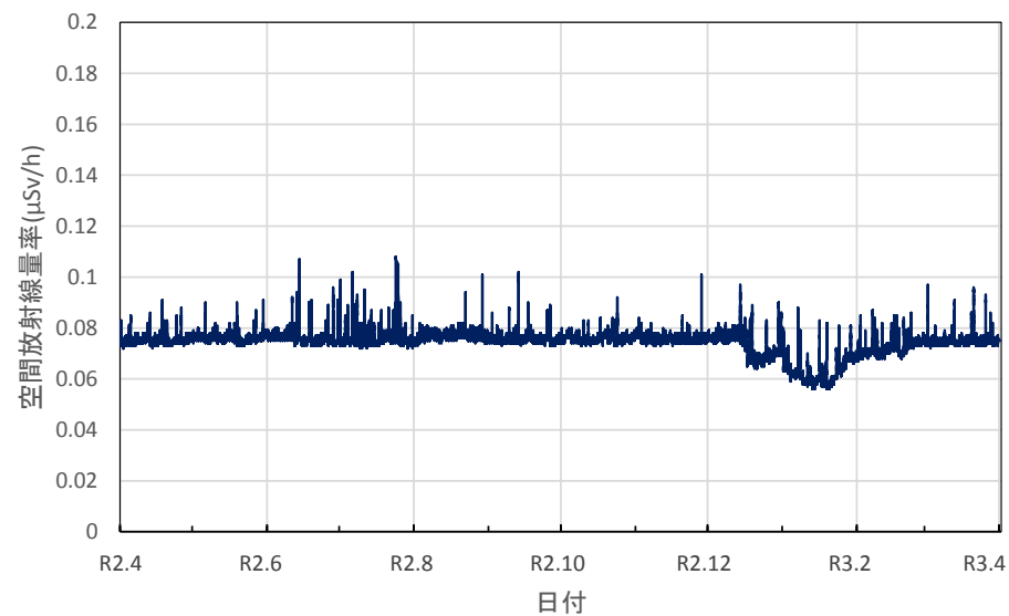
長野県大町市 大町合同庁舎の空間放射線量率(10分値使用)
