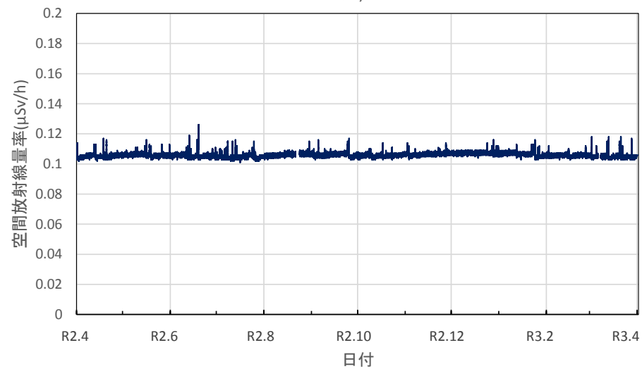
兵庫県神戸市 県立工業技術センターの空間放射線量率(10分値使用)
