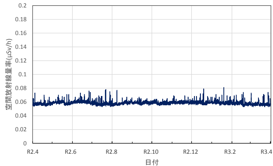
福島県田村市 船引公民館の空間放射線量率(10分値使用)
