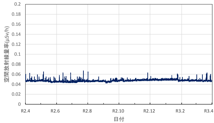
埼玉県加須市 県環境科学国際センターの空間放射線量率(10分値使用)
