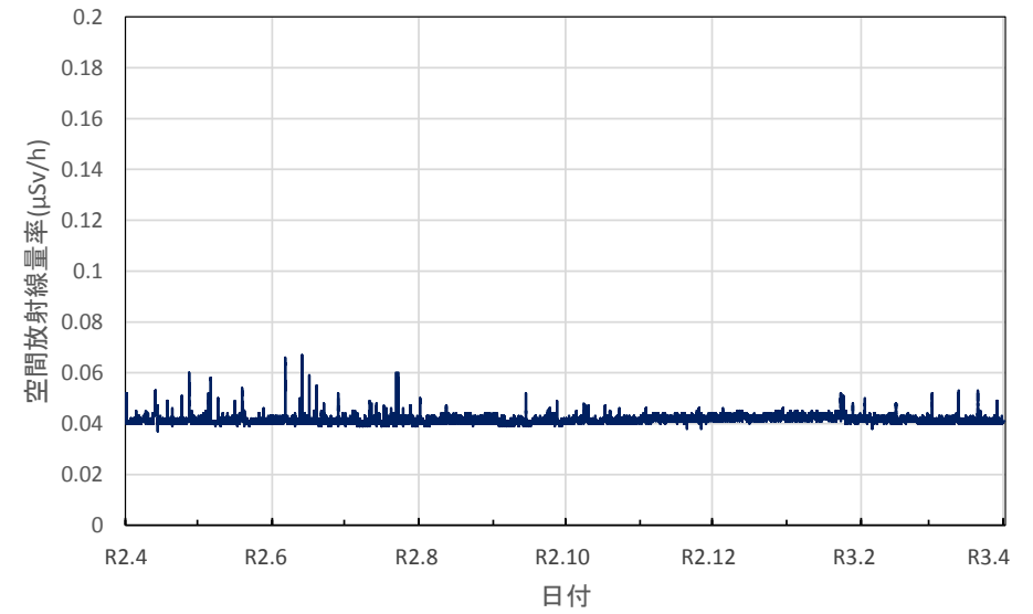
埼玉県狭山市 狭山保健所の空間放射線量率(10分値使用)
