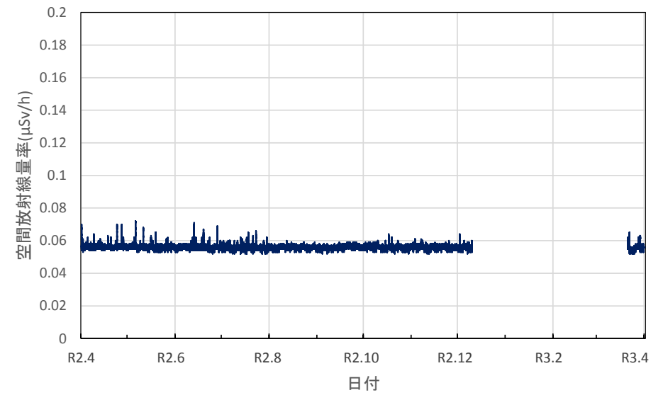
茨城県土浦市 土浦市役所大町庁舎の空間放射線量率(10分値使用)
