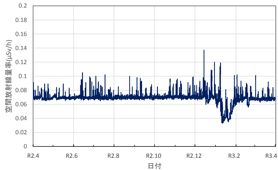
富山県高岡市 高岡厚生センターの空間放射線量率(10分値使用)
