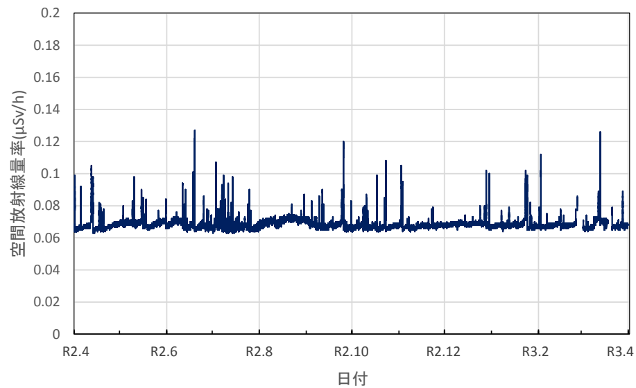
愛媛県新居浜市 県総合科学博物館の空間放射線量率(10分値使用)
