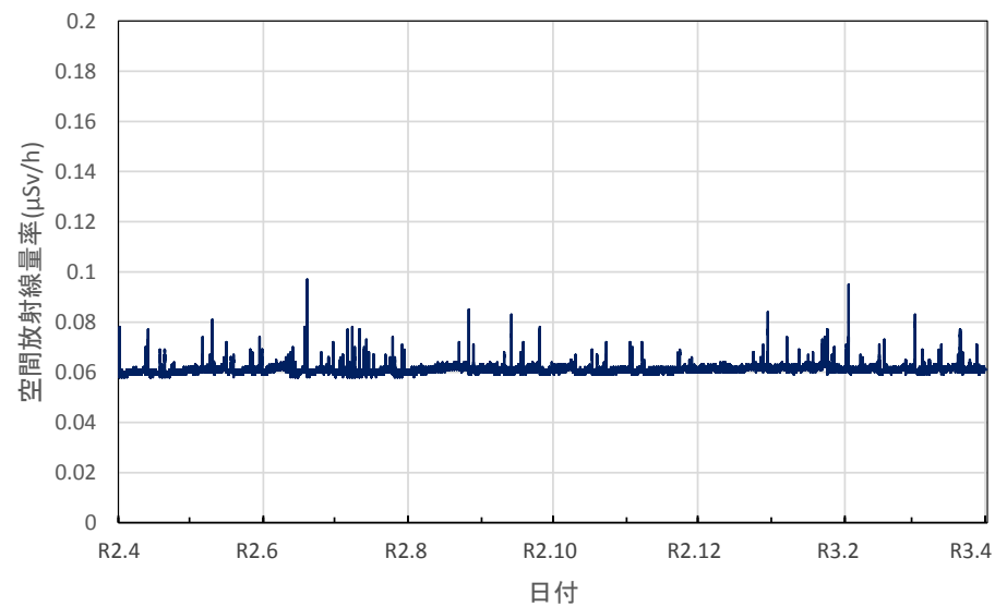
奈良県奈良市 奈良土木事務所の空間放射線量率(10分値使用)
