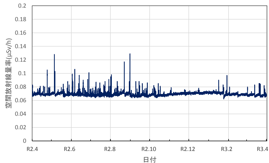
栃木県日光市 県西環境森林事務所の空間放射線量率(10分値使用)
