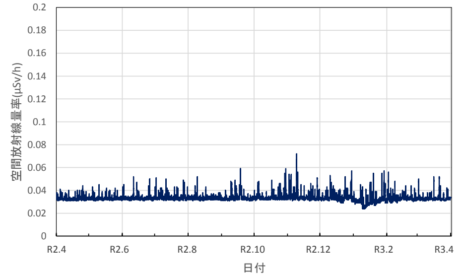
秋田県秋田市 県健康環境センターの空間放射線量率(10分値使用)
