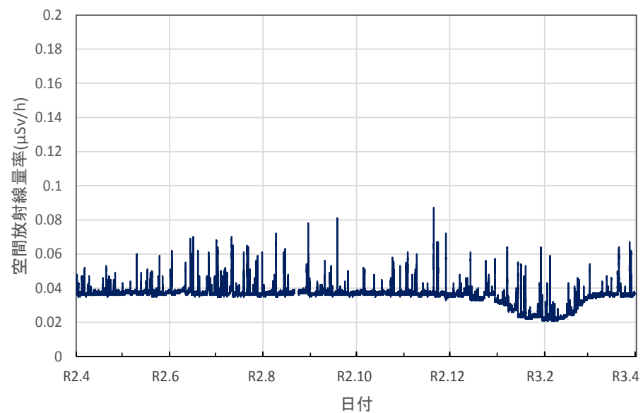
岩手県滝沢市 岩手県立大学の空間放射線量率(10分値使用)
