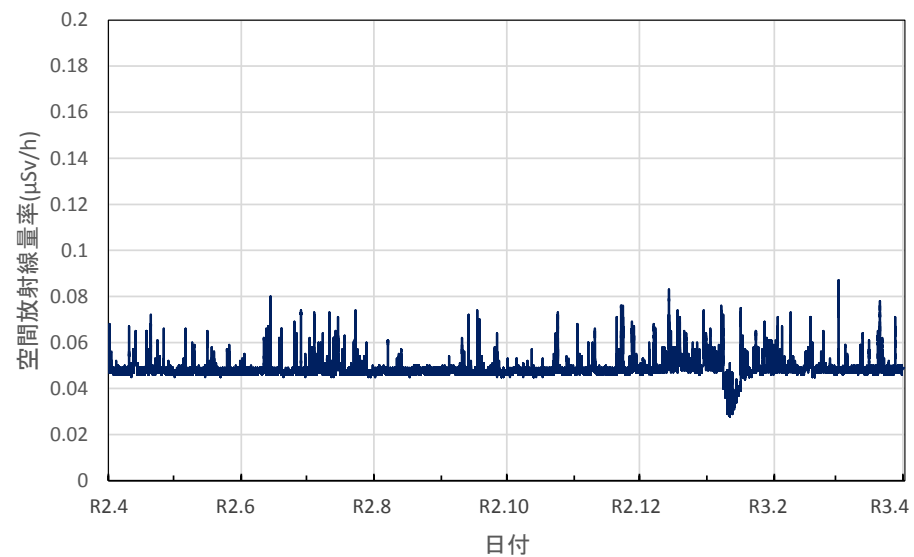
福井県福井市 越廼ふるさと資料館の空間放射線量率(10分値使用)
