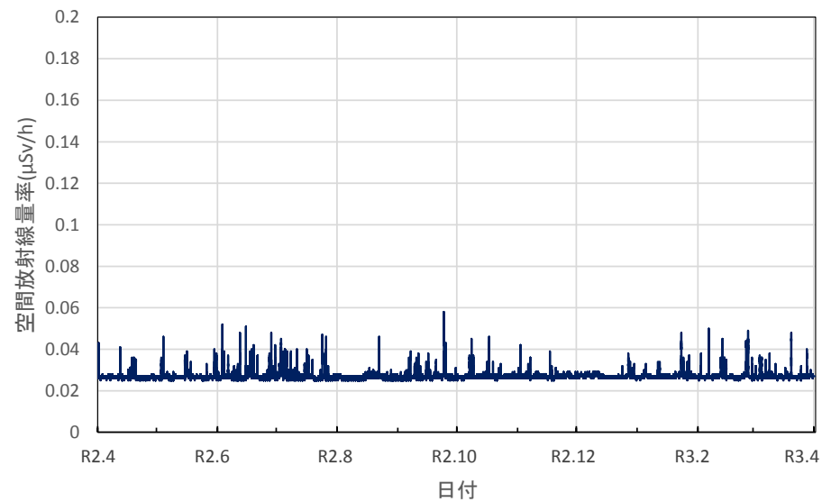
宮崎県宮崎市 県衛生環境研究所の空間放射線量率(10分値使用)
