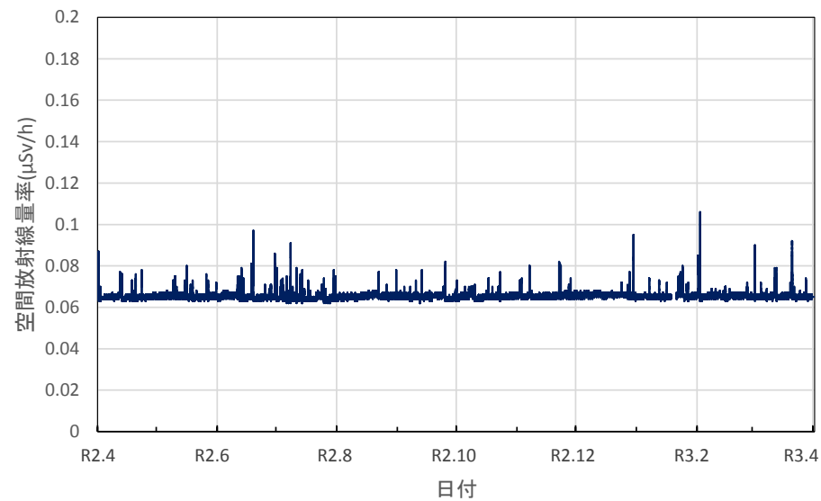
大阪府寝屋川市 寝屋川保健所の空間放射線量率(10分値使用)
