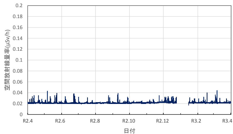
沖縄県うるま市 原子力艦放射能調査施設の空間放射線量率(10分値使用)
