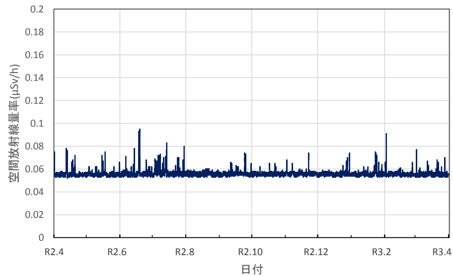
広島県尾道市 東部厚生環境事務所の空間放射線量率(10分値使用)
