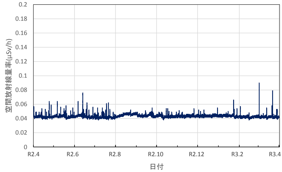
茨城県龍ヶ崎市 龍ヶ崎市役所の空間放射線量率(10分値使用)
