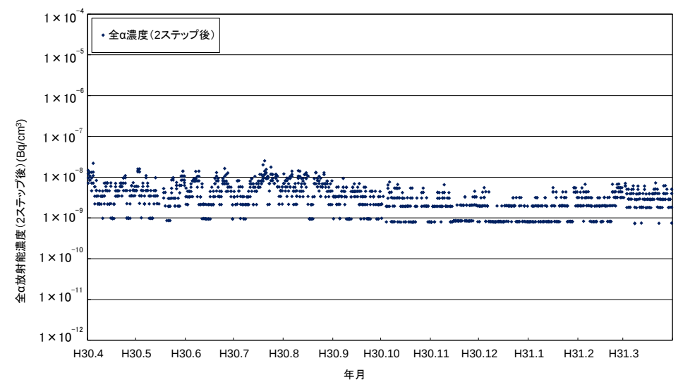
佐渡関岬測定所における大気浮遊じんの全 \alpha 放射能濃度(2ステップ後)の経時変化
