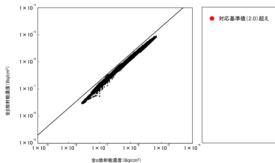
利尻測定所における全α及び全β放射能濃度分布 (集じん開始後40分以上の測定データを採用)
