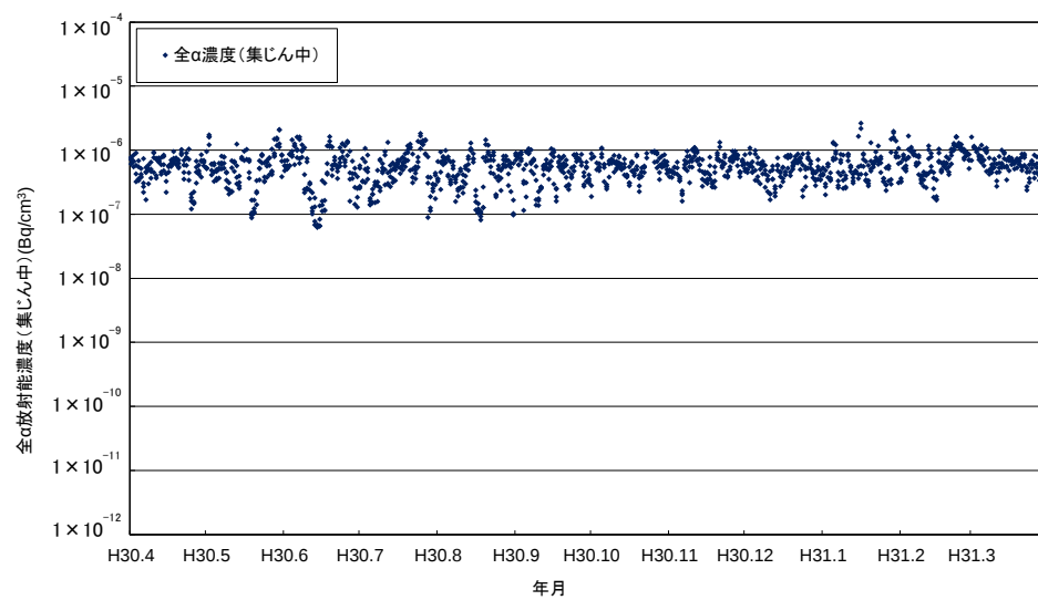
佐渡関岬測定所における大気浮遊じんの全 \alpha 放射能濃度(集じん中)の経時変化
