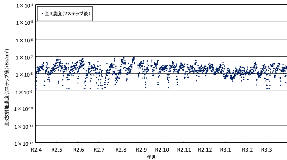
構原測定所における大気浮遊じんの全β放射能濃度(2ステップ後)の経時変化
