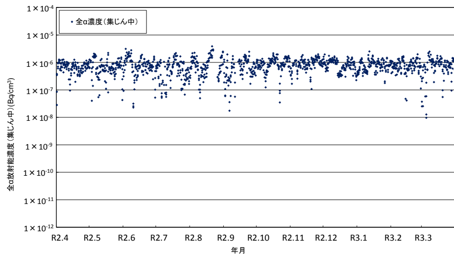
橿原測定所における大気浮遊じんの全α放射能濃度(集じん中)の経時変化
