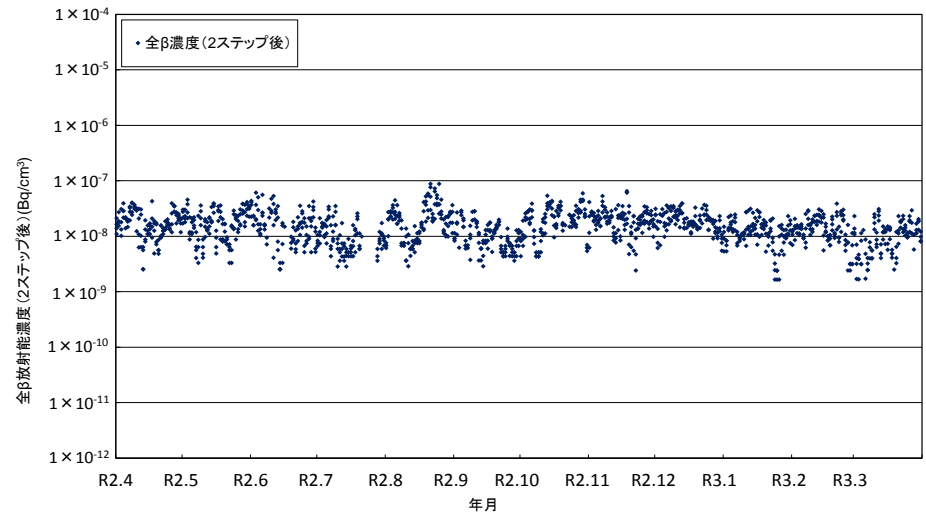
対馬測定所における大気浮遊じん全β放射能濃度(2ステップ後)の経時変化
