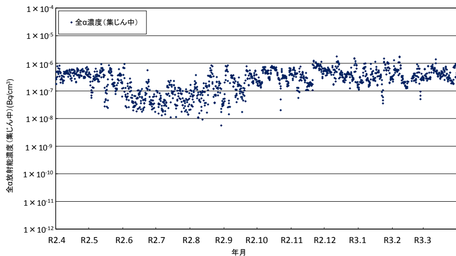
辺戸岬測定所における大気浮遊じんの全α放射能濃度(集じん中)の経時変化
