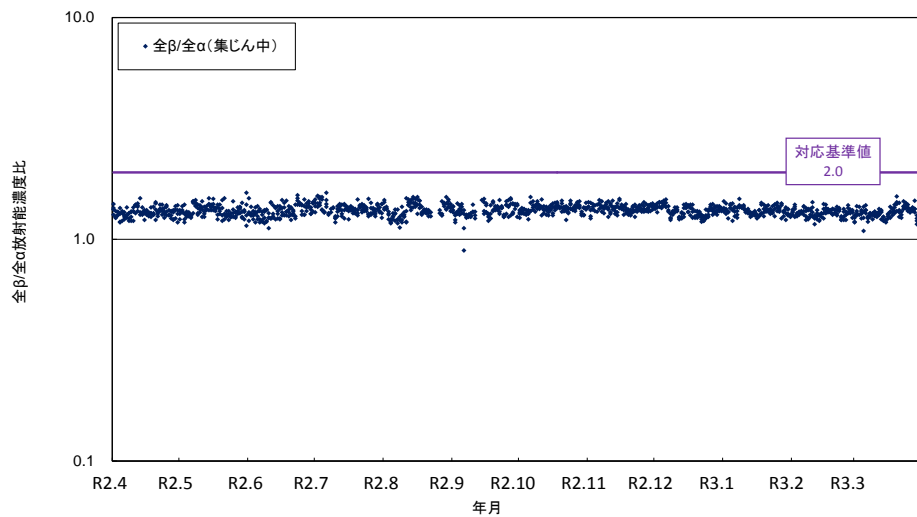
構原測定所における大気浮遊じんの全β/全α放射能濃度比(集じん中)の経時変化
