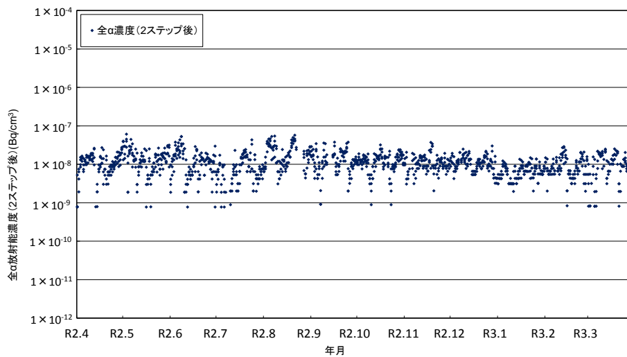
橿原測定所における大気浮遊じんの全α放射能濃度(2ステップ後)の経時変化
