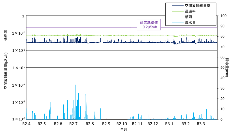
橿原測定所における空間放射線量率及び降水量との関係
