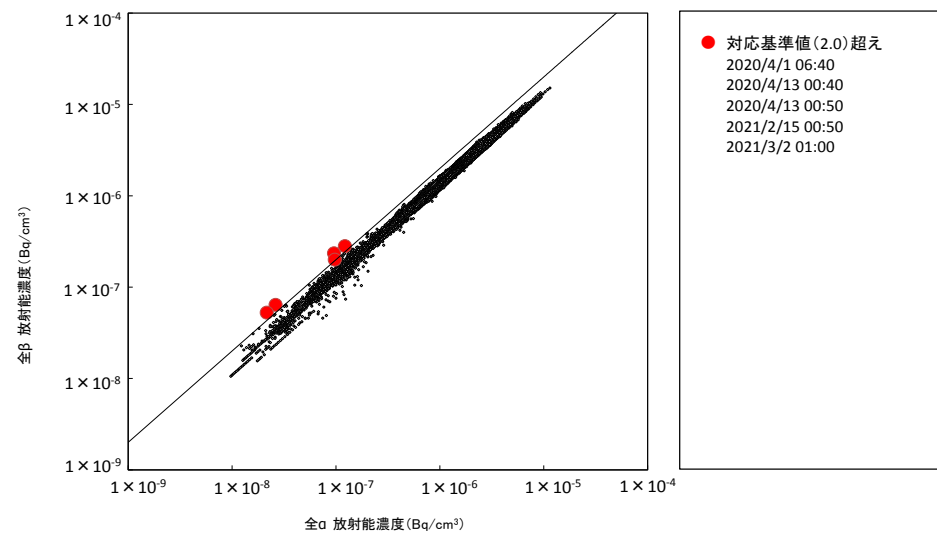
構原測定所における全α及び全β放射能濃度分布 (集じん開始後40分以上の測定データを採用)
