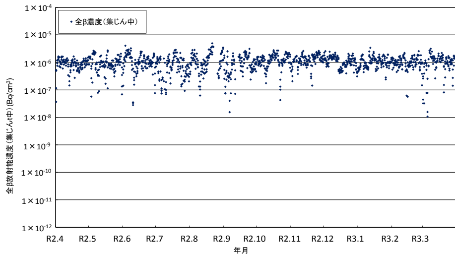
構原測定所における大気浮遊じんの全β放射能濃度(集じん中)の経時変化
