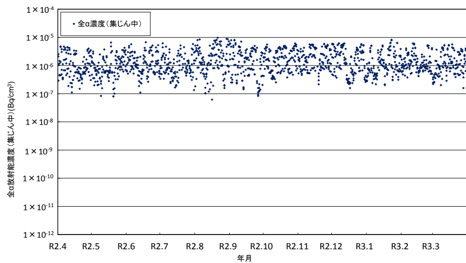
蟠竜湖測定所における大気浮遊じんの全α放射能濃度(集じん中)の経時変化
