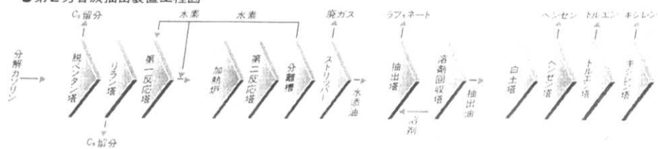
●第2芳香族抽出装置工程図
