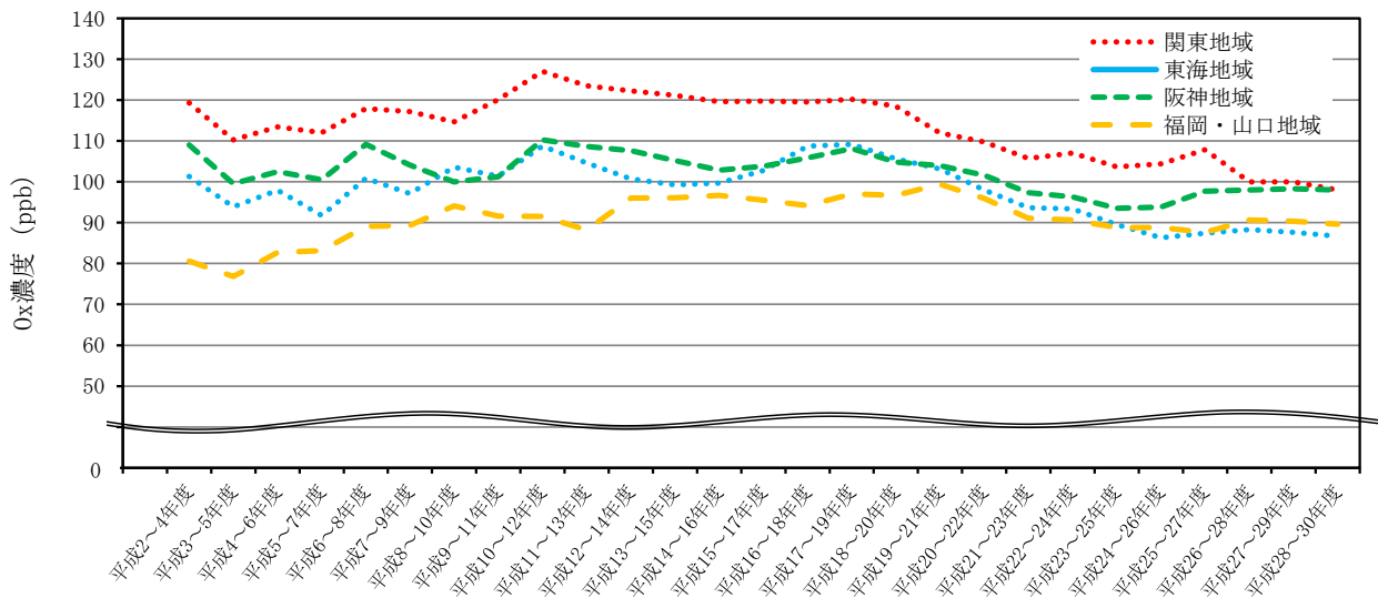
図4-2-7 光化学オキシダント濃度の長期的な改善傾向を評価するための指標（8時間値の日最高値の年間99パーセンタイル値の3年平均値）を用いた域内最高値の経年変化
