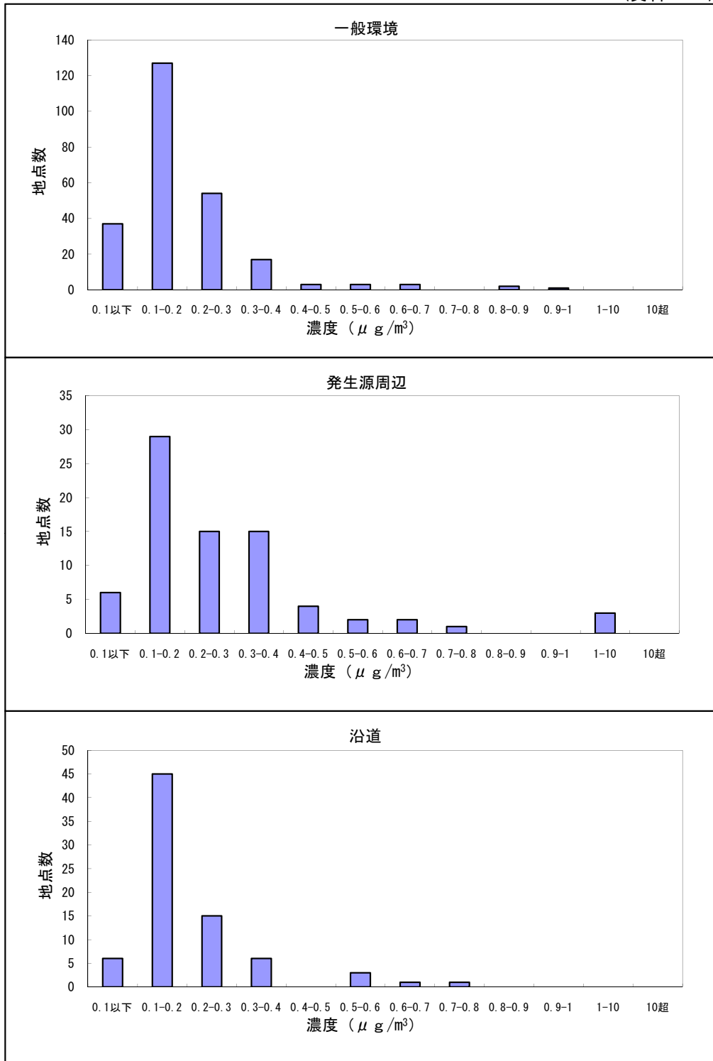
クロロホルムの大気環境中濃度分布
