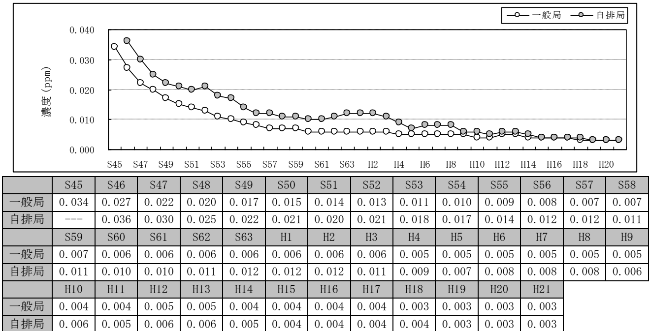
図 4-2 二酸化硫黄濃度の年平均値の推移
