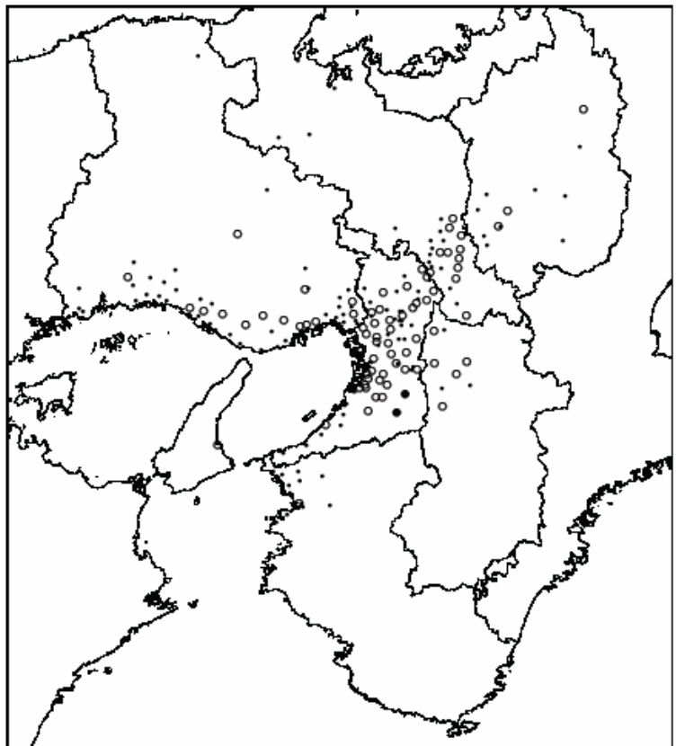
図3 - 5 注意報レベル(0.12ppm以上)の濃度が出現した日数の分布(関東地域、関西地域)
