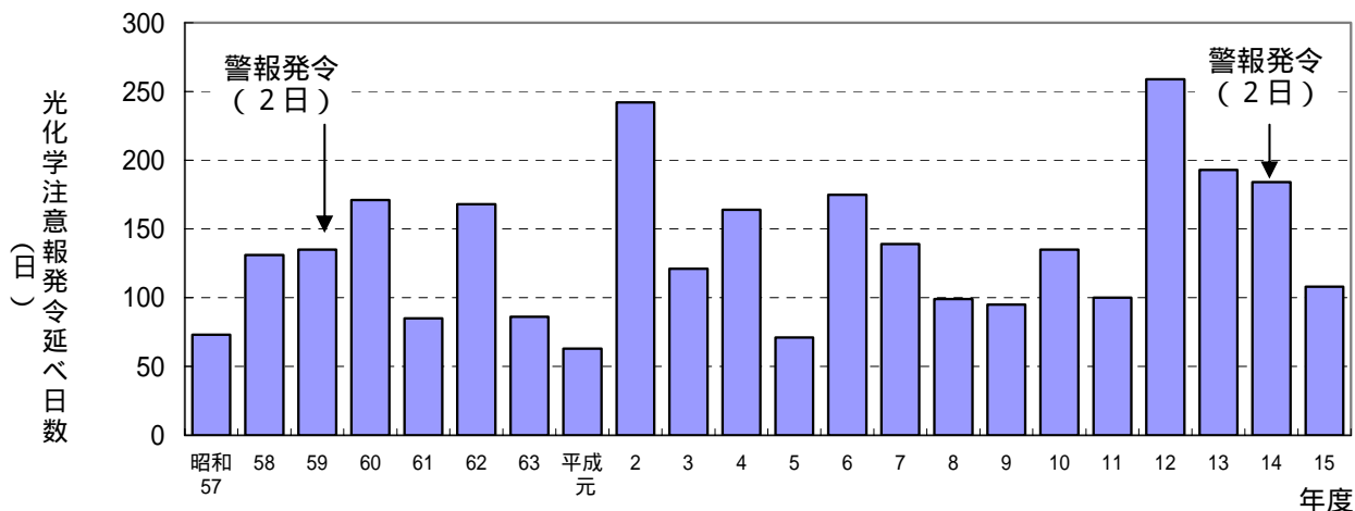
図3-2 光化学オキシダント注意報等発令日数の推移
