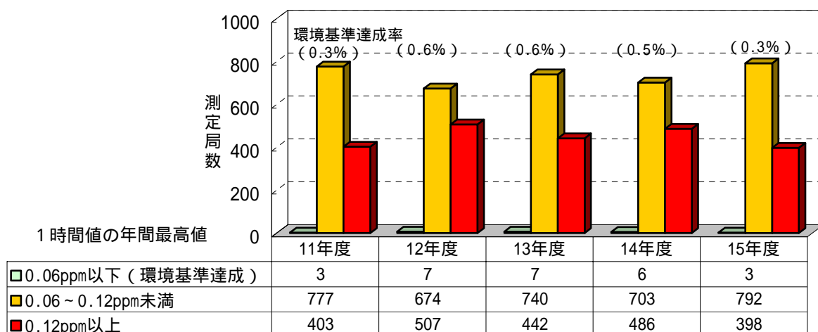
図3-1 光化学オキシダント(1時間値の最高値)濃度レベル別測定局数の推移
