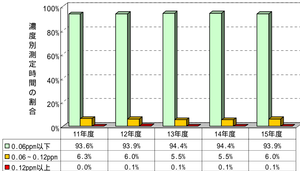
図3-3 光化学オキシダント濃度レベル別測定時間割合の推移（昼間）
