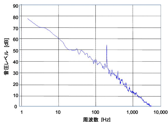
図 8 純音性成分を含む風車騒音の例 (FFT 狭帯域分析)
