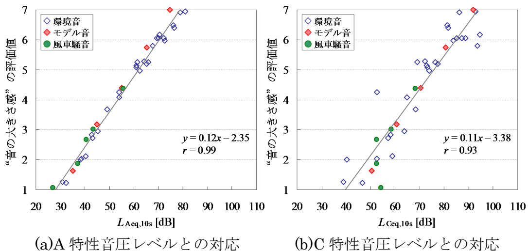
図 6 「音の大きさ」の判断結果と A 特性音圧レベル、C 特性音圧レベル (6)
