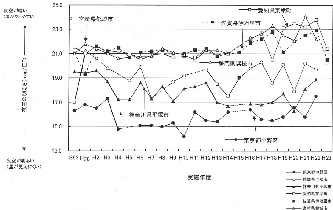
図 6 同一観測地点での夜空の明るさの推移（夏期）
