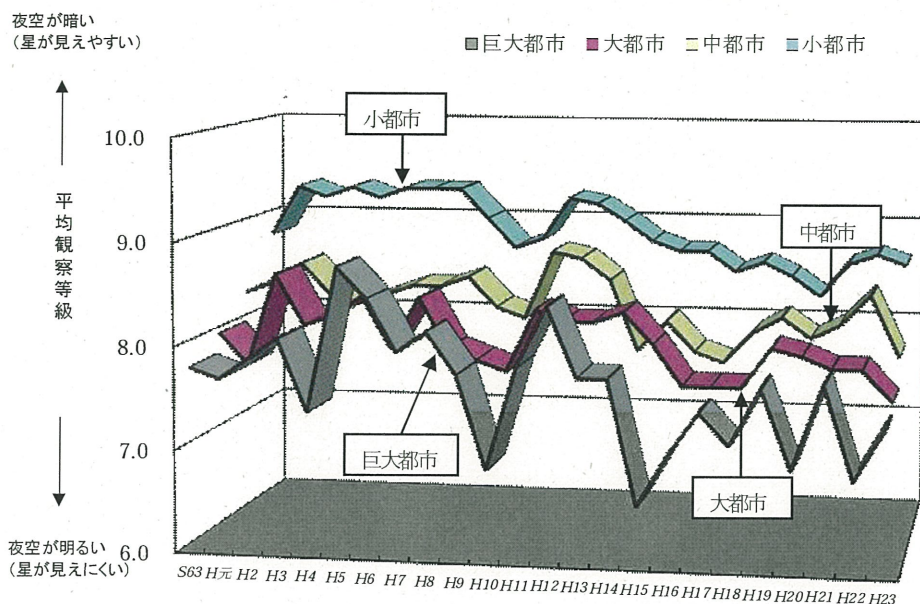
図4 都市規模別平均観察等級の推移（夏期）
