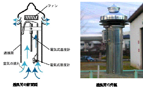
図 4.2 強制通風方式 資料) 気象庁
