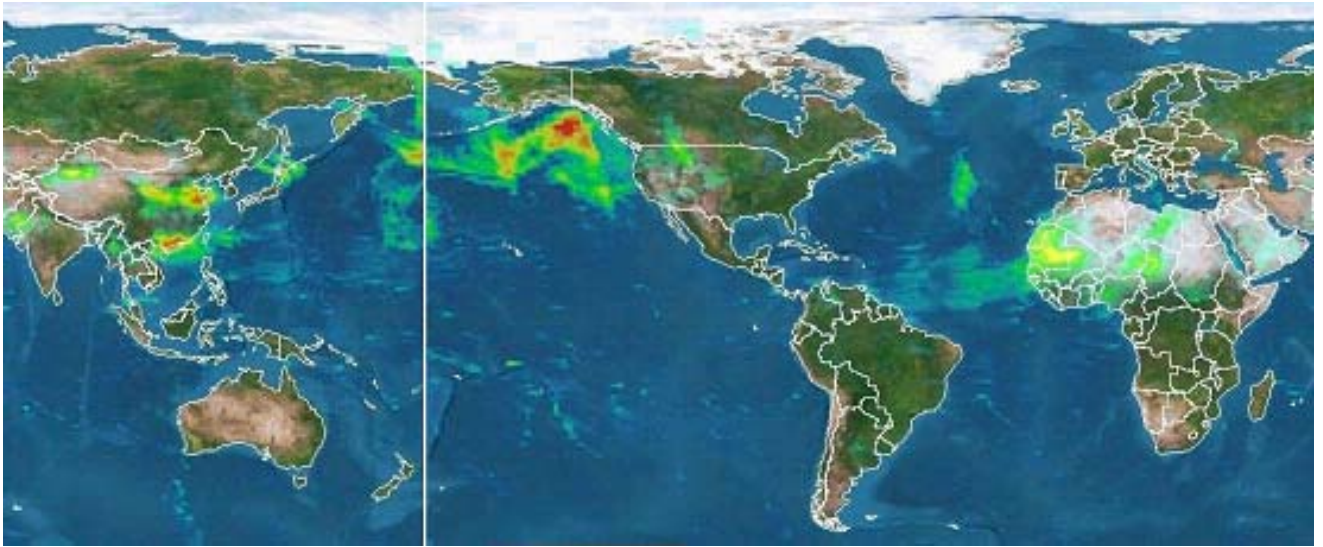
口絵 - 1 太平洋を横断するスケールの黄砂、2001年4月13日 (Earth Probe TOMS 2001)
