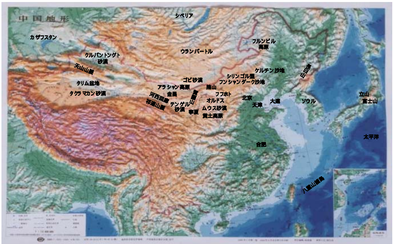
口絵 - 2 黄砂発生源地域・影響地域
