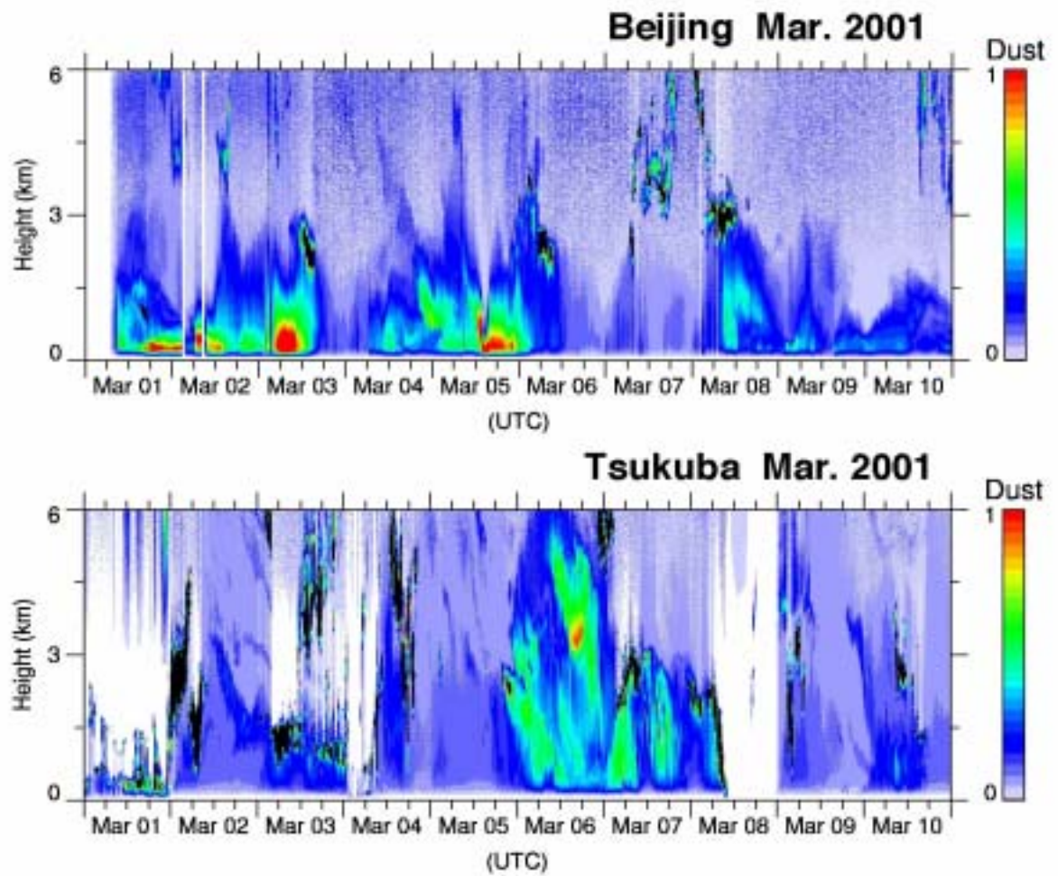
口絵 - 4 ライダー装置による黄砂観測記録 (西川 2003)
