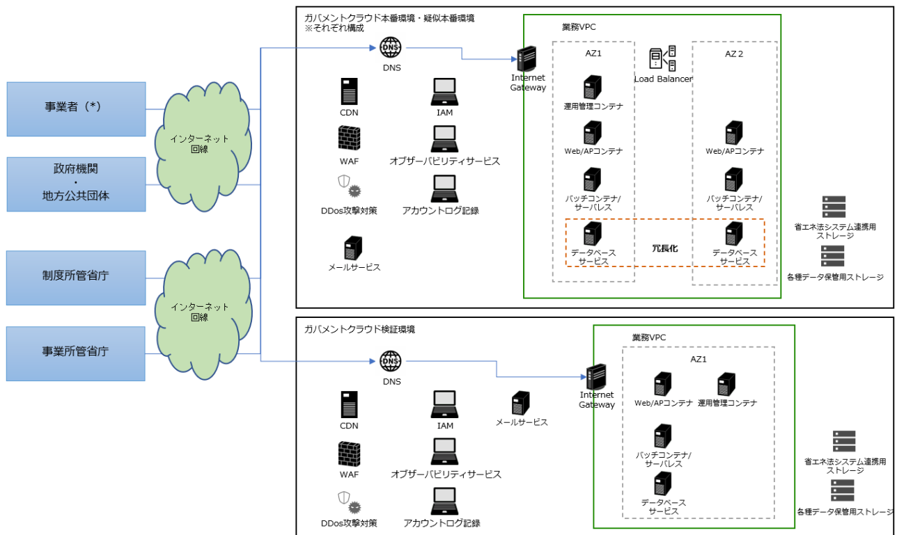
図 3-1 システム構成図 (本システムの本番環境・疑似本番環境・検証環境)
