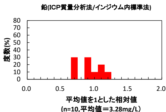
図 2-2-3-2(4) ICP 質量分析法のうちインジウム内標準法のヒストグラム
