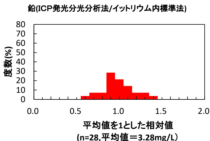
図 2-2-3-2(1) ICP 発光分光分析法のうちイットリウム内標準法のヒストグラム
