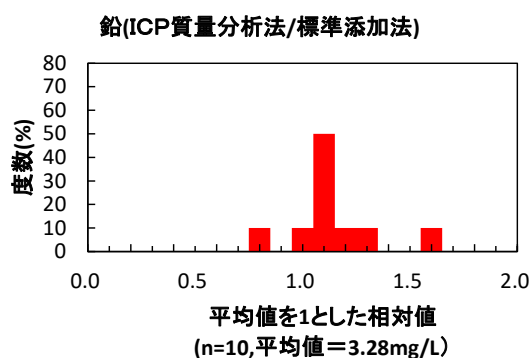
図 2-2-3-2(2) ICP 質量分析法のうち標準添加法のヒストグラム
