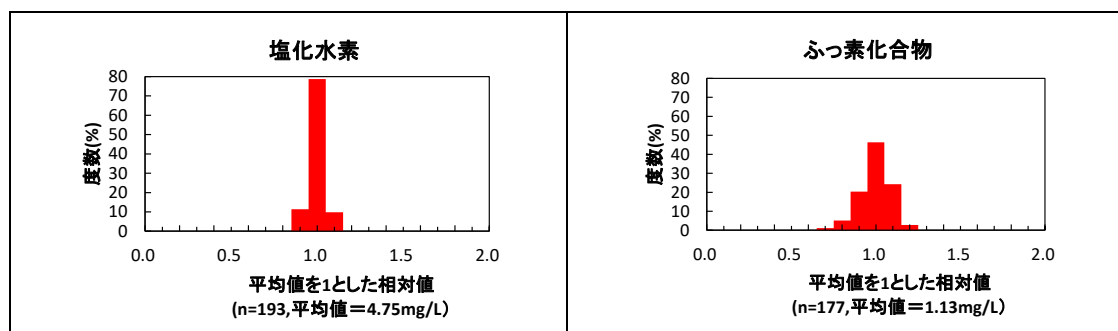
図 2-1-4 (2) 共通試料 2 (模擬排ガス吸収液試料：塩化水素等) に関するヒストグラム
