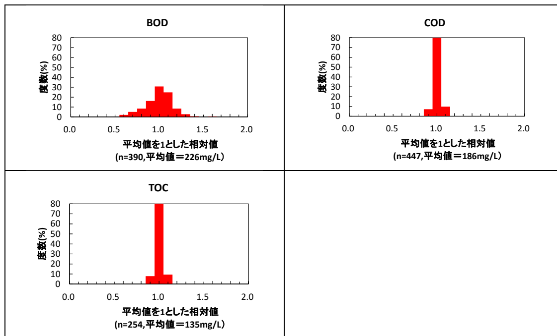
図 2-1-4(1) 共通試料 1（模擬排水試料：一般項等）に関するヒストグラム
