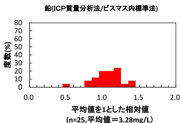
図 2-2-3-2(3) ICP 質量分析法のうちビスマス内標準法のヒストグラム
