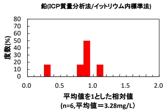
図 2-2-3-2(5) ICP 質量分析法のうちイットリウム内標準法のヒストグラム
