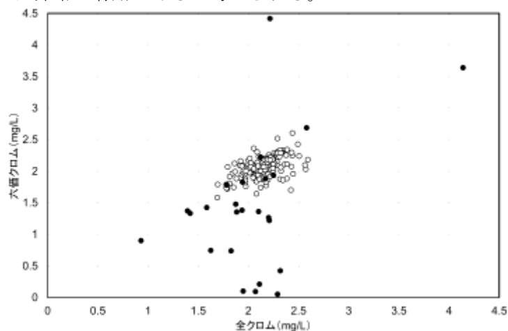
図 2-2-3-5(1) 全クロムと六価クロムと全クロムの報告値の比較
