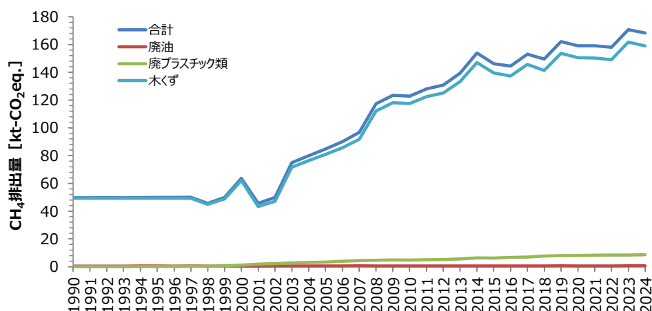
図 2 廃棄物の原燃料利用に伴う CH 4 排出量（産業廃棄物）の推移
