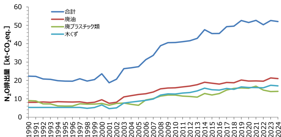
図 3 廃棄物の原燃料利用に伴う N 2 O 排出量（産業廃棄物）の推移
