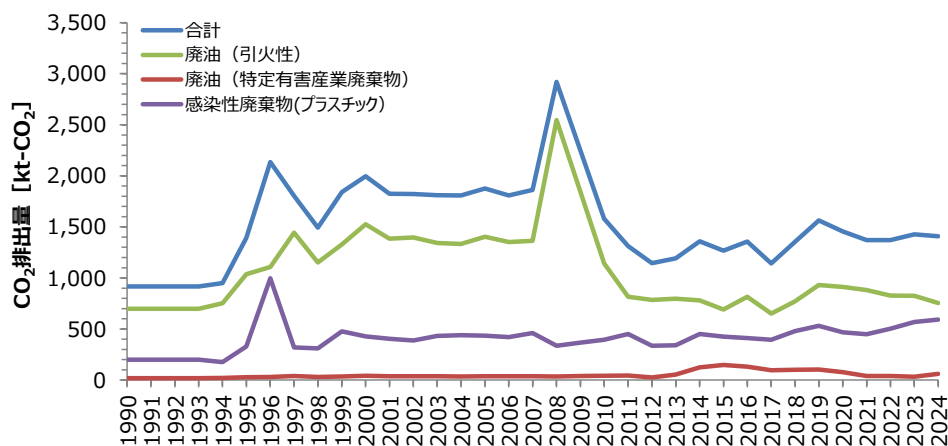
図 1 廃棄物の単純焼却に伴う CO 2 排出量（特別管理産業廃棄物）の推移
