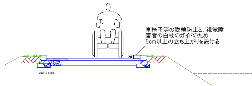
図 15 路側の立ち上がりは 5cm 以上とす ズ
