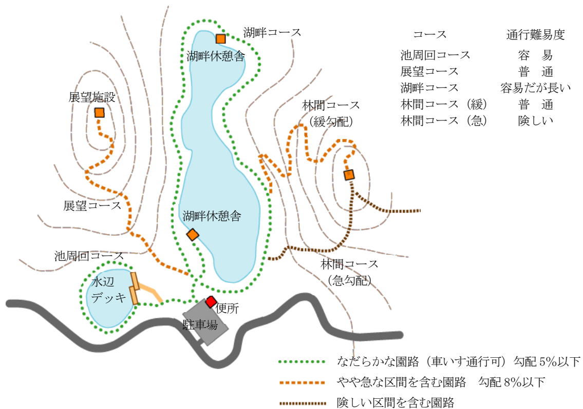
図 14 多様な園路ネットワークの整備例
