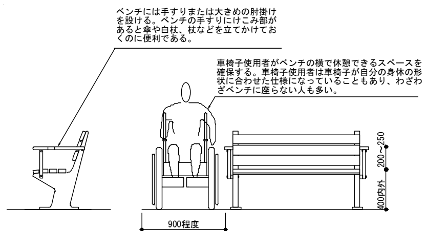
図 18 ベンチの例
