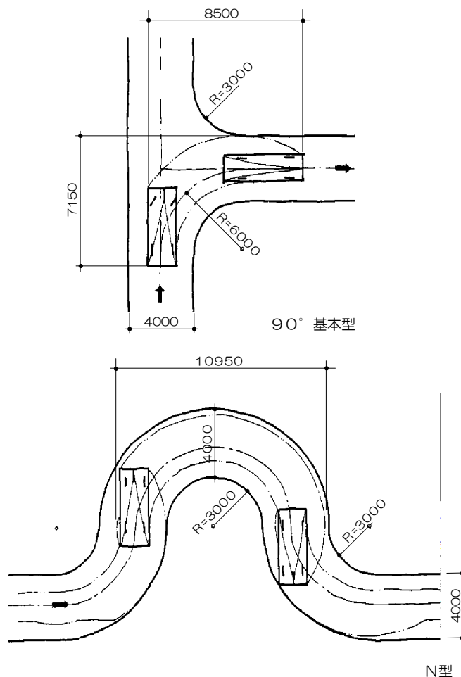
図 8 車両の回転半径の事例
