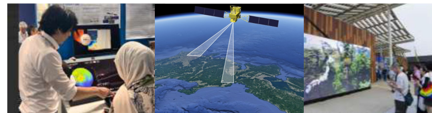
↑ GOSAT観測データの説明
