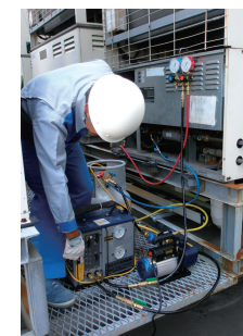
スーパーマーケット冷蔵ショーケース(室外機)からのフロン類冷媒回収の様子
