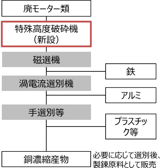
新設した破砕・選別フローの概略
