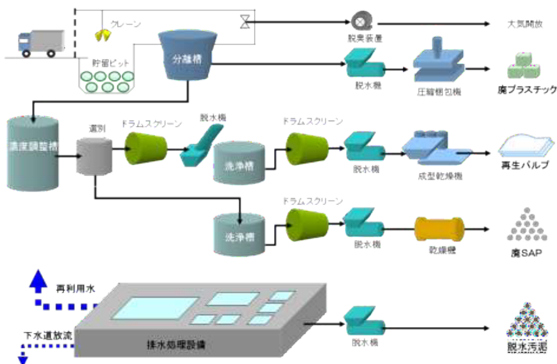
図 5-1 「水溶化・分離処理によるパルプ・プラスチック回収」の流れ
