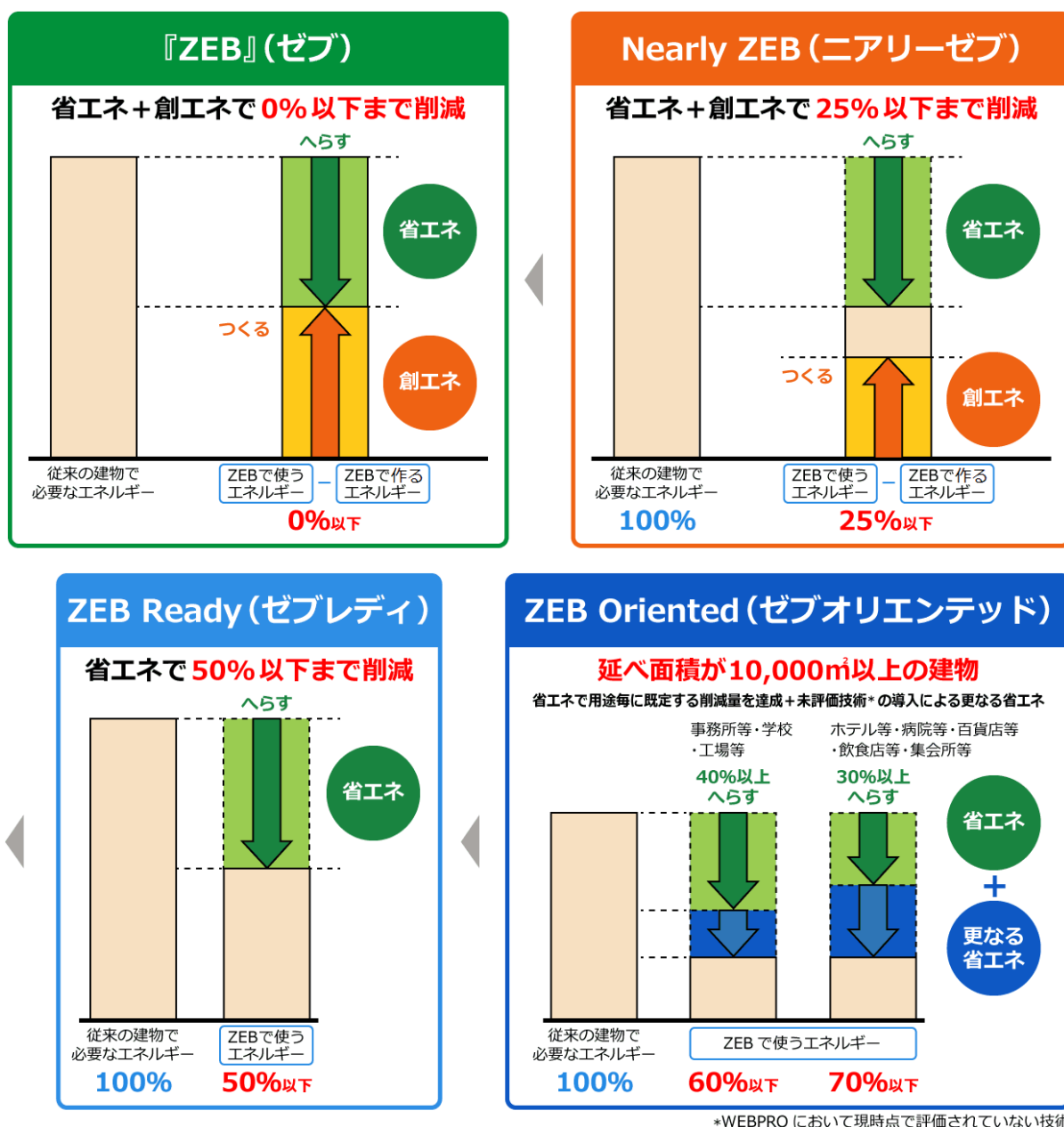
図1 4段階のZEBの定義
