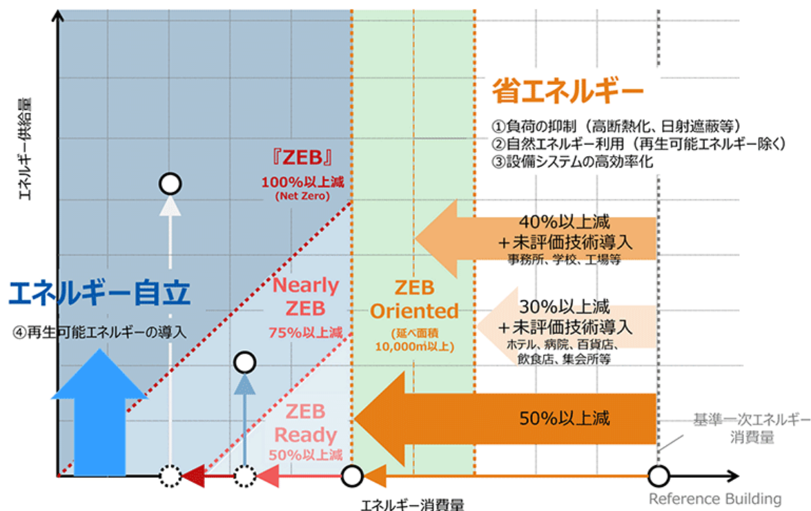
図 2 ZEB の定義及び対応の方向
