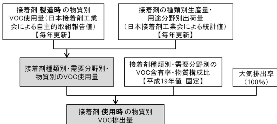
図 13 接着剤使用による VOC 排出量推計フロー
