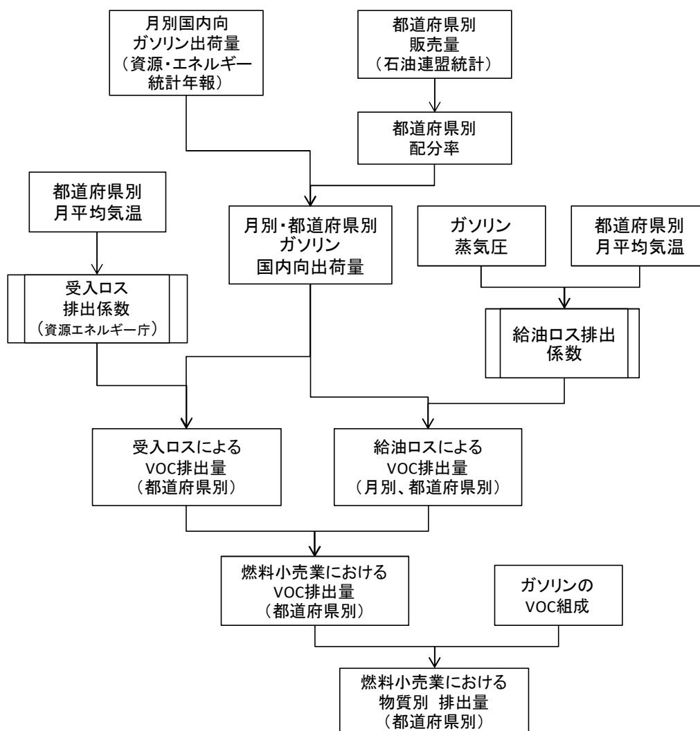
図 1 給油所における VOC 排出量の推計フロー
