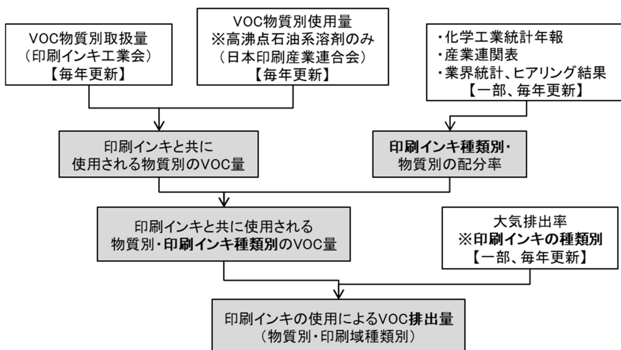
図 7 印刷インキの使用による VOC 排出量推計フロー(概要)
