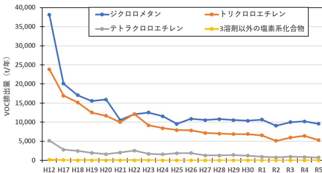
図 17 工業用洗浄剤の使用による物質別排出量の推移(工業用洗浄剤:塩素系洗浄剤)
