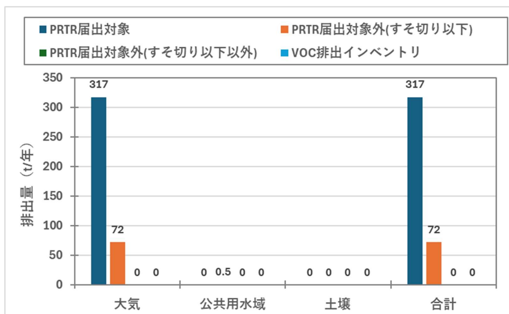
図 25 媒体別排出量(1-ヘキセン)
