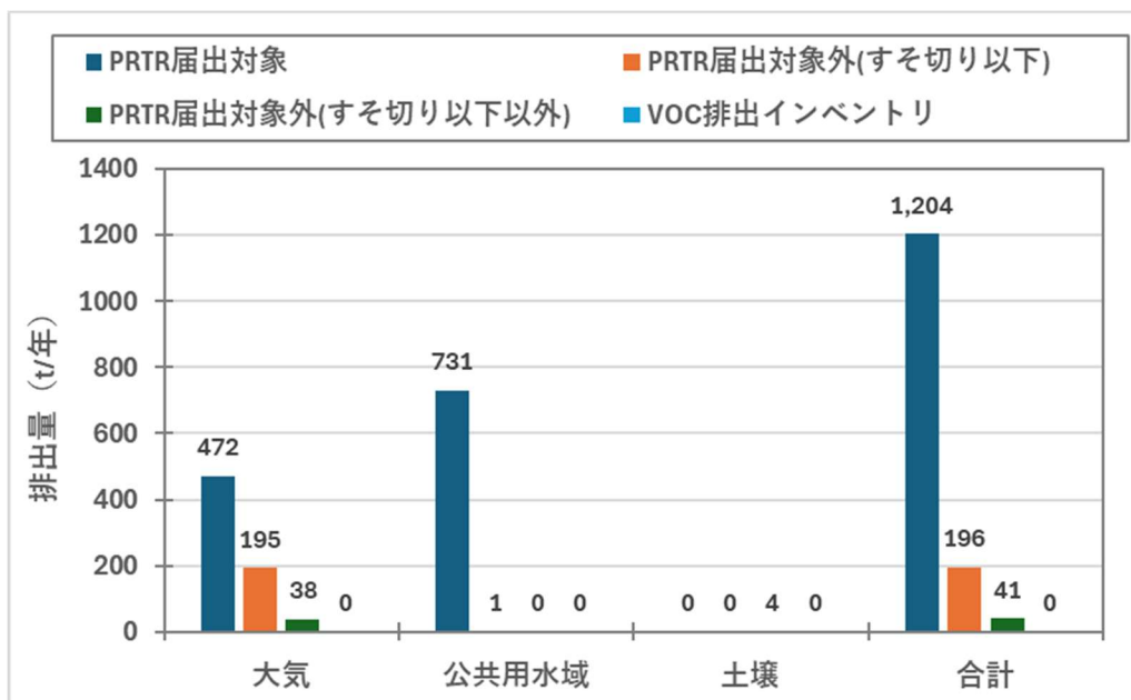
図 27 媒体別排出量(N-メチル-2-ピロリドン)
