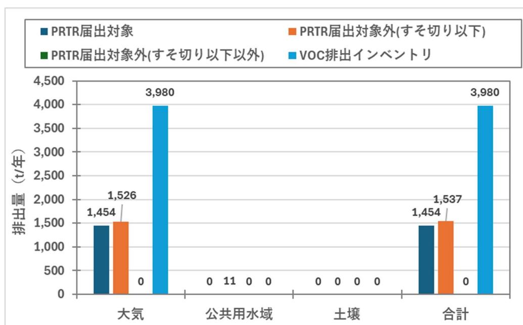
図 23 媒体別排出量(シクロヘキサン)
