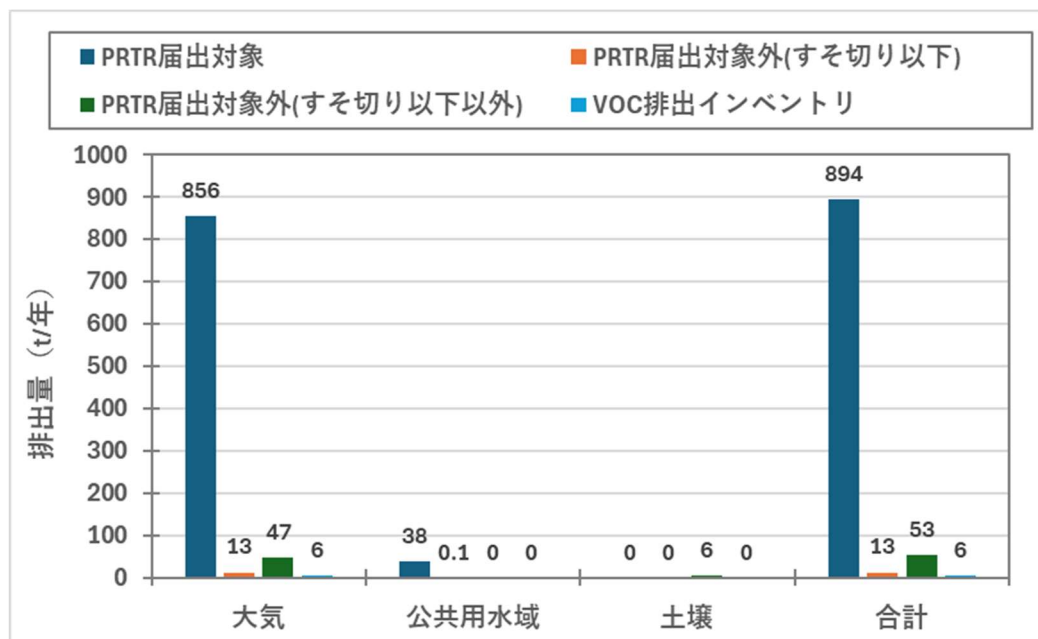
図 22 媒体別排出量(ジエチレングリコールモノブチルエーテル)
