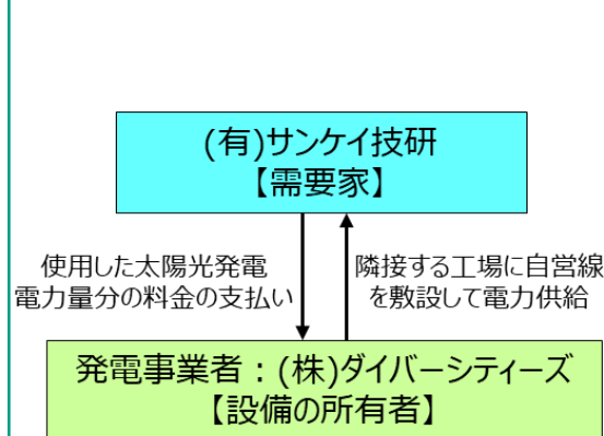
電力需要施設 ((有)サンケイ技研 工場)
