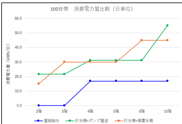
消費電力量
