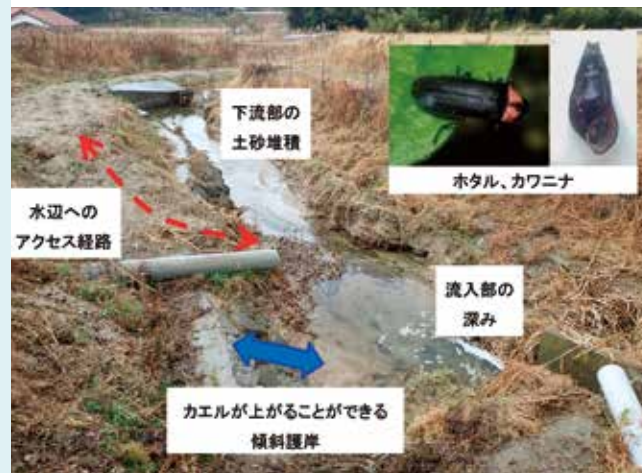
① 環境配慮型水路(整備後6年経過時点)
