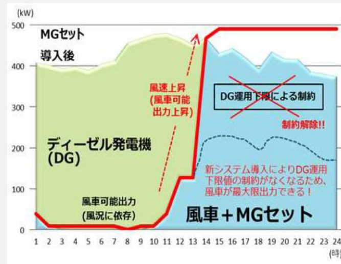
風車 + MGセットの運用イメージ
