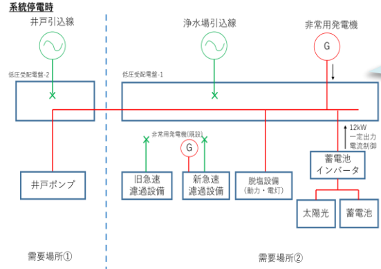
系統停電時のシステム構成
