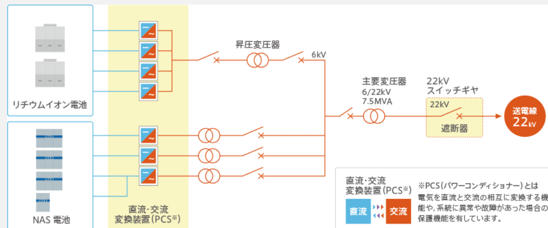
リチウムイオン電池とNAS電池の系統接続イメージ
