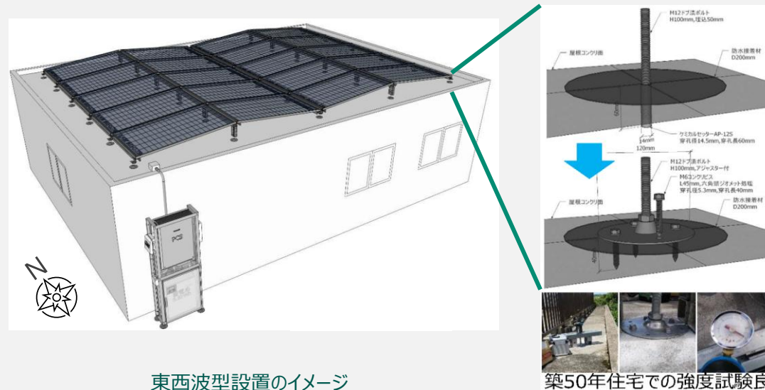
プラグレスアンカー施工のイメージ
