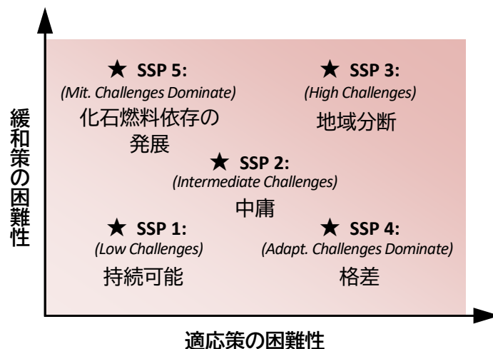
図 19 SSP1～SSP5 のコンセプト
