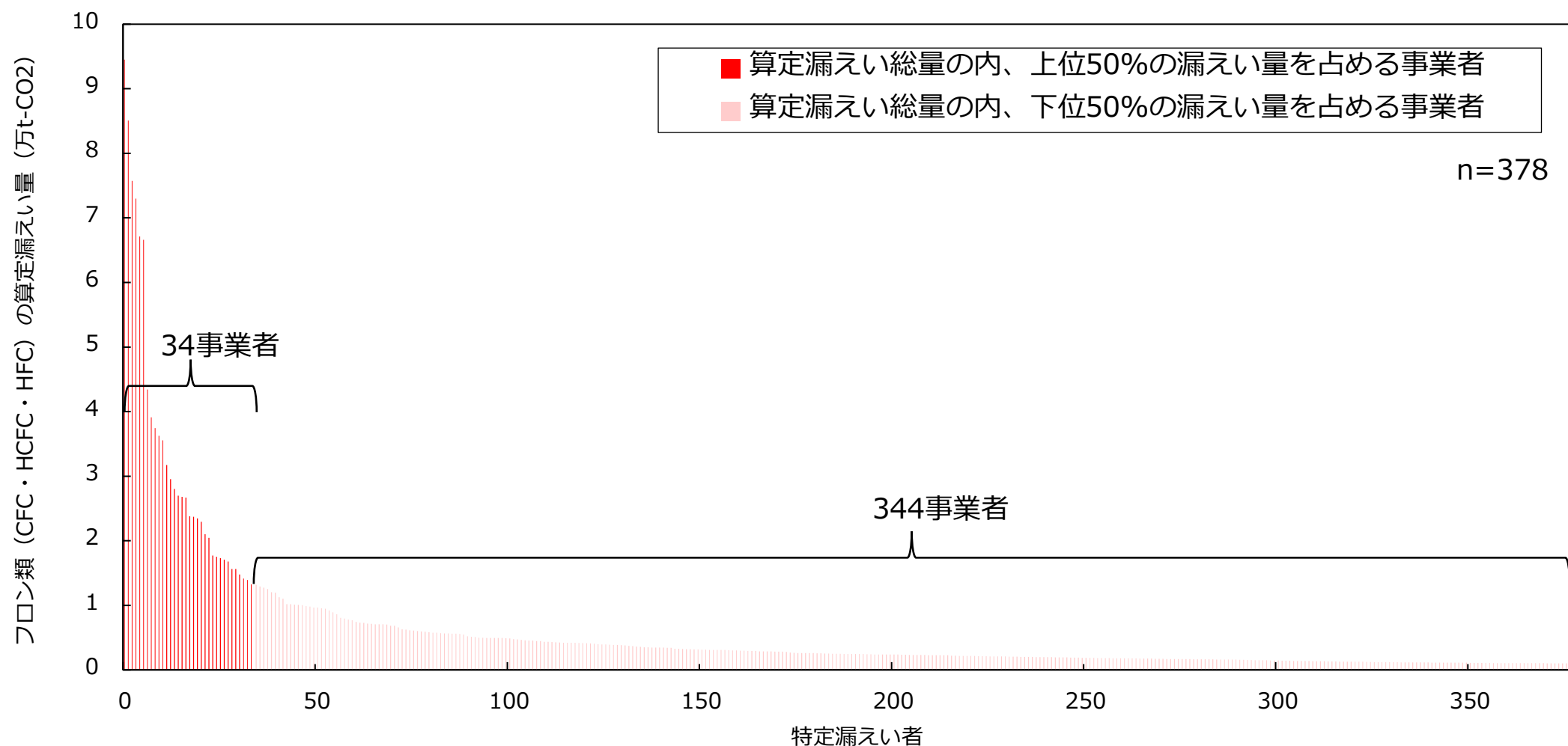
図. 事業者別の算定漏えい量
