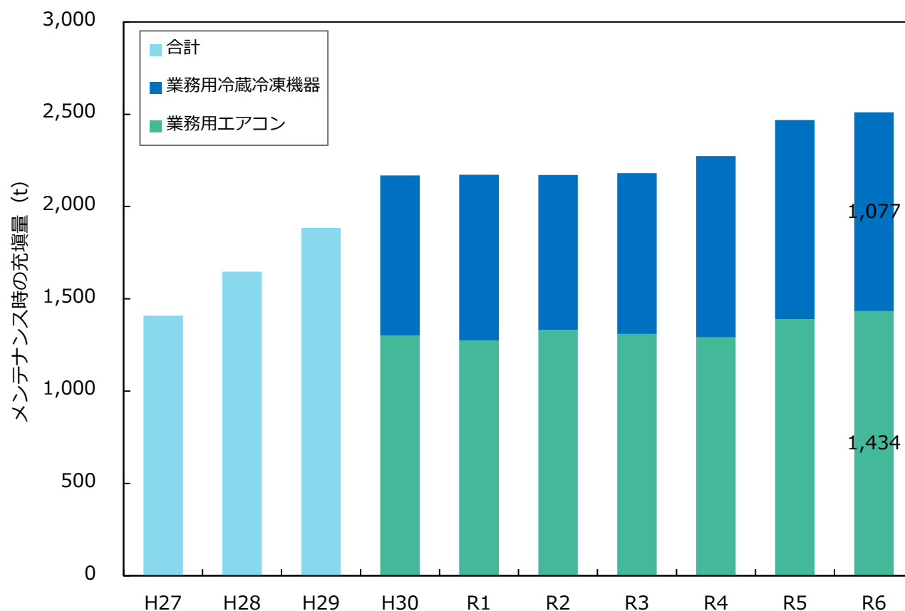
稼動中機器のメンテナンス時の充填量（HFCsのみ）
