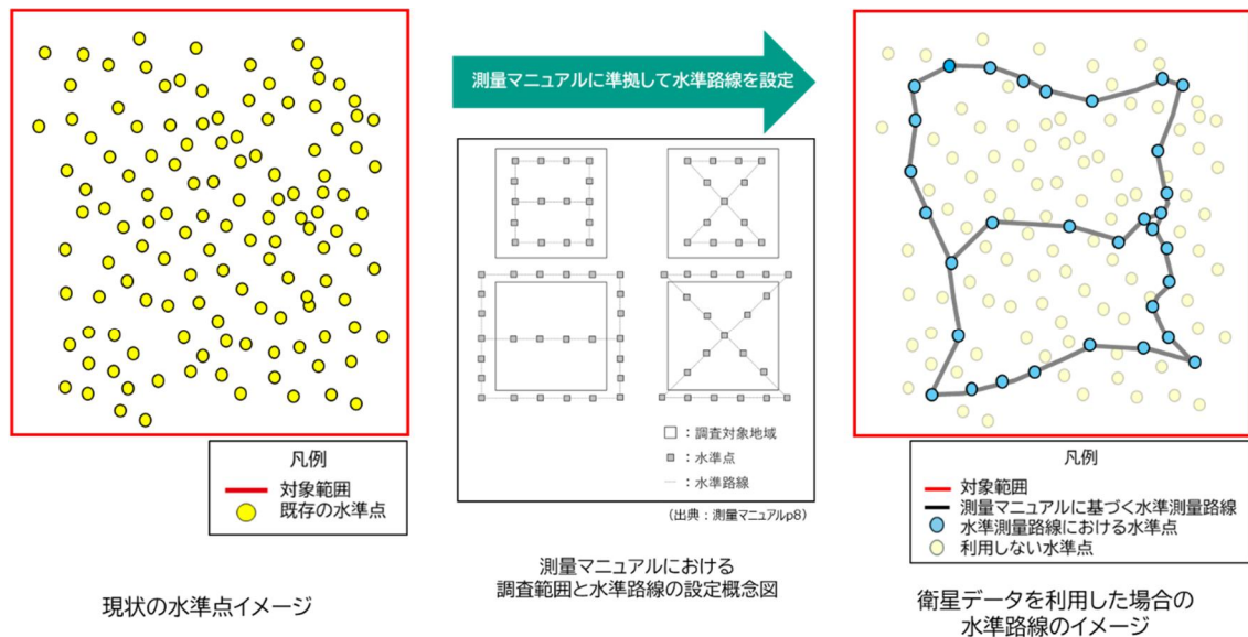
図 1-6 衛星データと水準測量を併用した測量作業の効率化のイメージ
