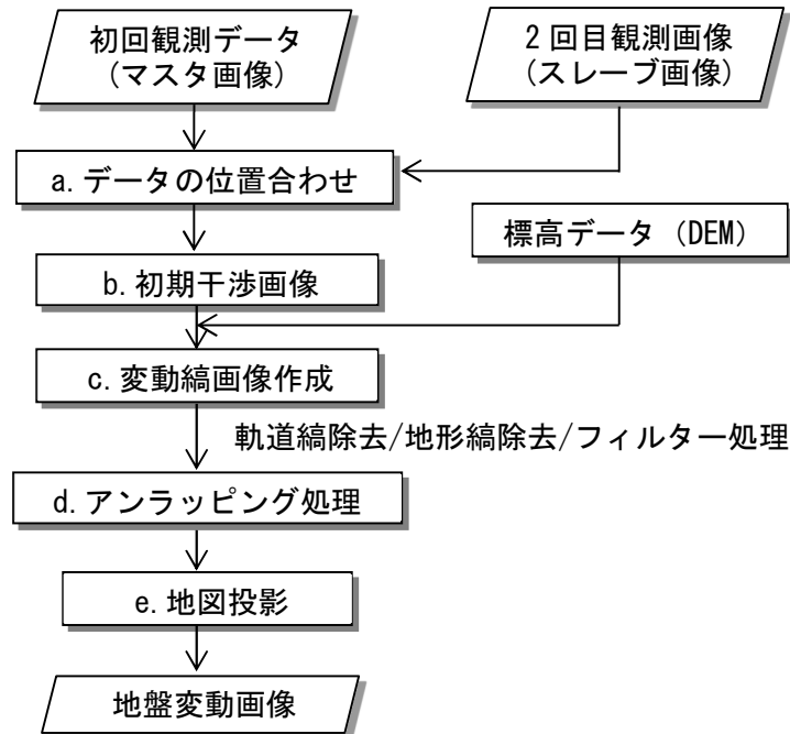
図 2-15 1 ペアの干渉 SAR 解析の流れ
