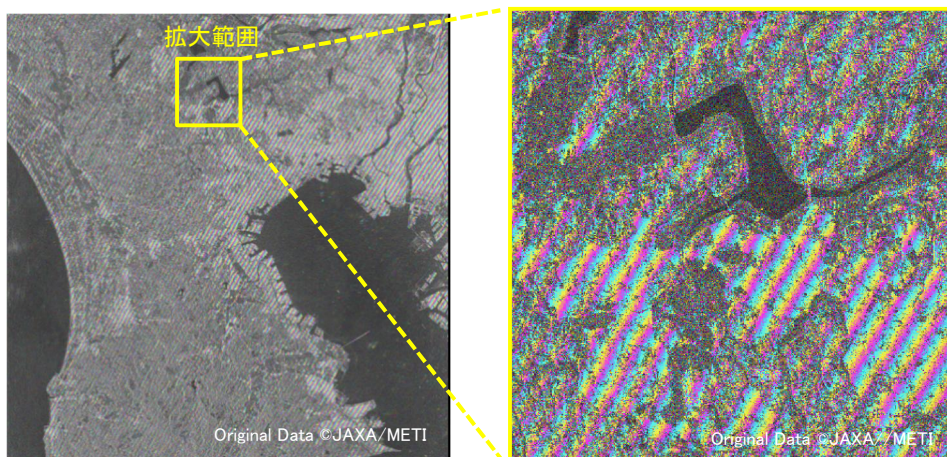
図 2-17 初期干渉画像の例 (ALOS データ利用)
