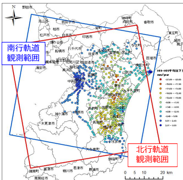
図 3-1 九十九里平野を対象とした ALOS での観測範囲と精度検証に用いた水準点の分布
