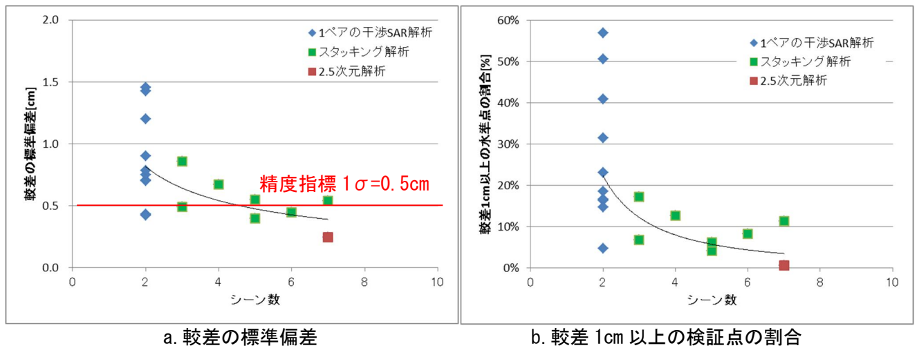
図 2-9 干渉 SAR 解析のシーン数と精度の関係（対象地：九十九里平野）
