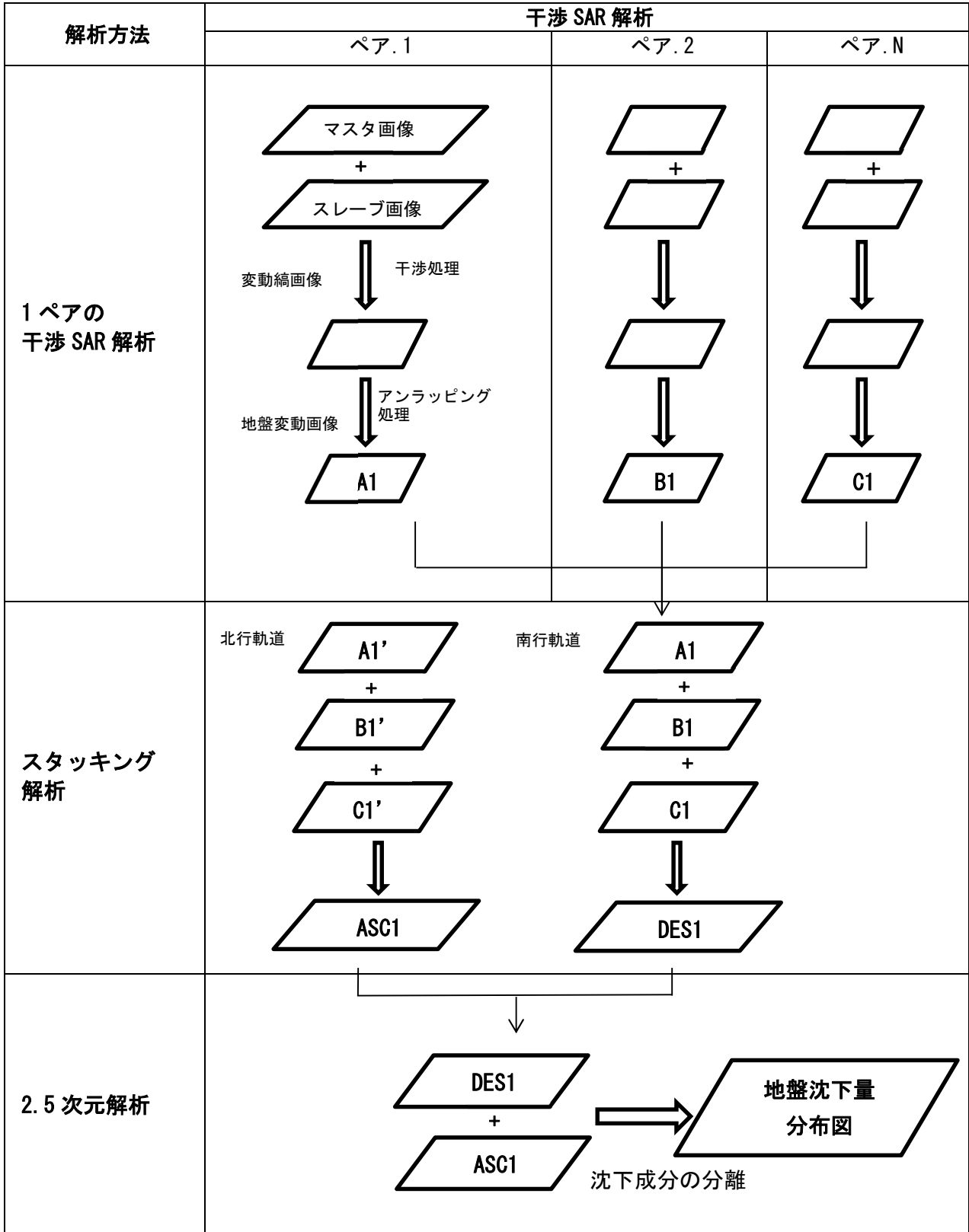
図 2-14 干渉 SAR 解析の全体の流れ
