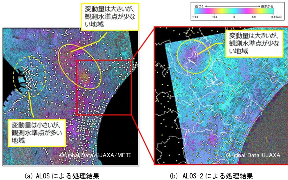
図 3-12 干渉 SAR 解析による変動画像と水準測量観測点の重ね合わせ結果の例
