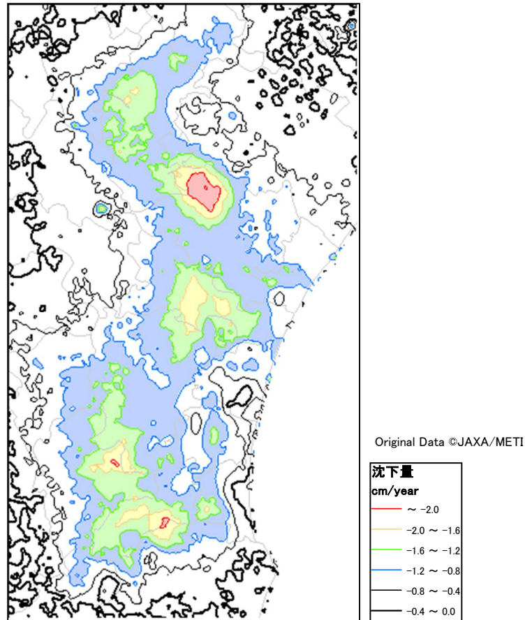
図 2-24 干渉 SAR 解析による地盤沈下量分布図の解析例 (千葉県九十九里平野)
