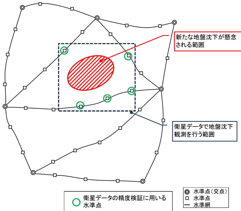
図 2-5 衛星データの精度検証に用いる水準点の位置
