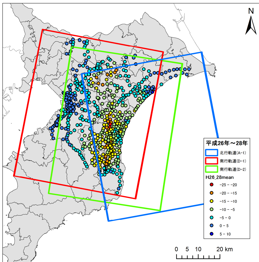
図 3-7 九十九里平野を対象とした ALOS-2 での観測範囲と精度検証に用いた水準点の分布
