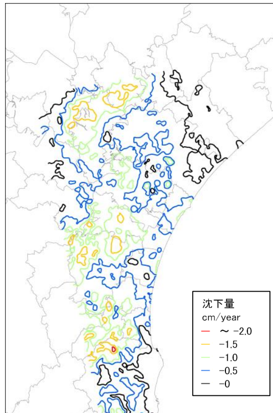
図 3-11 九十九里平野における ALOS-2 による地盤沈下量分布図
