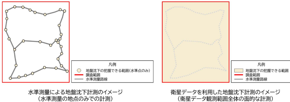
図 1-7 水準測量による地盤沈下計測と衛星データを利用した地盤沈下計測のイメージ (計測範囲の違い)
