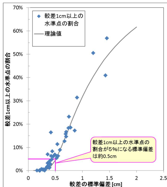
図 2-8 較差の標準偏差と較差 1cm 以上の点の割合の関係
