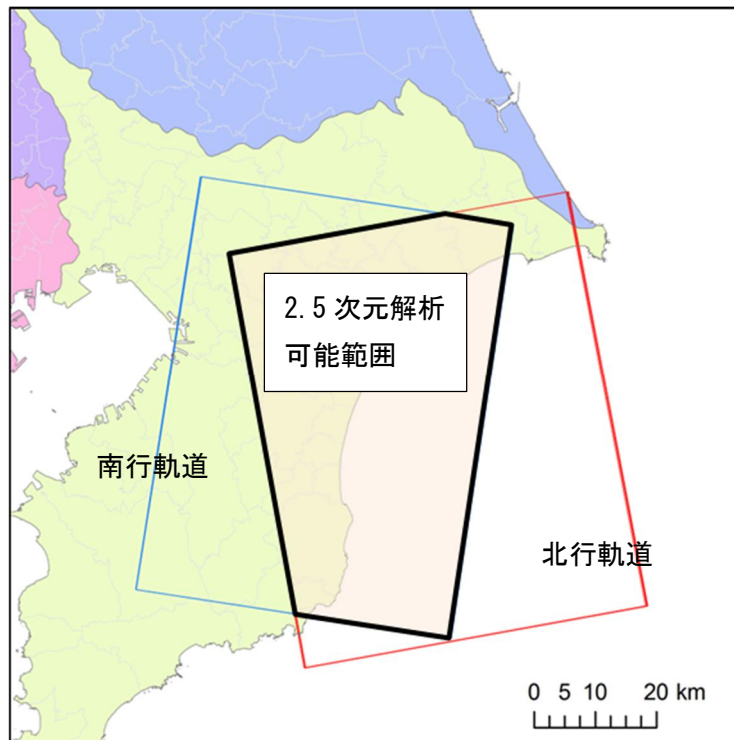
図 2-7 九十九里平野の2.5次元解析の解析可能範囲例
