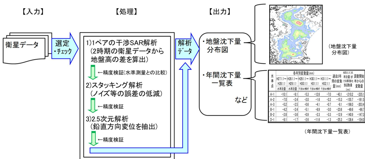
図 1-2 地盤沈下観測のための作業手順 (概略)
