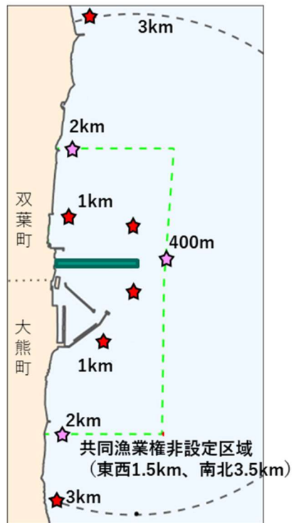
図1 測点図（放水口位置から約3 km 以内）
