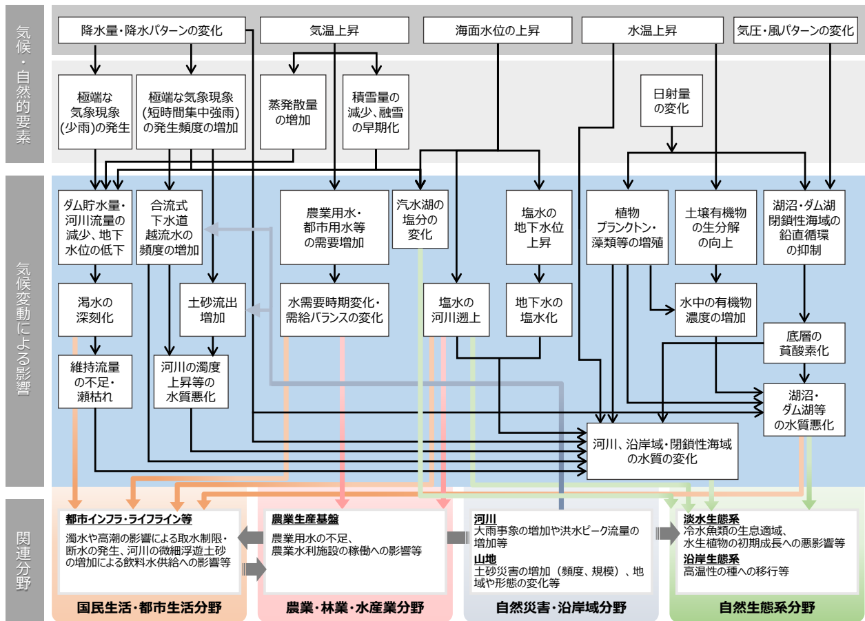
図 3-2 気候変動により想定される影響の概略図（水環境・水資源分野） 6
