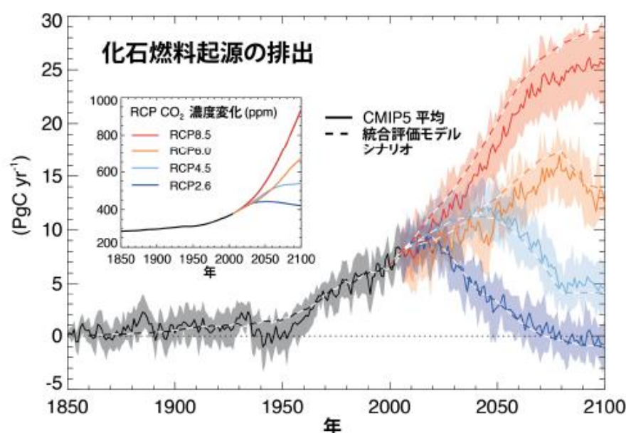
図A-1 RCPシナリオに基づく二酸化炭素の濃度変化(図内側)とRCP シナリオに対応する化石燃料からの二酸化炭素排出量(図外側);地球システムモデルによる逆算の結果。細線:個々のモデルの結果、太線:複数のモデルの平均)。PgCは炭素換算で10億トン( 10^{15}\text{g} )。
