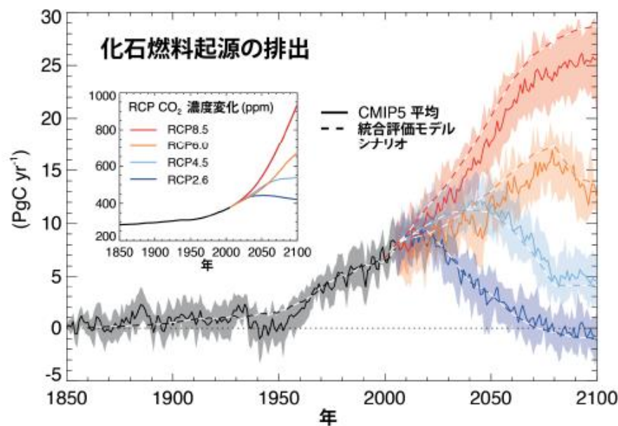
図 A-1 RCP シナリオに基づく二酸化炭素の濃度変化（図内側）と RCP シナリオに対応する化石燃料からの二酸化炭素炭素排出量（図外側；地球システムモデルによる逆算の結果。細線：個々のモデルの結果、太線：複数のモデルの平均）。PgC は炭素換算で 10 億トン（10 15 g）。
