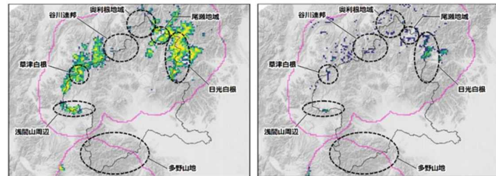
群馬県周辺における亜高山帯針葉樹林の植生図
