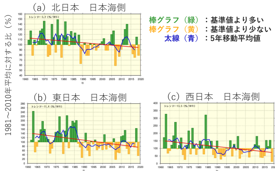
図13 日本の年最深積雪深の基準値に対する比の経年変化（1962～2019年）
