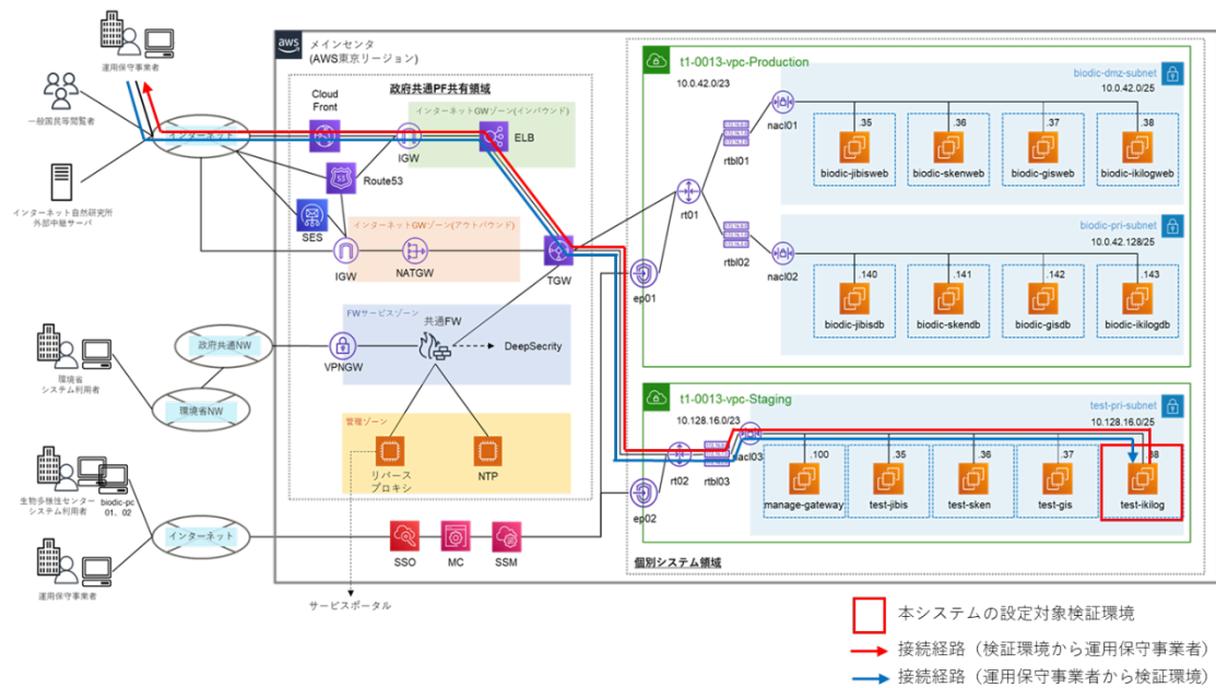
図 3-1 ハードウェア構成図 (想定)
