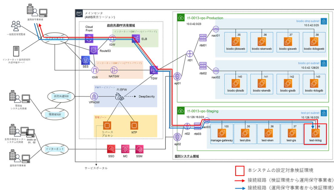
図 2 システム構成概要 (想定)
