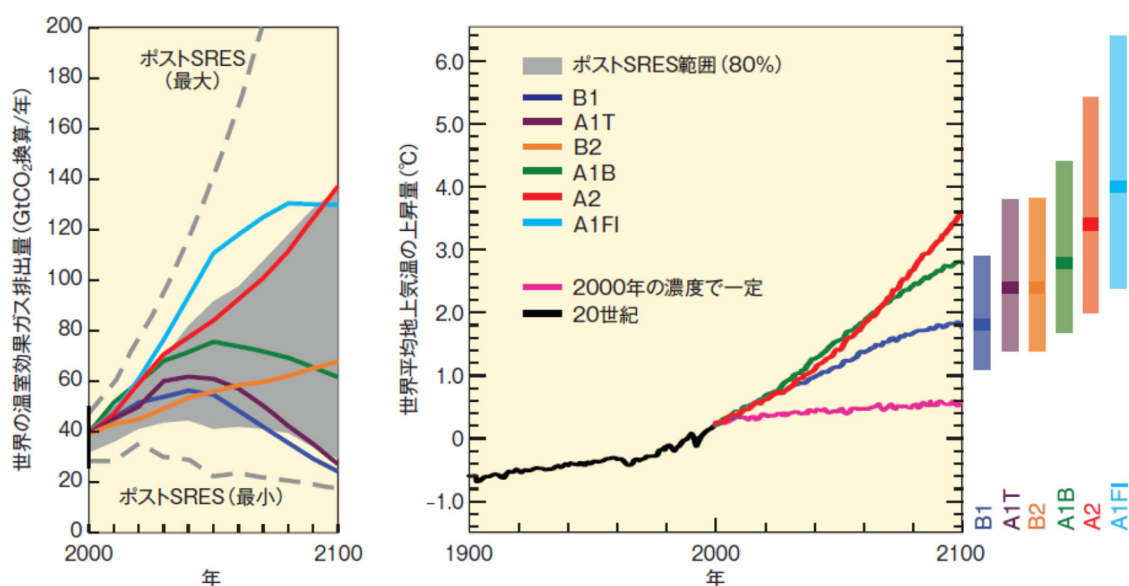
図 A-5 （左図）追加的な気候政策を含まない場合の世界の温室効果ガス排出量（CO 2 換算）：6つのSRES マーカーシナリオ（彩色した線）、SRES 以降に公表された最近のシナリオ（ポスト SRES）の 80 パーセンタイル（灰色の彩色範囲）。点線はポスト SRES シナリオ結果のすべての範囲を示す。排出量には CO 2 、CH 4 、N 2 O 及びフロンガスが含まれる。
