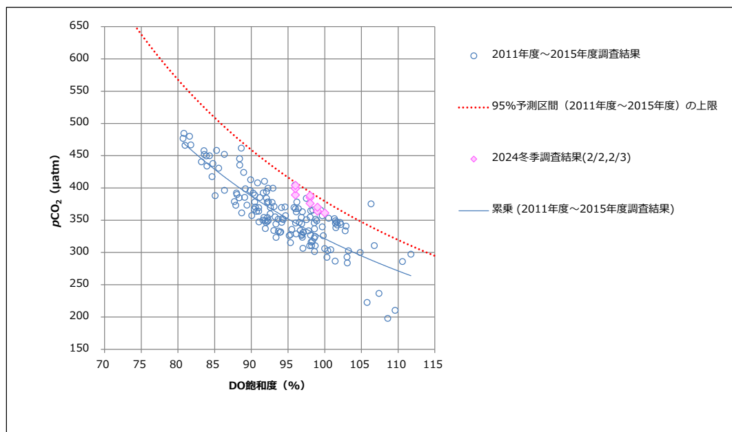
図2 p\text{CO}_2 と DO 飽和度との関係
