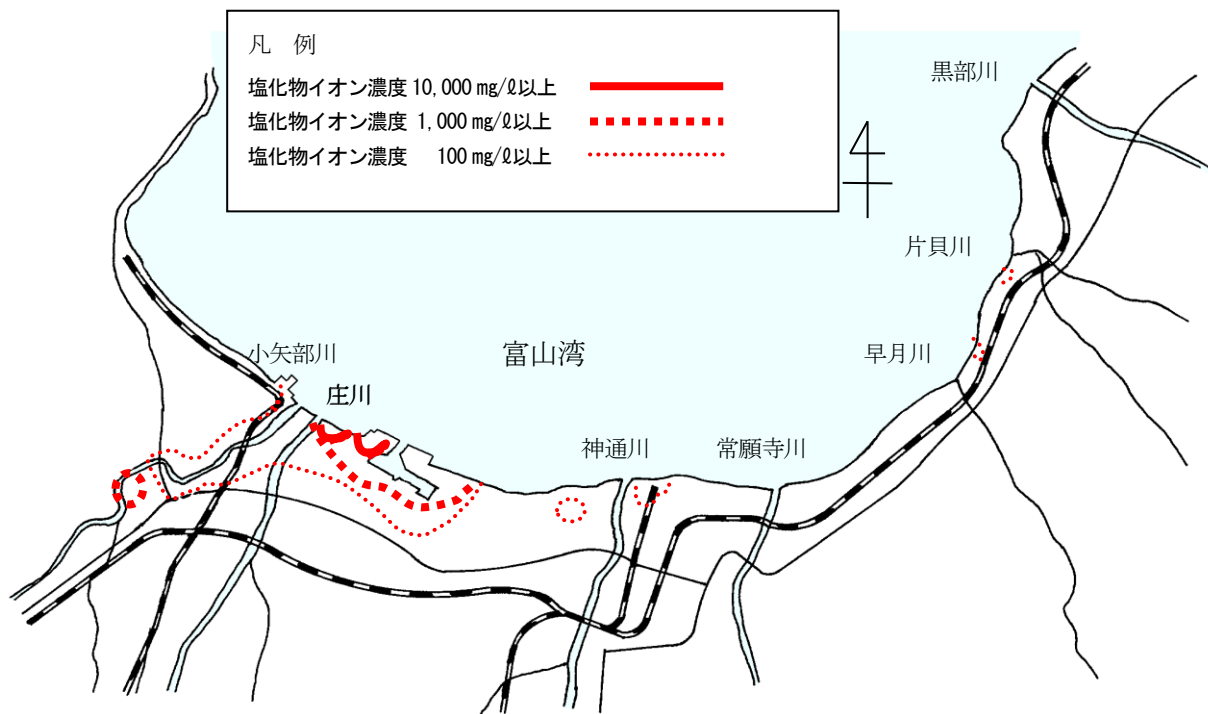
富山・砺波平野 塩素イオン濃度分布図（令和6年度）
