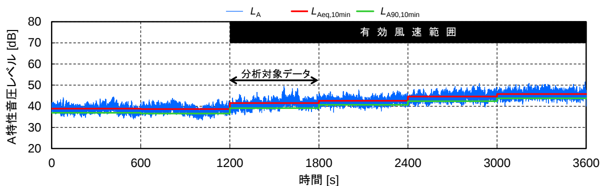
(a). 風車が停止から徐々に稼働したとき
