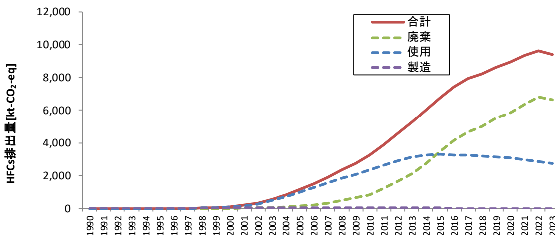
図 1 「2.F.1.- 固定空調機器（家庭用エアコン）の製造、使用及び廃棄」からの HFCs 排出量の推移
