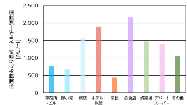
建物用途別の床面積あたり エネルギー消費原単位 (2018年)
