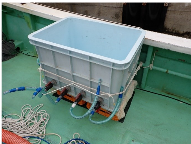
別図 11-5 400 L タンク
