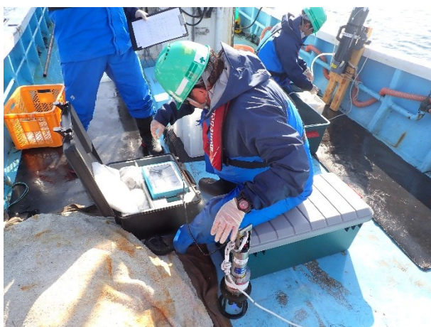
別図 11-10 CTD のデータ確認 (令和 6 年 5 月 30 日撮影)
