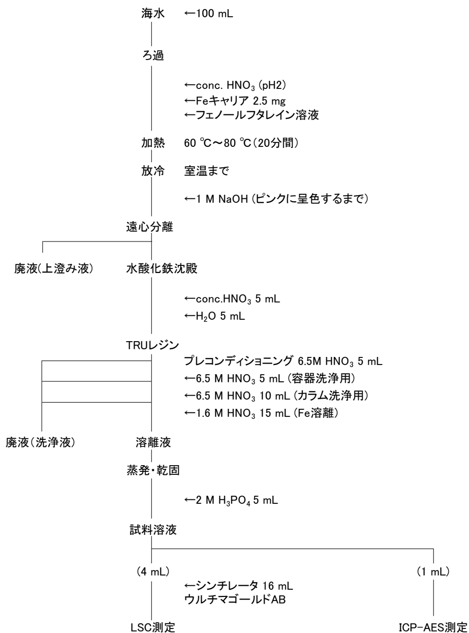
図 4-9 海水の鉄 55 分析フロー
