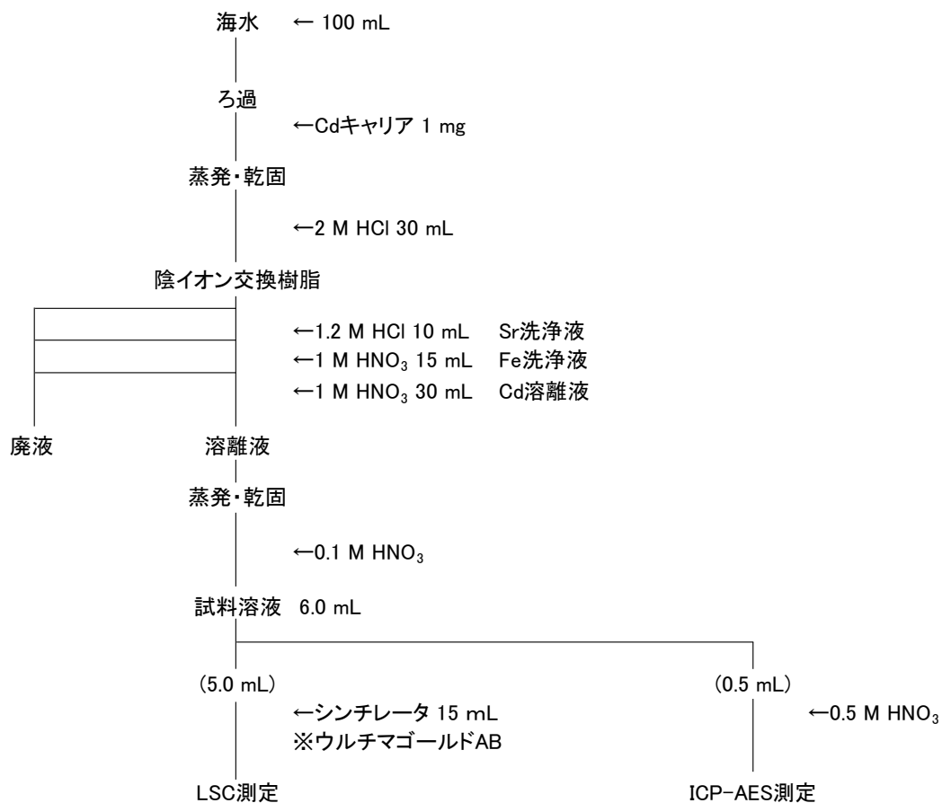
図 4-6 海水のカドミウム 113m 分析フロー
