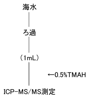
図 4-7 海水のヨウ素 129 分析フロー
