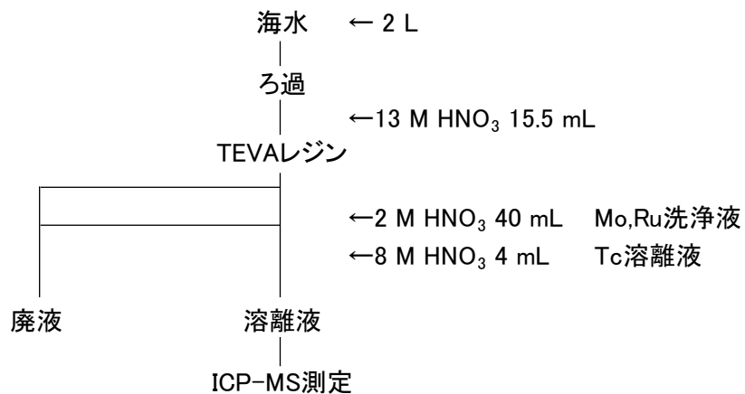
図 4-5 海水のテクネチウム 99 分析フロー
