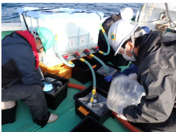
別図 11-22 20 L 容器の洗浄 (令和 6 年 11 月 12 日撮影)
