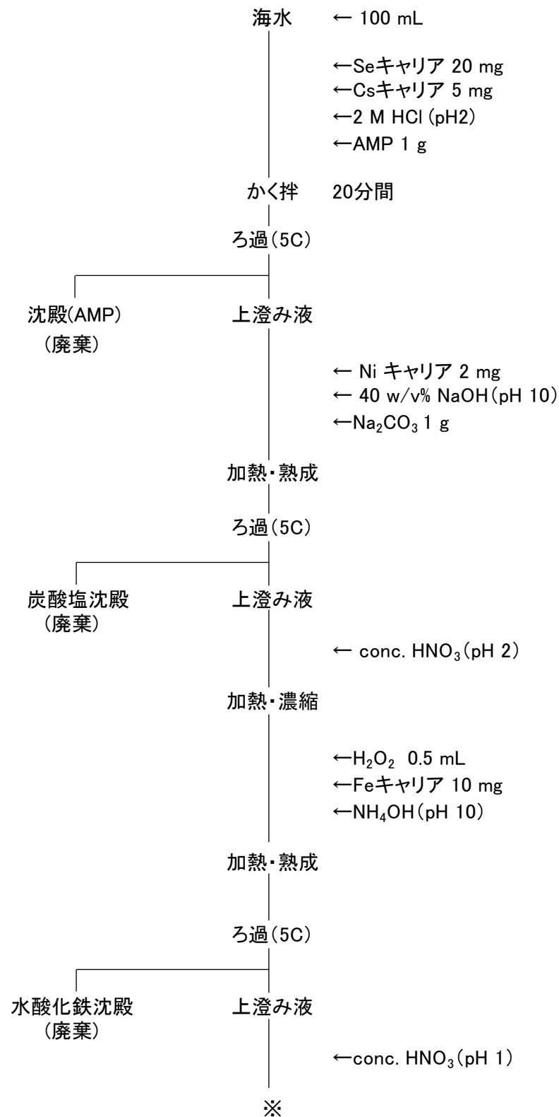
図 4-10 海水のセレン 79 分析フロー
