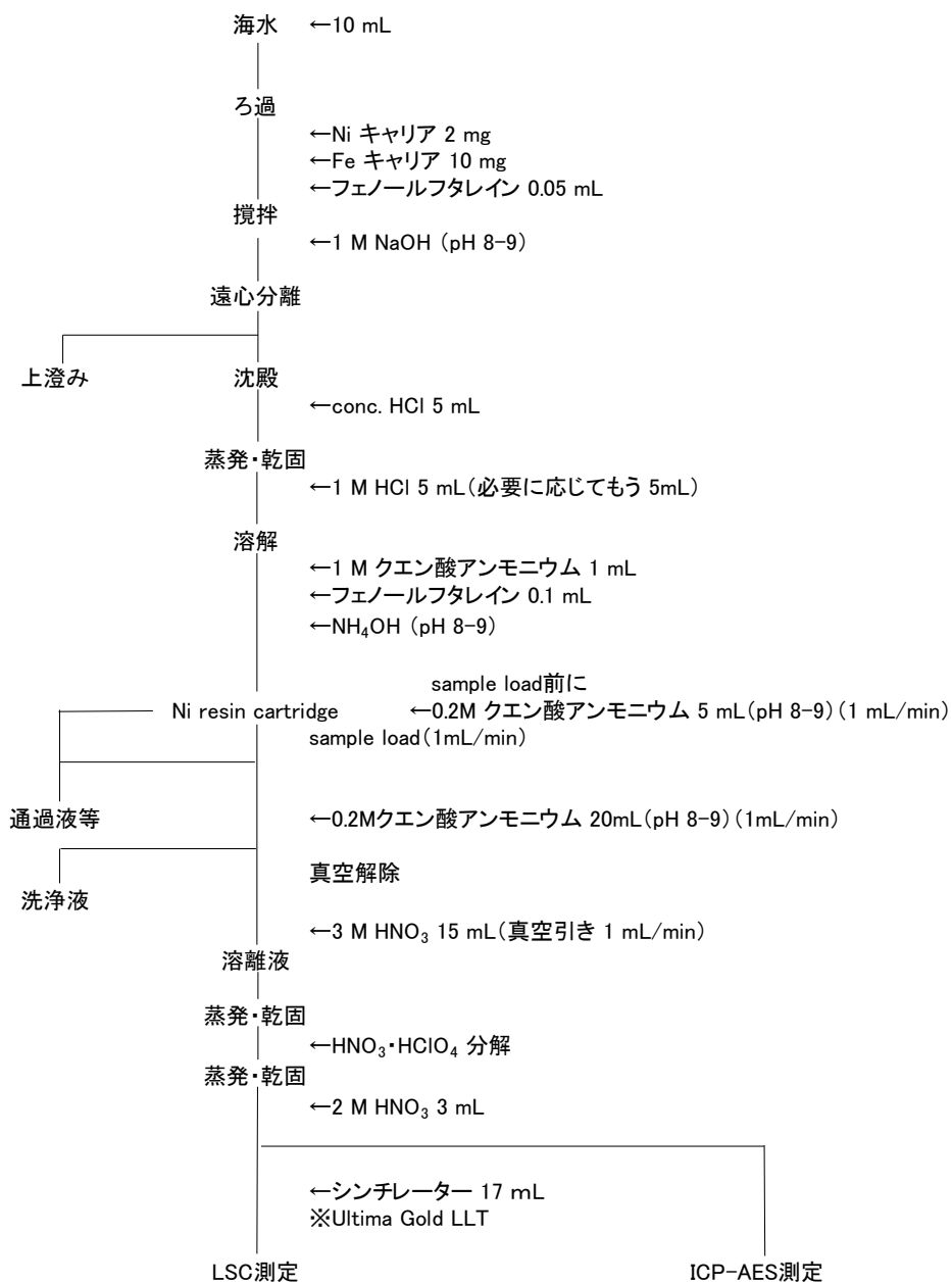
図 4-8 海水のニッケル 63 分析フロー
