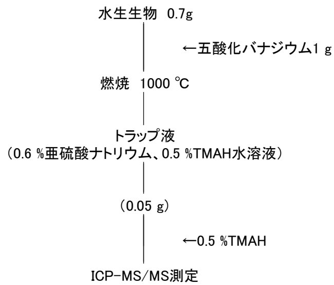
図 4-11 水生生物(海藻類)のヨウ素 129 分析フロー
