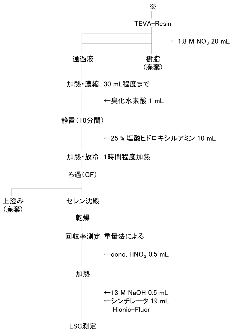
図 4-10 海水のセレン 79 分析フロー(続き)
