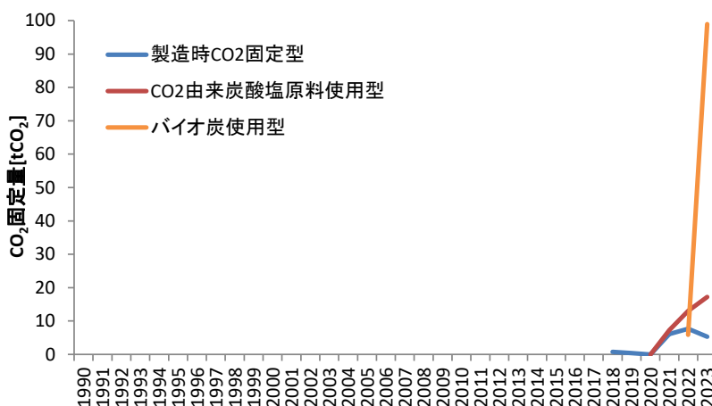
図 1 環境配慮型コンクリートによる CO 2 固定量の推移
