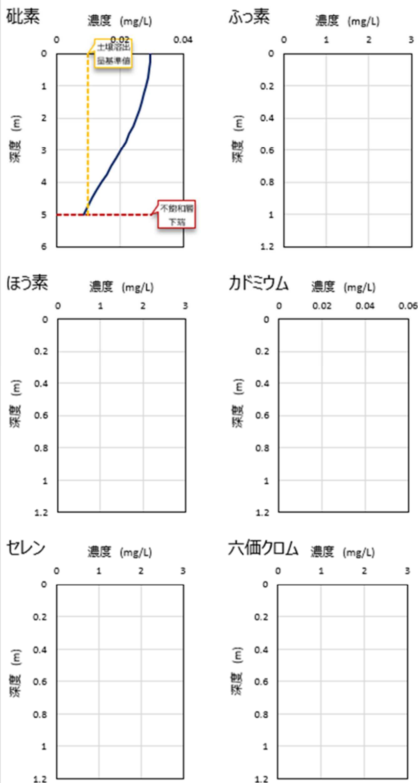
図-20 計算例 4 の場合の不飽和層内の濃度分布
