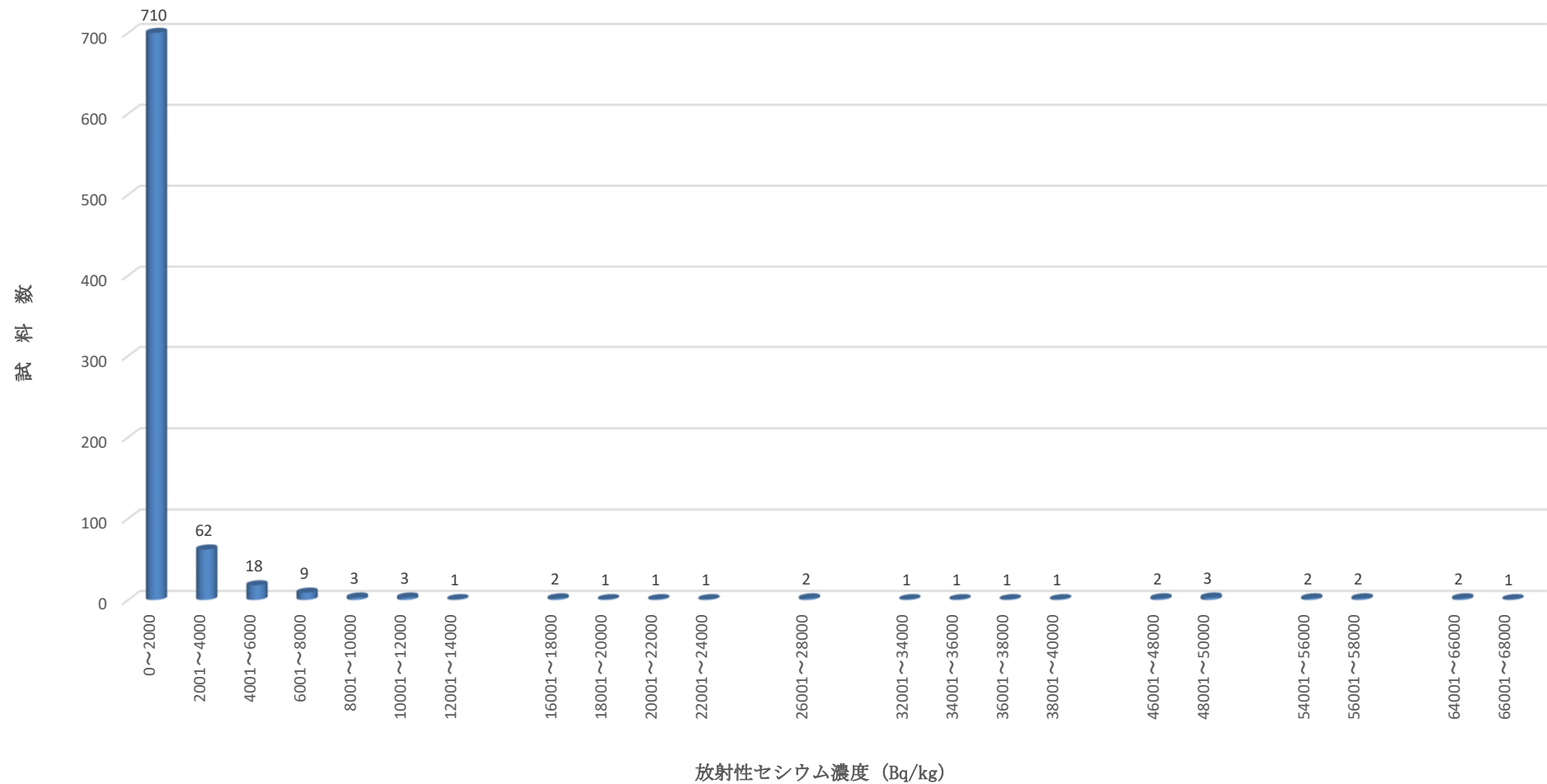
湖沼（底質）の放射性セシウム濃度（2000Bg/kg）ごとの頻度（令和6年度）
