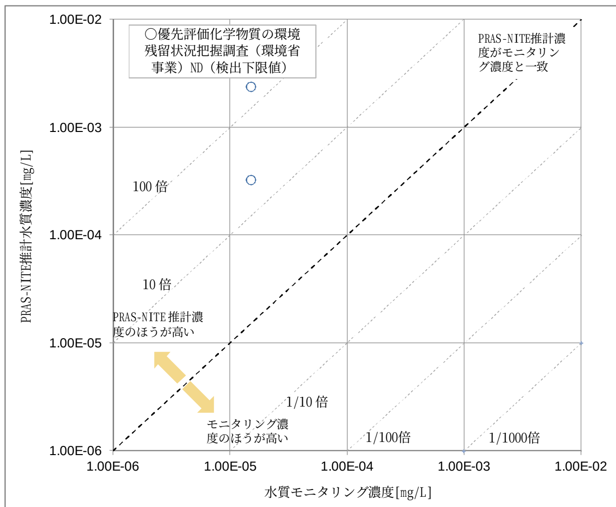
図 5 PRAS-NITE 推計水質濃度 (PRTR、平成 25 年度) と水質モニタリング濃度 (優先評価化学物質の環境残留状況把握調査(環境省請負事業)、平成 27 年度) の比較
