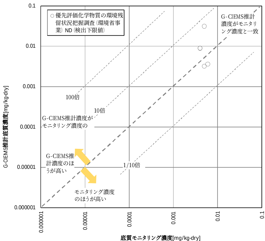
2 3 図 4 G-CIEMS 推計底質濃度 (PRTR、平成 25 年度) と底質モニタリング濃度 (優先評価化学物質の環 4 境残留状況把握調査(環境省請負事業)、平成 27 年度) の比較 5
