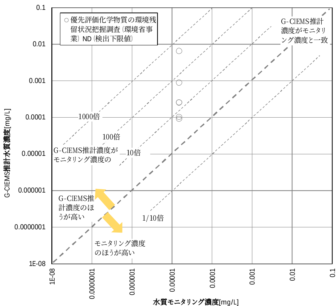
図 3 G-CIEMS 推計水質濃度 (PRTR、平成 25 年度) と水質モニタリング濃度 (優先評価化学物質の環境残留状況把握調査(環境省請負事業)、平成 27 年度) の比較
